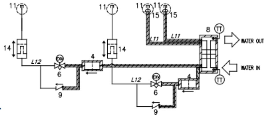
Abbildung 25 – Kältemittel (P&ID) - Kreislaufschem für DUAL-Kreislauf EWYT~CZ-Inneneinheit
