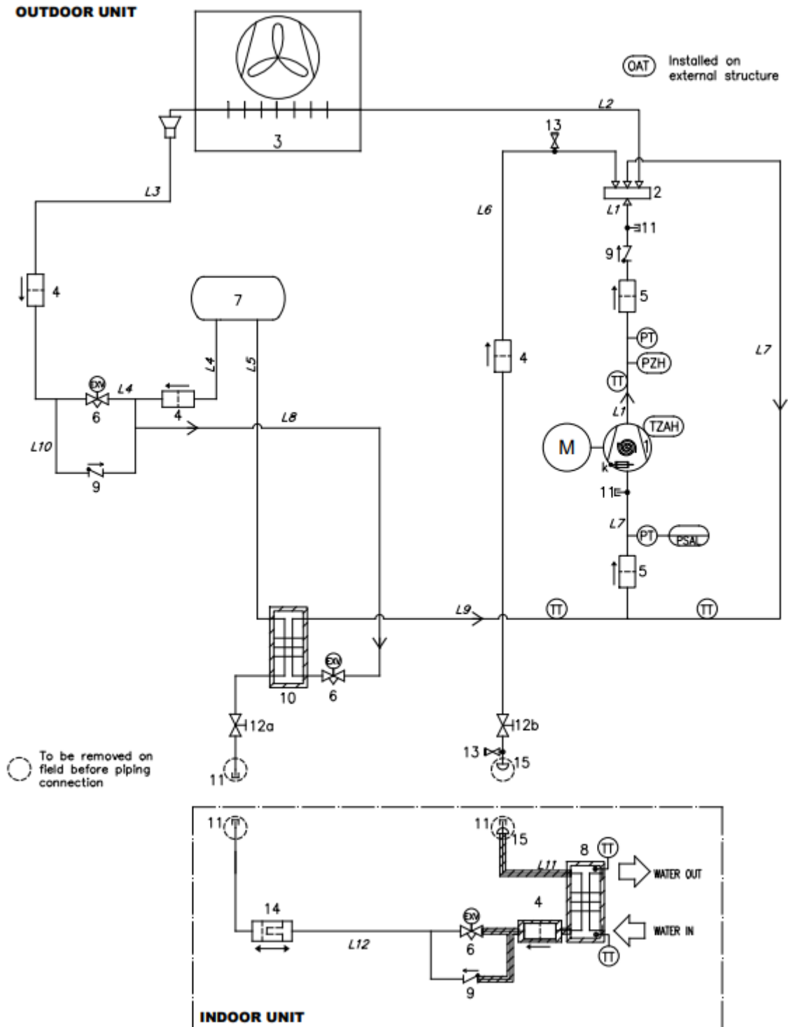
Abbildung 23 – Kältemittel (P&ID)-Kreislaufschemata für MONO-Kreislauf EWYT-CZ-Gerät
