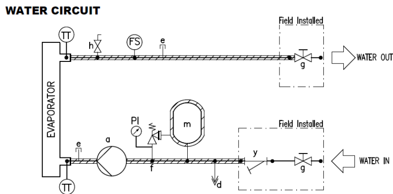
Abbildung 15 – Hydraulisches Schema
