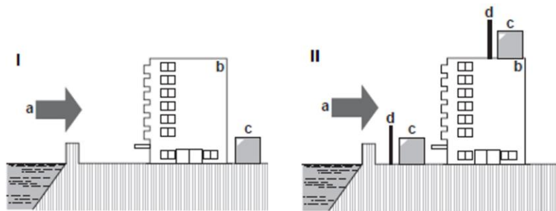
Figura 13 – Instalación junto al mar de la unidad exterior
