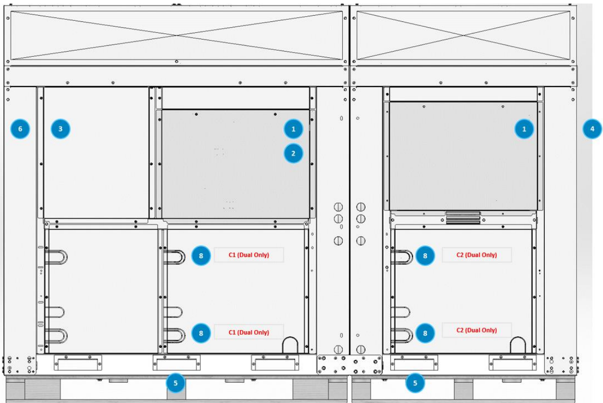
Rysunek 26 – Tabliczki na jednostce zewnętrznej
