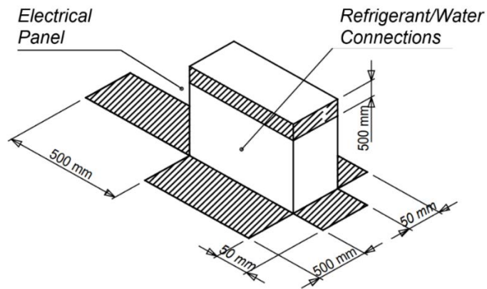
Rysunek 12 – Wymagania dotyczące przestrzeni minimalnej
