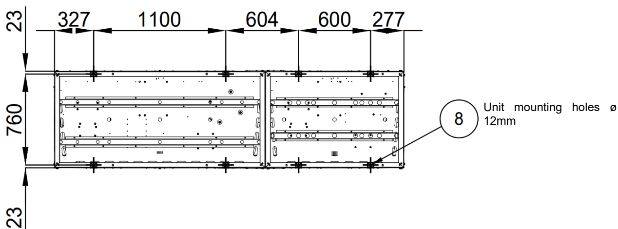
Obrázek 8 – Umístění montážních otvorů (pohled zdola)
