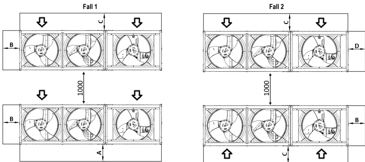
Abbildung 11 – Einheiten, die mit ihren längeren Seiten nebeneinander installiert werden (Fall 1 und Fall 2)
