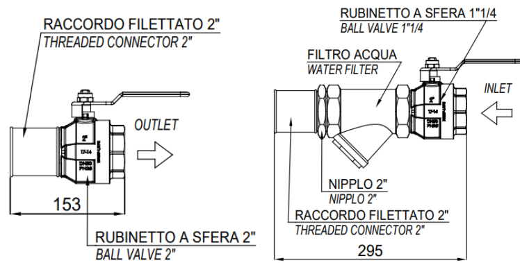
Abbildung 16 – Hydraulische Elemente
