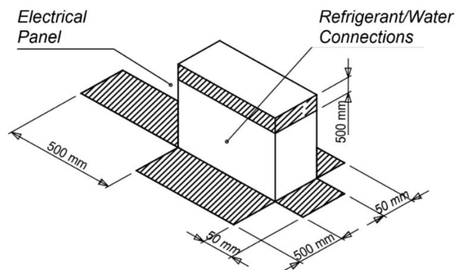
Abbildung 12 – Mindestabstände der Inneneinheit
