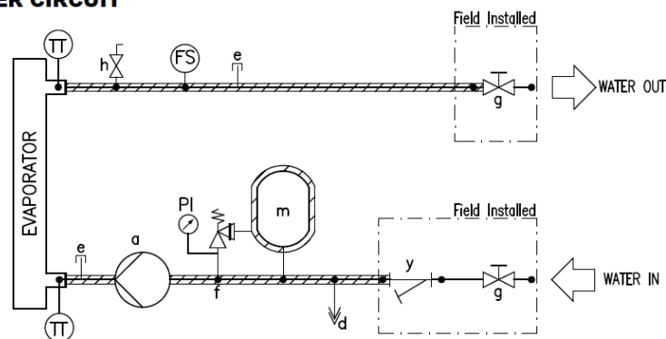
Abbildung 15 – Hydraulisches Schema
