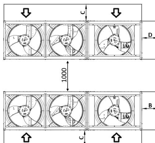
Εικόνα 11 – Μονάδες εγκατεστημένες η μία δίπλα στην άλλη κατά μήκος των μεγαλύτερων πλευρών τους (Περίπτωση 1 και Περίπτωση 2)
