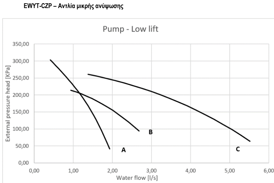
Εικόνα 18 – Εξωτερική κεφαλή πίεσης αντλίας νερού
