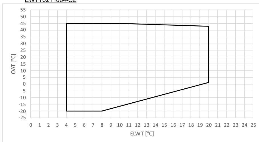
INTERVALO OPERATIVO REFRIGERACIÓN – EWYT_CZ EWYT021~064-CZ
