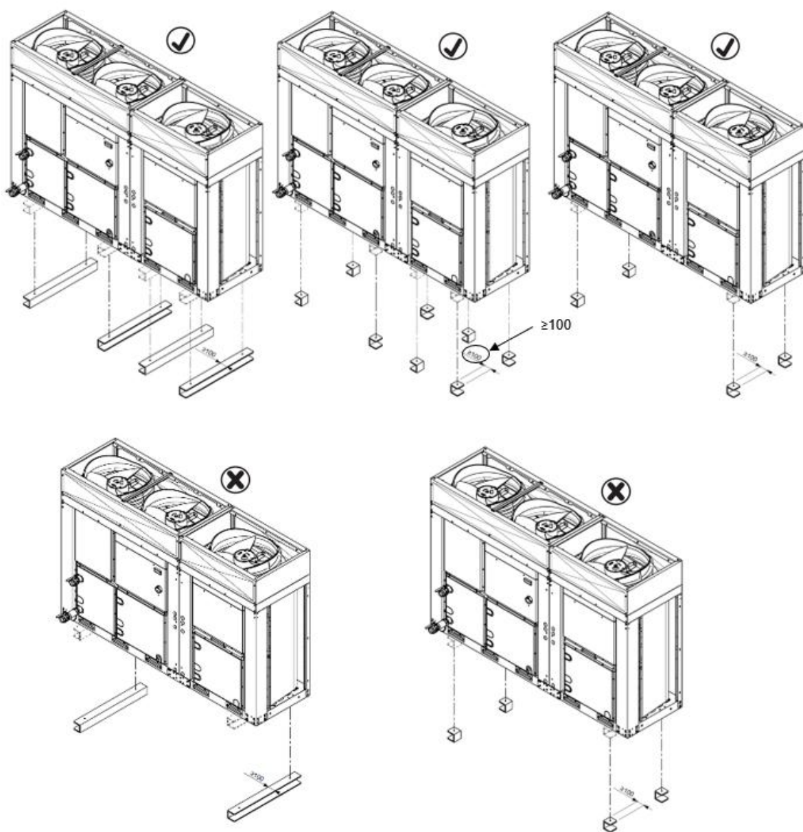
Figura 7 – Posicionamiento de la unidad DOBLE
