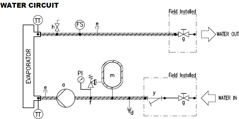
Figura 15 – Schema idraulico
