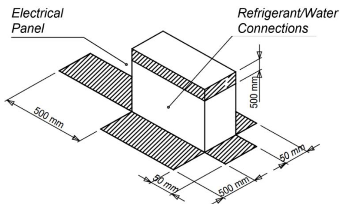
Figura 12 – Requisiti minimi di spazio per l'unità interna
