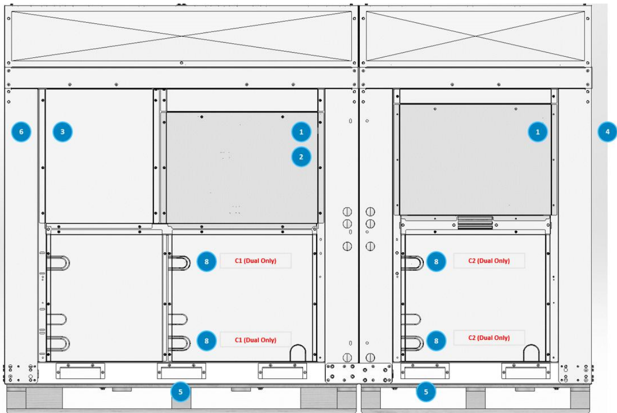
Figura 26 – Etichette sull'unità esterna
