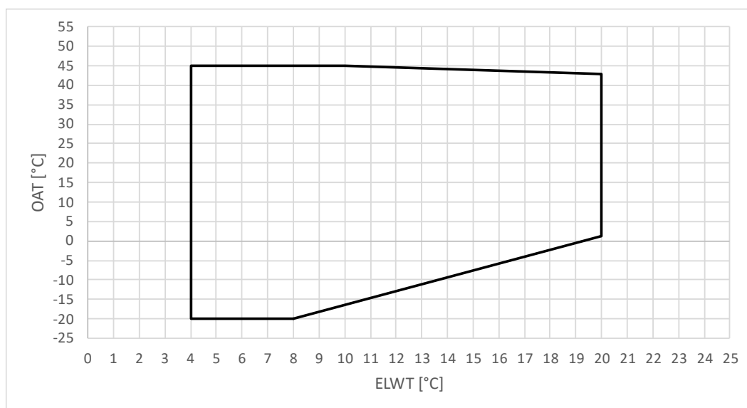
Rysunek 1 – Ograniczenia robocze EWYT_CZ w trybie chłodzenia
