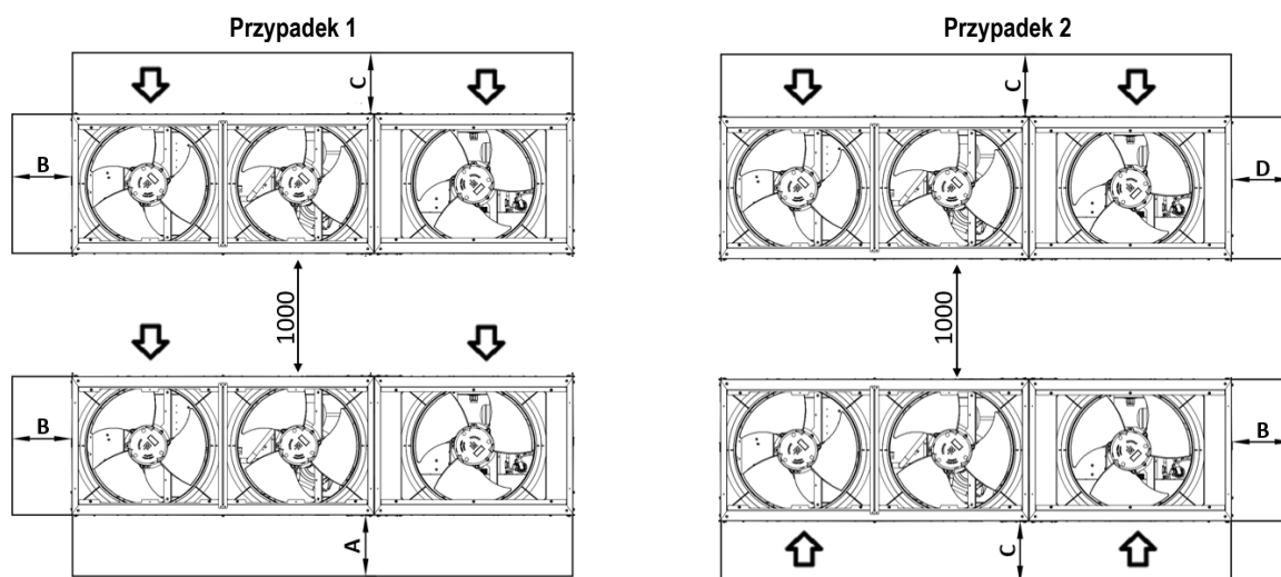
Rysunek 11 – Jednostki instalowane obok siebie wzdłuż dłuższych boków (Przypadek 1 i Przypadek 2)
