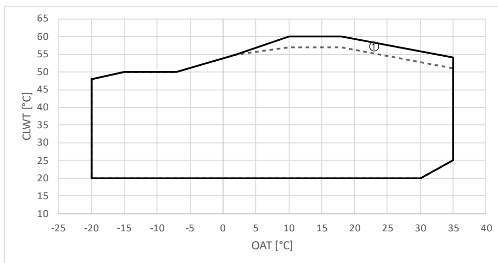
Rysunek 2 – Ograniczenia robocze EWYT_CZ w trybie ogrzewania
