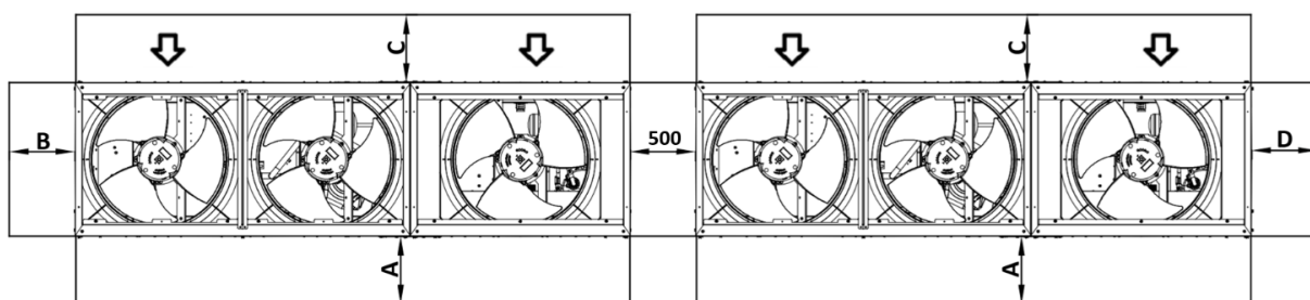
Figura 10 – Unidades instaladas lado-a-lado ao longo dos lados mais curtos, B ou D Caso 1
