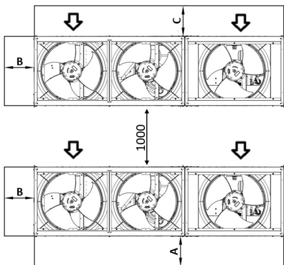
Figura 10 – Unidades instaladas lado-a-lado ao longo dos lados mais curtos, B ou D Caso 1
