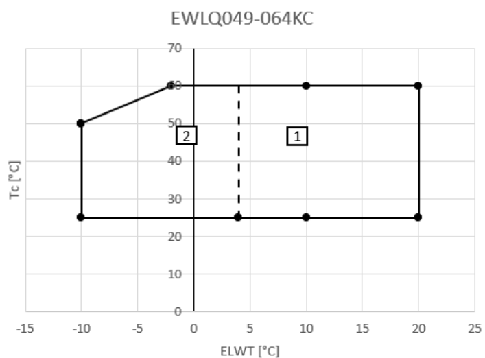
Rysunek 4 - EWLQ049-064KC
