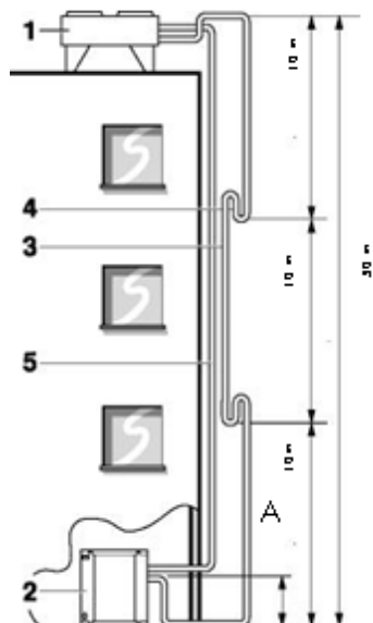
Figura 5-Conexión del circuito de refrigerante (1)
