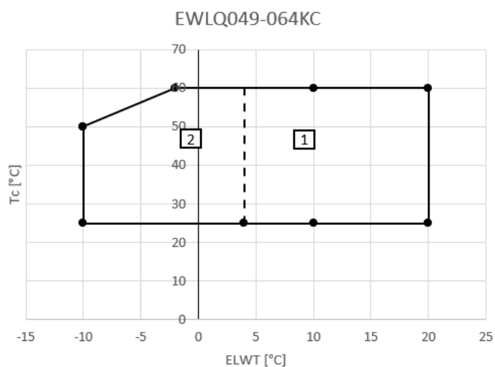
Figura 4 - EWLQ049-064KC
