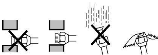
Obrázek 7- Připojení okruhu chladiva (4).
