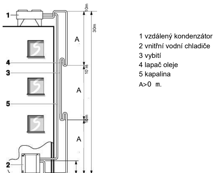
Obrázek 5- Připojení okruhu chladiva (1).
