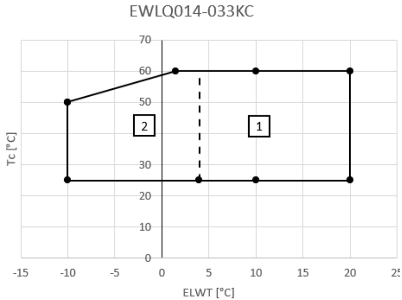
Abbildung 3 - Betriebsbereich EWLQ014-033KC
