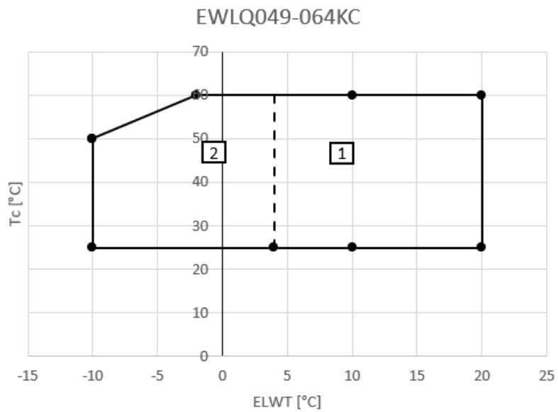
Abbildung 4 - EWLQ049-064KC
