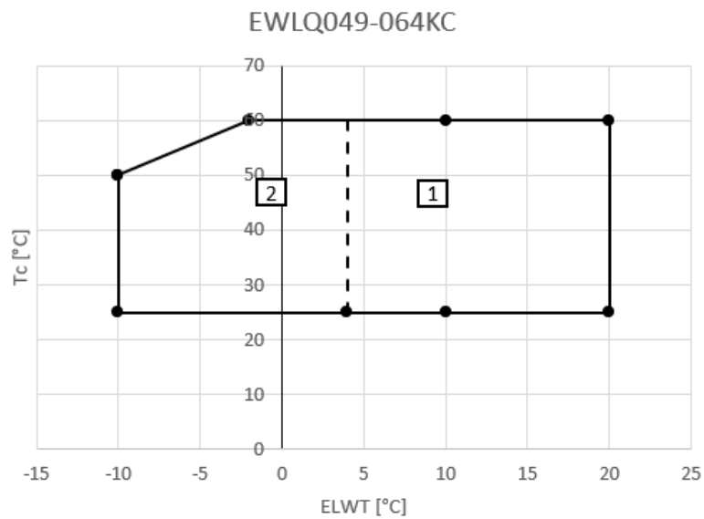
Εικόνα 4 - EWLQ049-064KC
