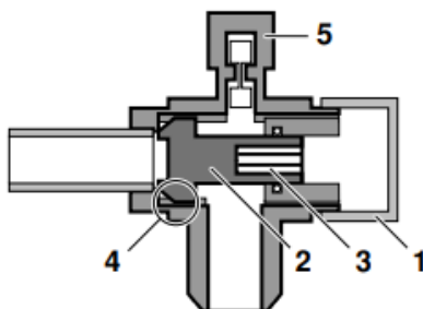
Εικόνα 9 - Πλήρωση της μονάδας
