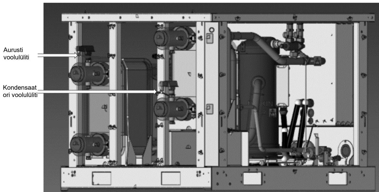
Joonis. 13 – Aurusti voolulüliti kaablite marsruut
