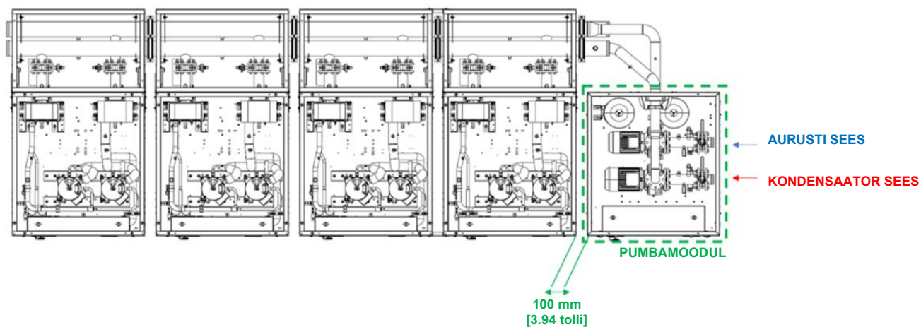
Joonis. 43 – Pumbamooduli paigaldamine – torustiku detailid
