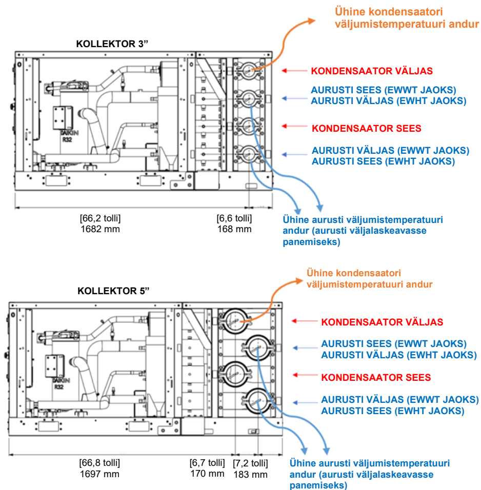
Joonis. 59 – 3" ja 5" kollektori temperatuurisondide asendid
