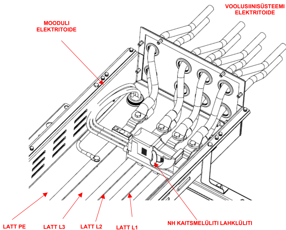
Joonis. 56 – Üksikasjalikud andmed algseadme mooduli elektriühenduse kohta
