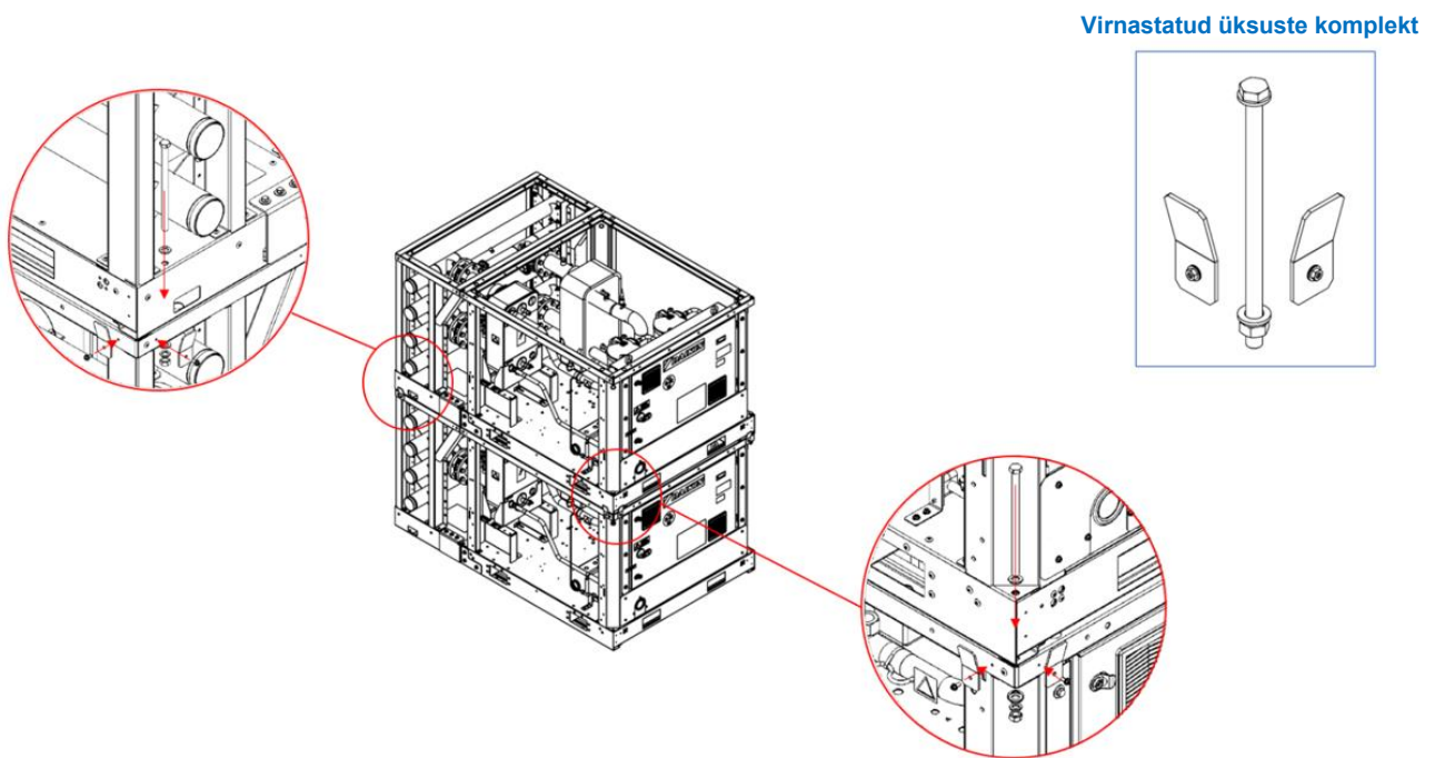
Joonis. 40 – Virnastatud üksuste paigaldusjuhised
