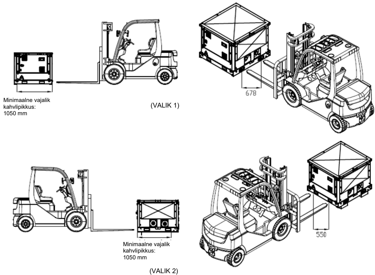
Joonis. 47 – Pumbamooduli käsitlemine kahveltõstukiga
