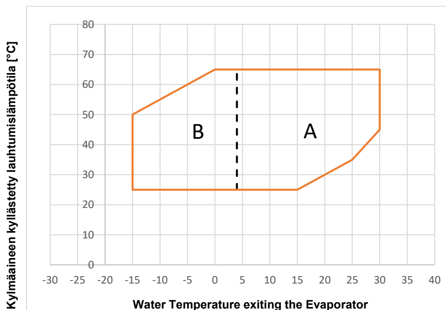
Kuva 7 – EWLT-Q Toimintarajat
