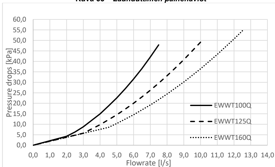
Kuva 63 – Lauhduttimen painehäviöt
