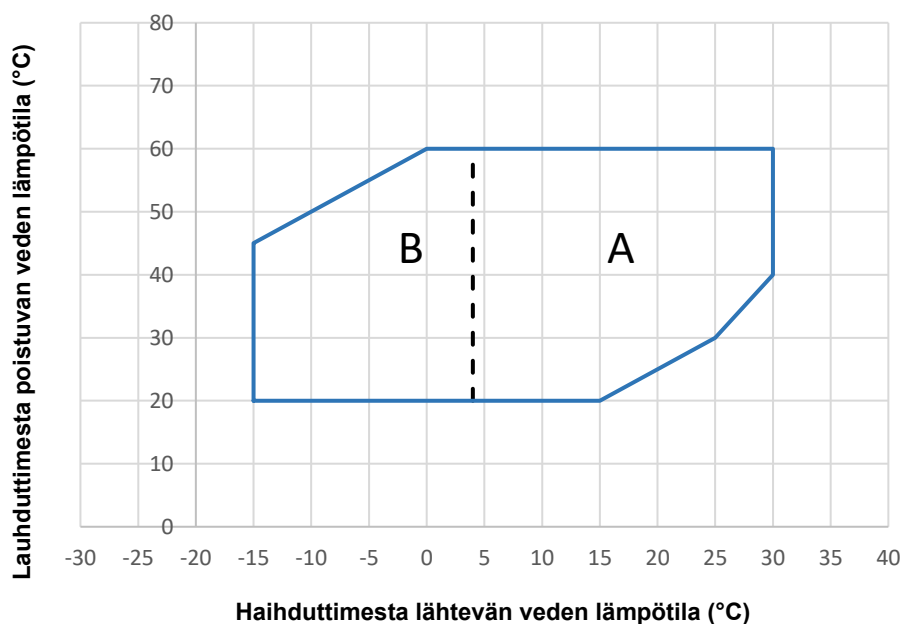
Kuva 7 – EWLT-Q Toimintarajat
