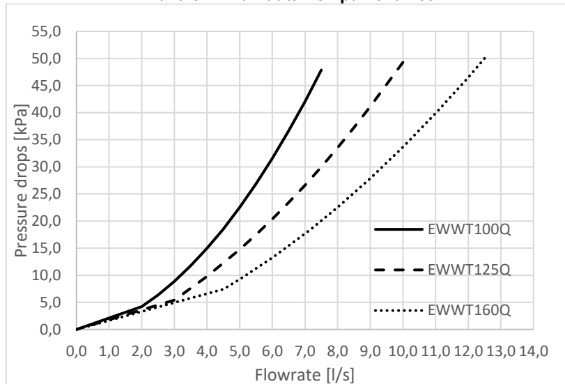
Kuva 63 – Lauhduttimen painehäviöt
