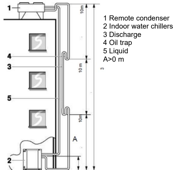
Kuva 17 – Kylmäainepiirin kytkeminen (1)
