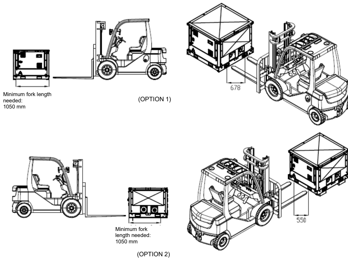
Fig. 47 – Manevrarea modului pompei cu ajutorul motostivuitoarelor
