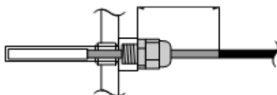
Fig. 16 – Sondă de temperatură a apei \leq 50 mm
