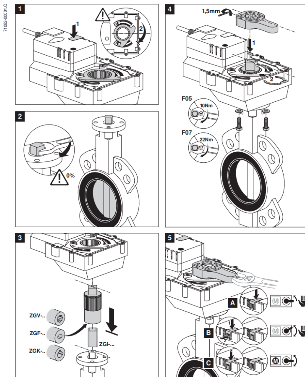
Figur 31– Monteringsinstruktioner för ventilens ställdon
