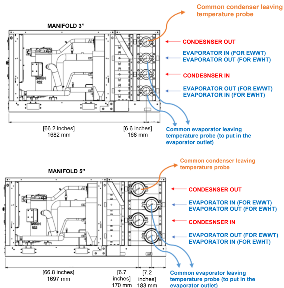
Figur 61– Positioner för temperaturgivare för grenrör 3" och 5"
