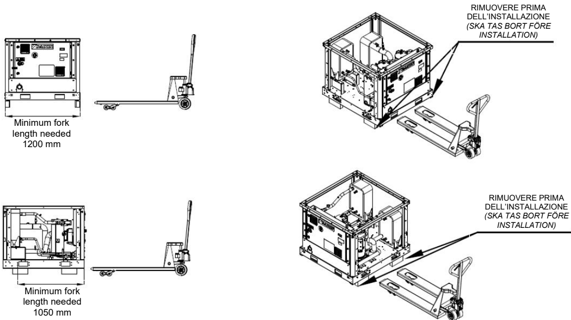
Figur 10– Alternativ hanteringsmetod med pallyftare
