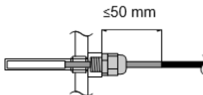
Figur 18– Vattentemperaturgivare
