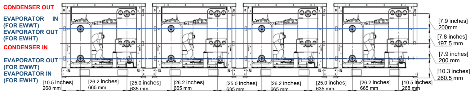
Figur 27– Vattenrörledningens konfiguration
