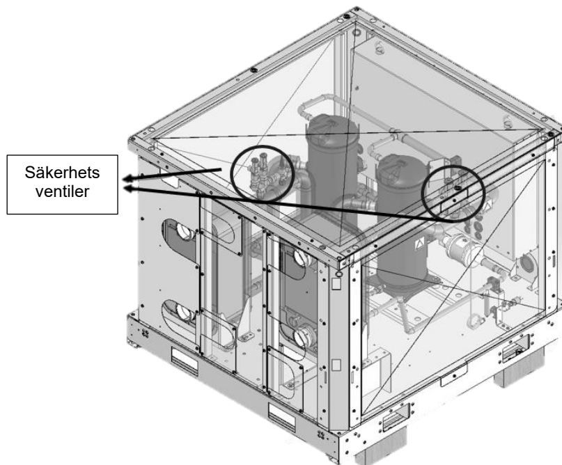
Figur 12– Enhetssäkerhetsventilens position
