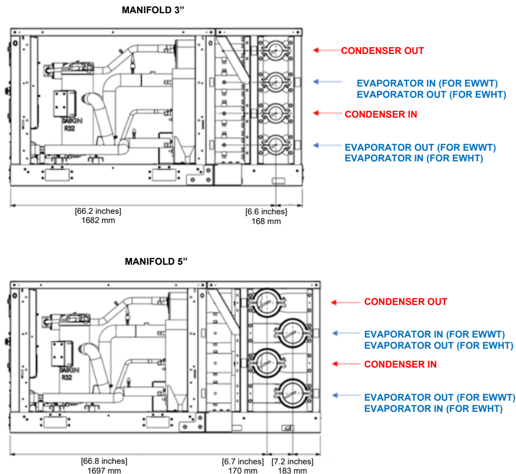
Figur 29– Storlekar för vattengrenrör
