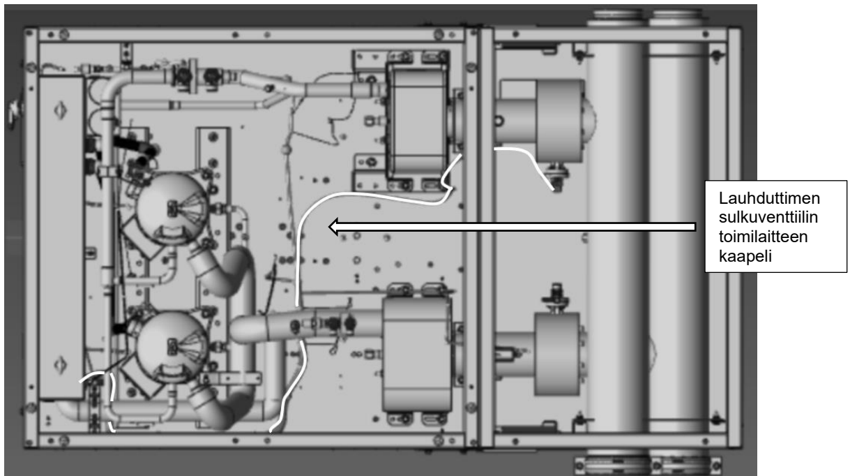
Kuva 37 – Lauhduttimen sulkuventtiilin toimilaitteen kaapelin reititys
