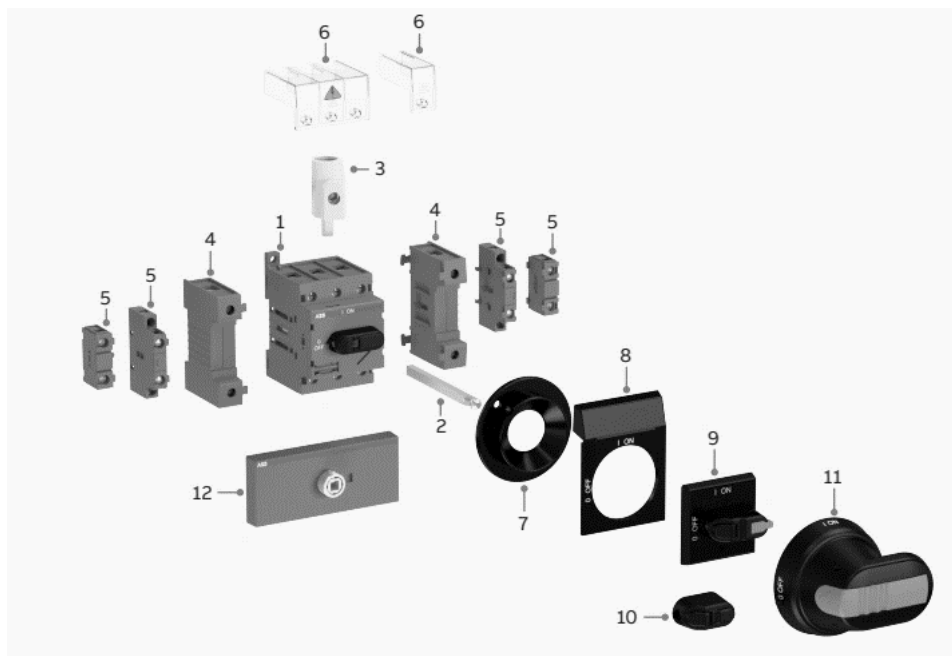
Kuva 20 – Kahvan asennusohjeet
