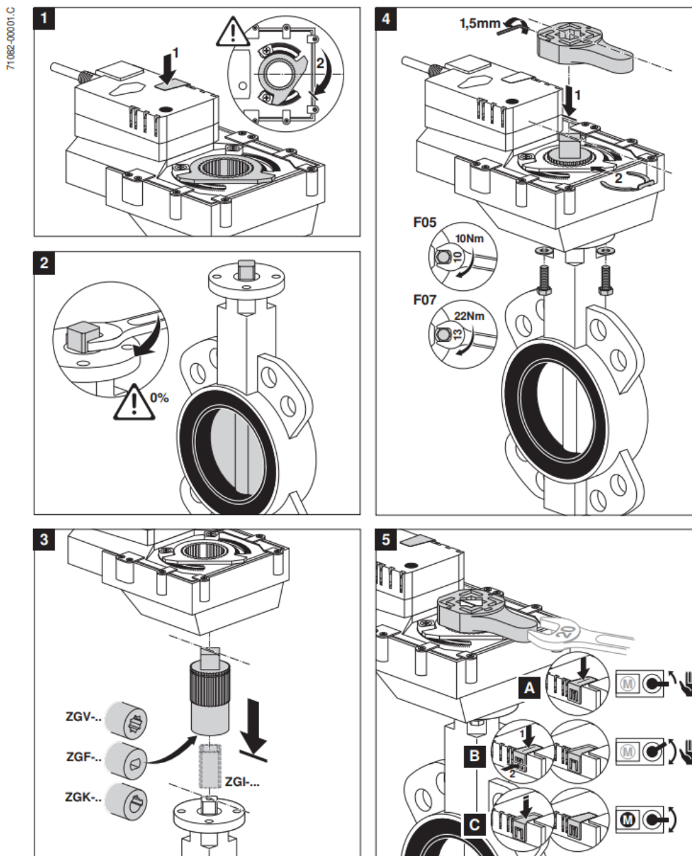
Kuva 30 – Toimilaitteen rajakytkimien asennusohjeet
