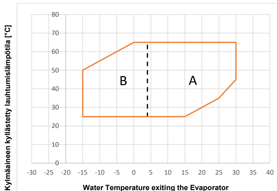
Kuva 7 – EWLT-Q Toimintarajat
