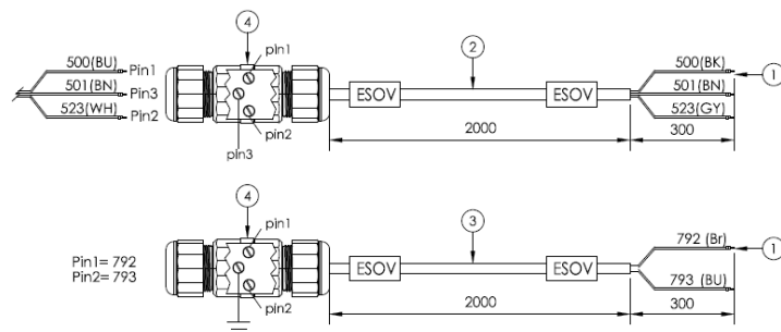
Fig. 33 – Adaptoare de cablu pentru mecanismul de acționare a supapei de închidere a evaporatorului și limitatoare de cursă
