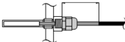
Fig. 16 – Sondă de temperatură a apei ≤50 mm
