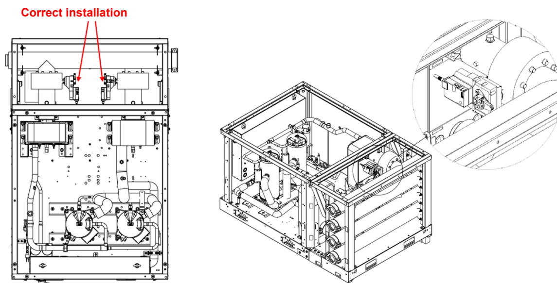
Fig. 31 – Indicații de montare pentru mecanismul de acționare a supapei
