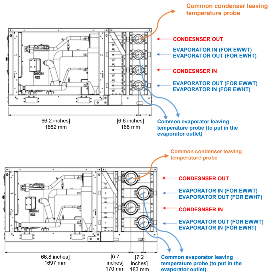
Fig. 59 – Pozițiile sondelor de temperatură pentru colectorul de 3” și 5”
