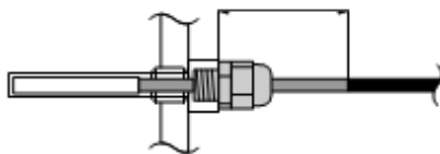
Slika 18 – Sonda za temperaturo vode ≤50 mm
