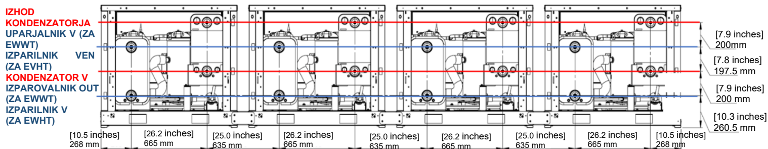
Slika 27 – Konfiguracija vodovodnih cevi
