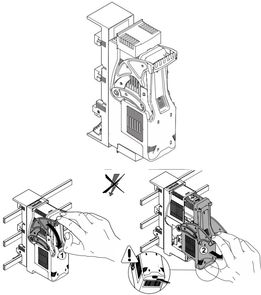
Slika 60 – NH varovalka stikalo odklopnik
