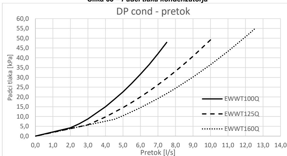
Slika 65 – Padeč tlaka kondenzatorja
