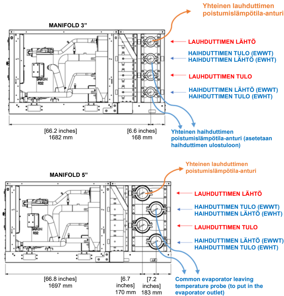
Kuva 62 – 3” ja 5” jakotukkien lämpötila-anturien asennot
