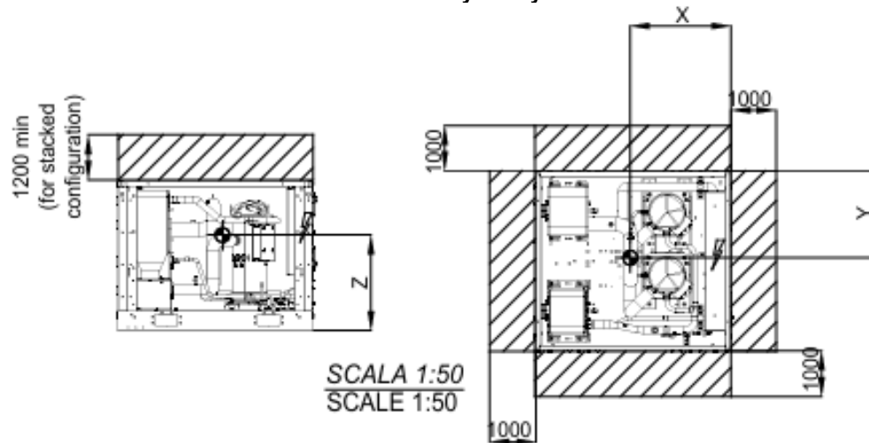
Kuva 8 –Huoltotilan vaatimukset yhden yksikön asennuksessa
