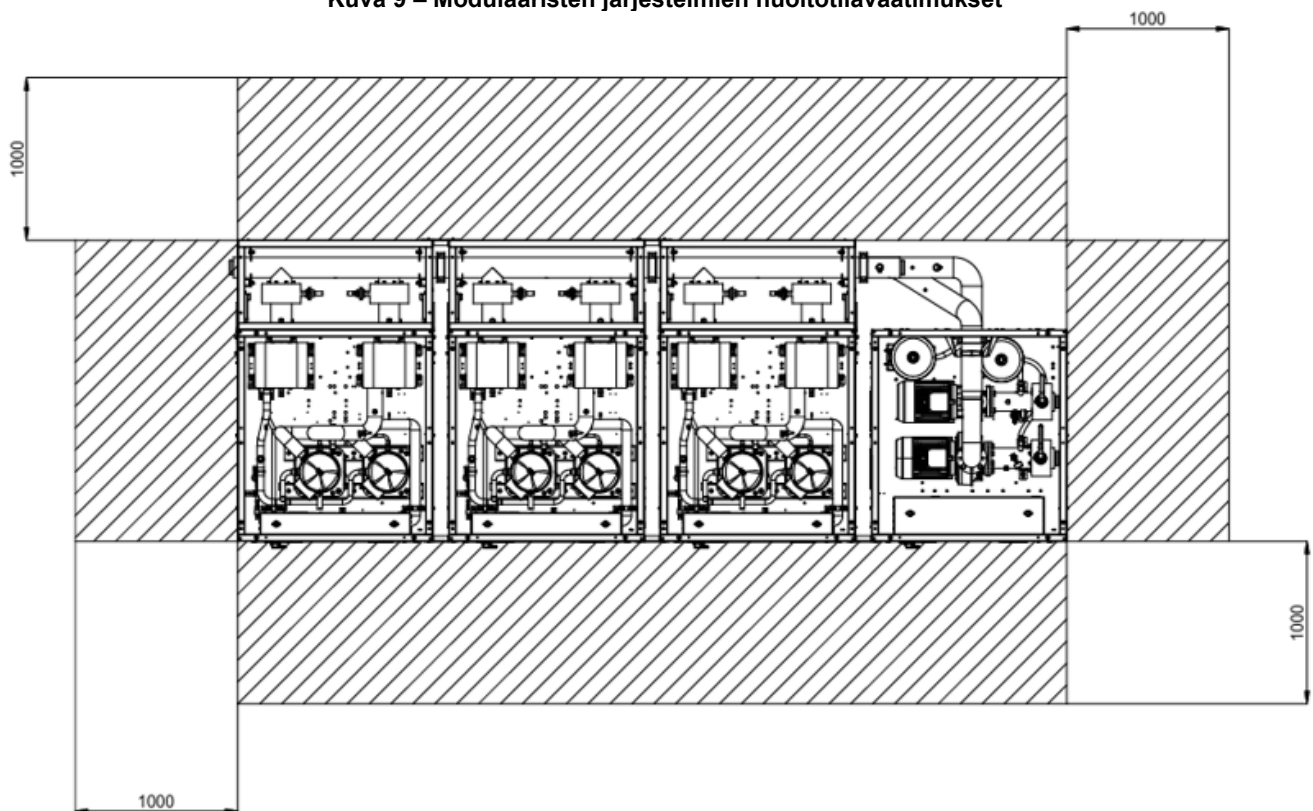
Kuva 9 – Modulaaristen järjestelmien huoltotilavaatimukset
