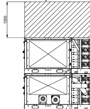
Kuva 10 - Pinottavan kokoonpanon huoltotilan vaatimukset
