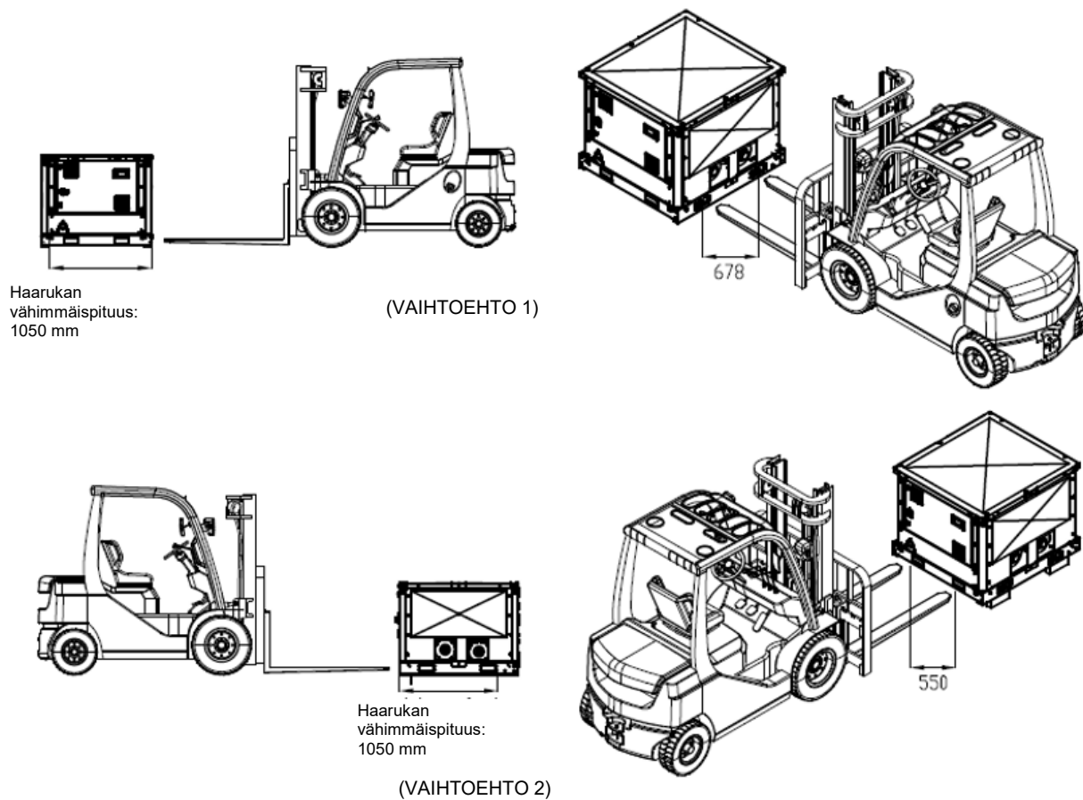
Kuva 50 – Pumppumoduulin käsittely trukilla
