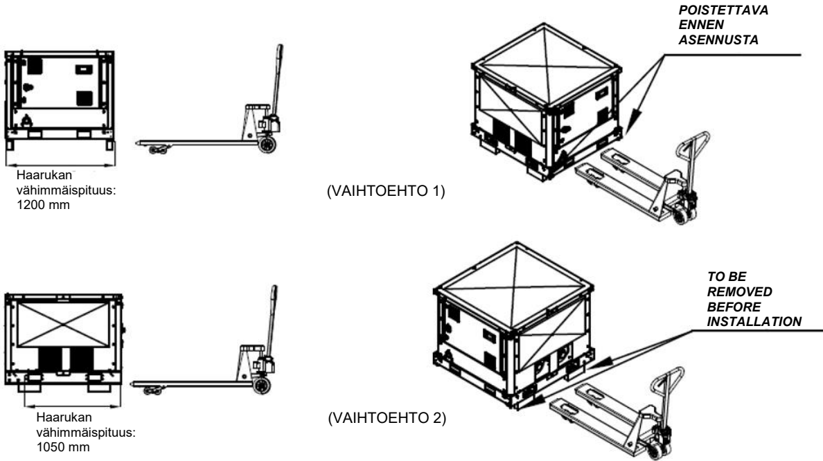
Kuva 51 – Pumpumoduulin käsittely lavansiirtovaunussa
