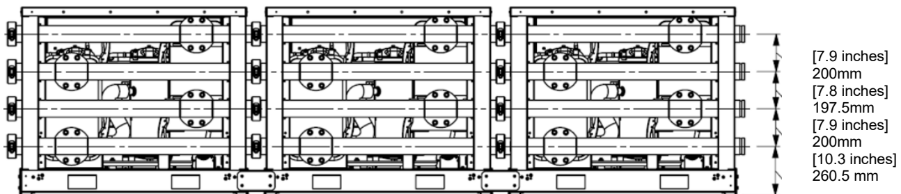
Kuva 31 – Vesiliitäntä moduuleihin
