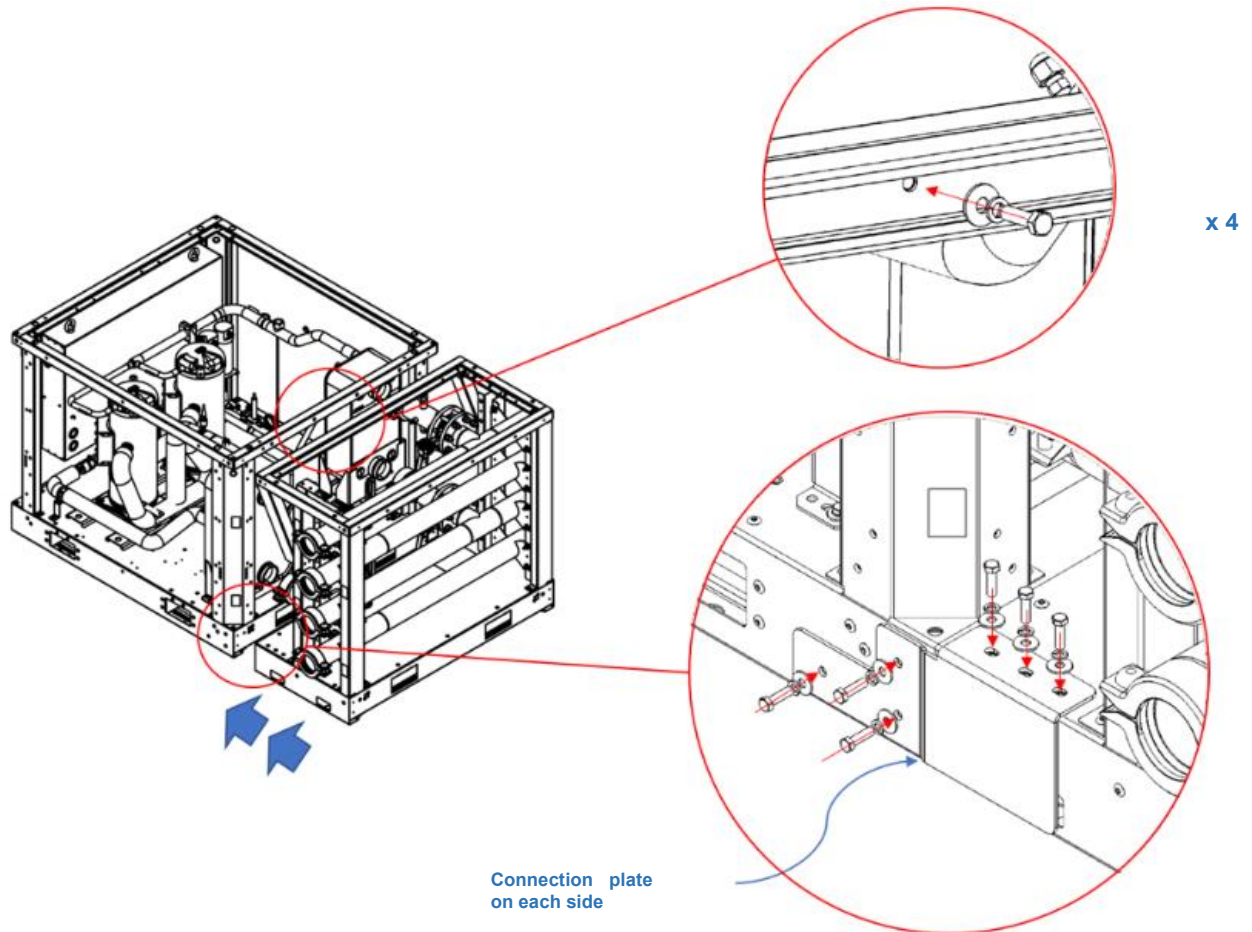
Kuva 26 – Jäähdyttimen ja jakotukin moduulien väliset kytkentäohjeet
