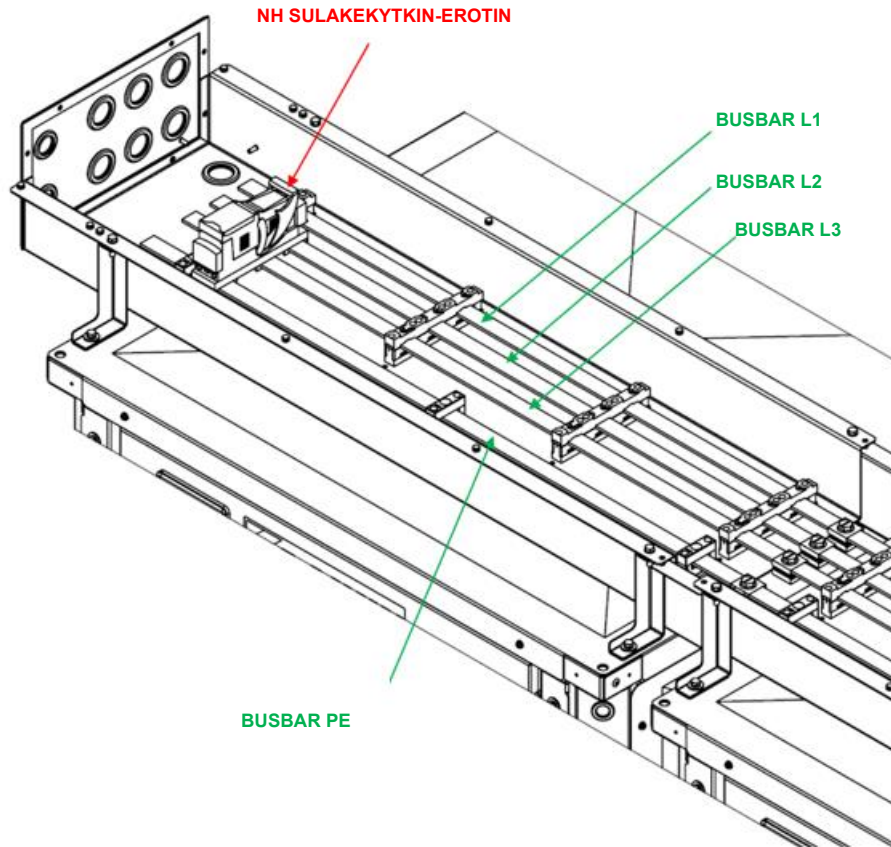
Kuva 58 – Yksityiskohta sulakkeista ja laatikosta tehopalkkimoduulin kaapeleiden reititystä varten
