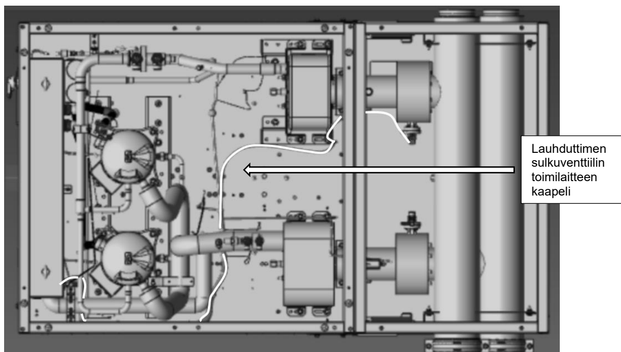
Kuva 40 – Lauhduttimen sulkuventtiilin toimilaitteen kaapelin reititys
