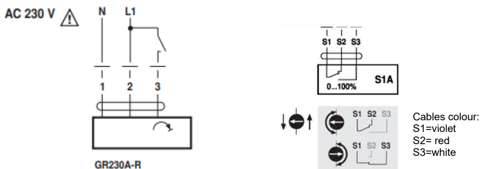
Kuva 35 – Moottorin kytkentäkaavio (vasen kuva) ja rajakytkimet (oikea kuva)
