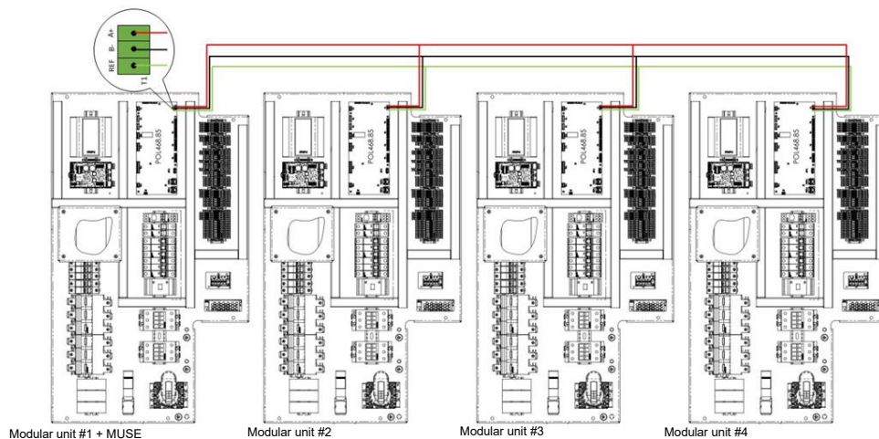
Kuva 64 – 4 PLC:n kytkentä samaan Modbus-verkkoon
