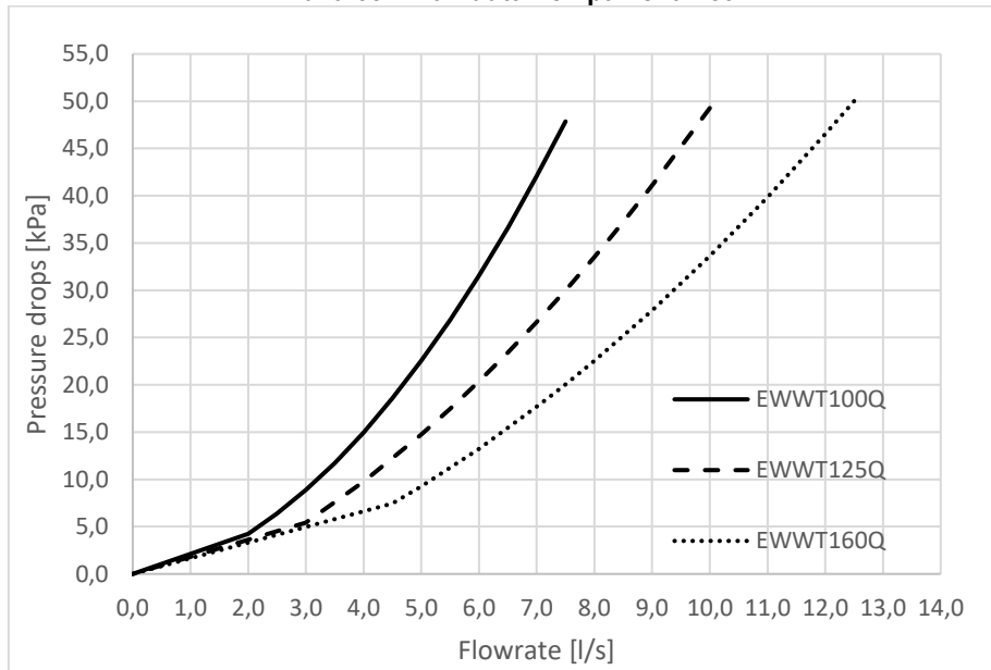
Kuva 66 – Lauhduttimen painehäviöt
