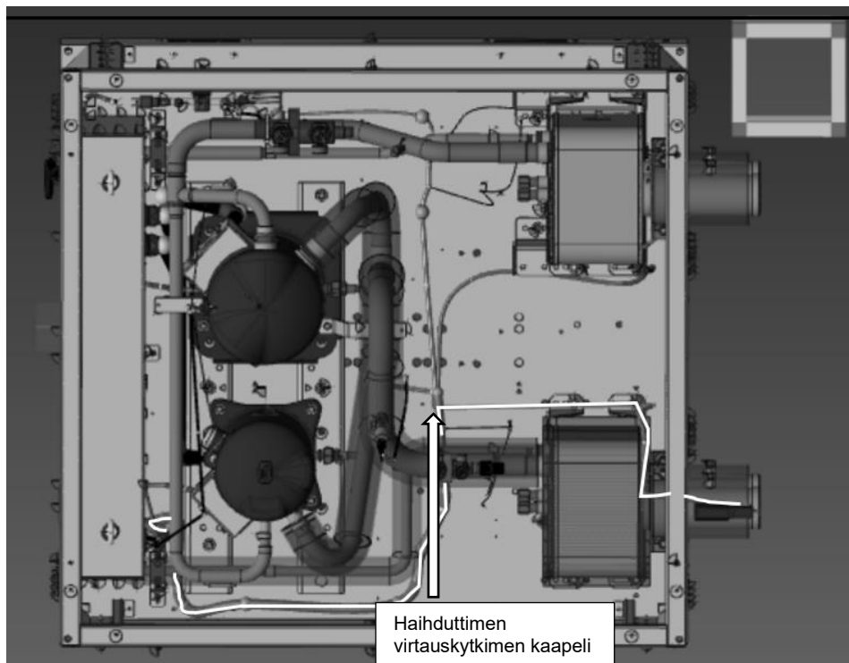
Kuva 16 – Haihduttimen virtauskytkimen kaapelien reititys
