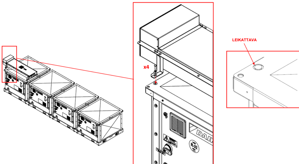
Kuva 55 – Tehopalkkijärjestelmän kiinnitys laitteeseen
