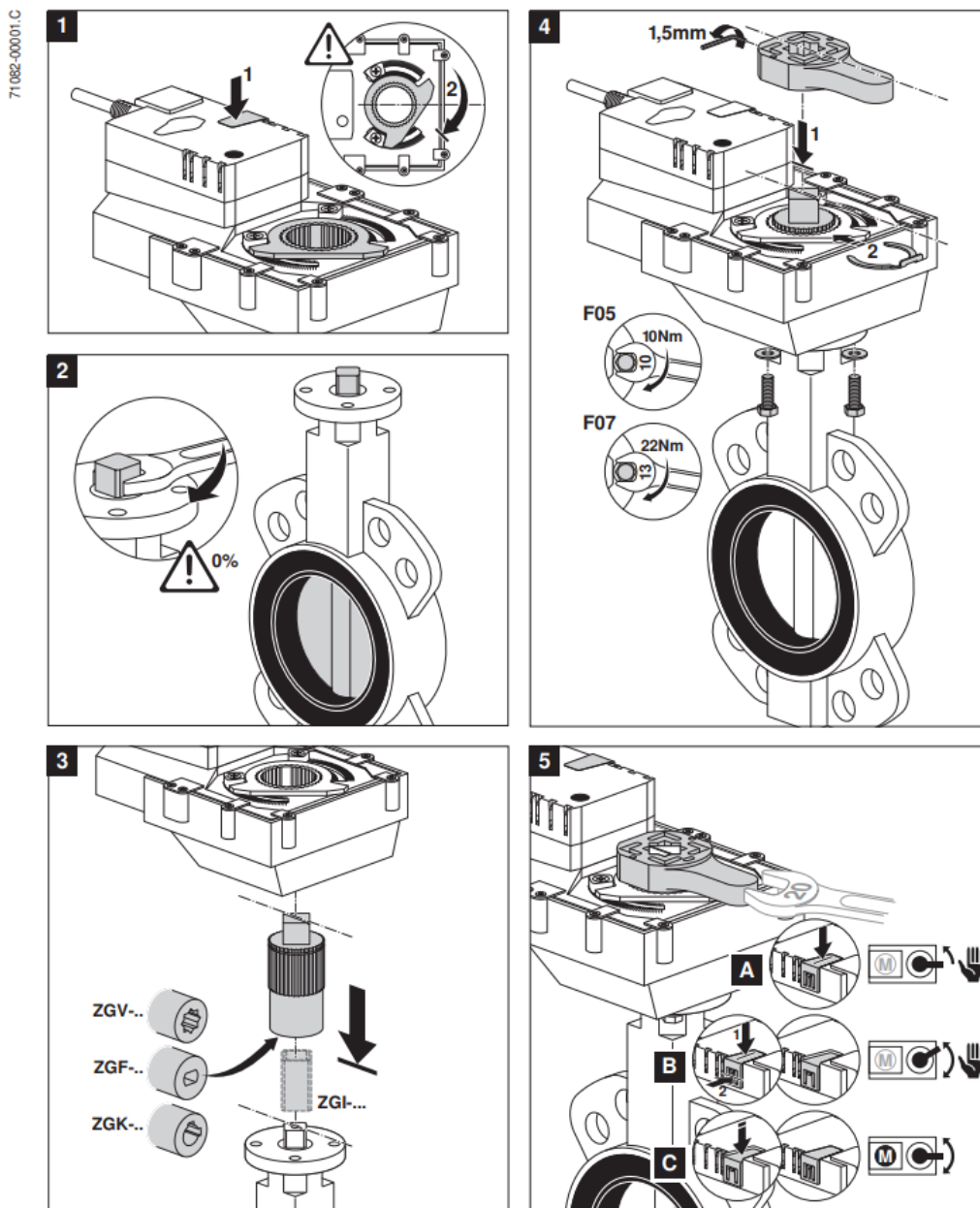
Kuva 32 – Venttiilin toimilaitteen asennusohjeet
