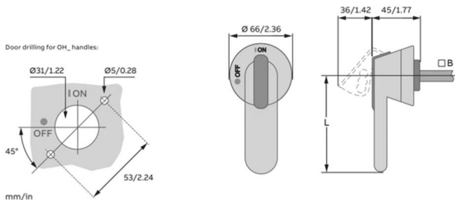
Kuva 24 – Pistoolin kahvan yksityiskohdat
