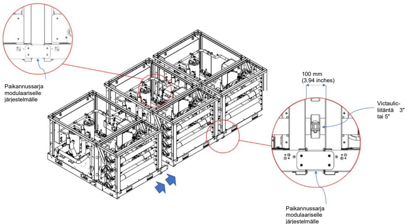
Kuva 29 – Modulaaristen järjestelmien liitäntä
