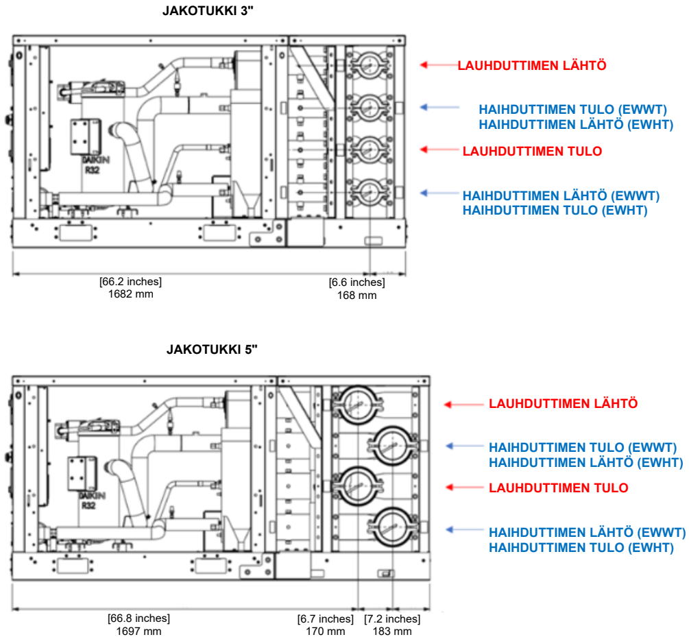
Kuva 30 – Vesiputkistojen koot
