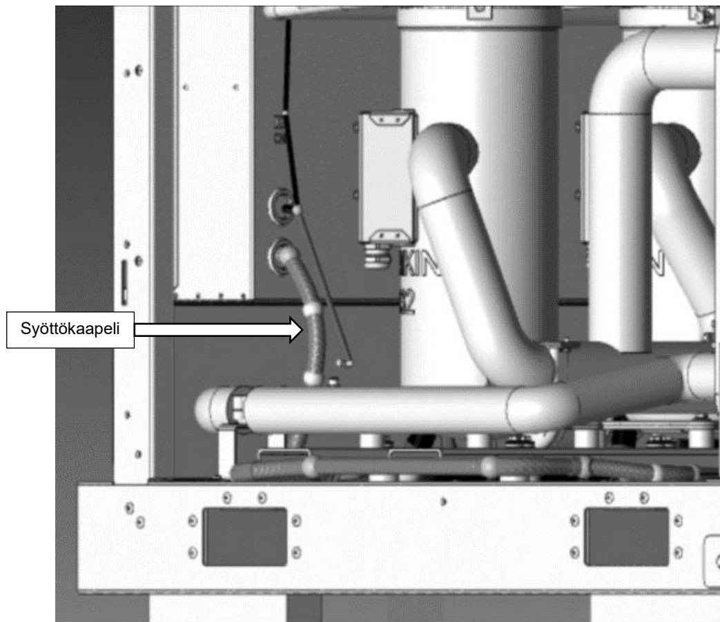
Kuva 41 – Haihduttimen ja lauhduttimen sulkuventtiilin toimilaitekaapeleiden sähkötaulun sisääntulo
