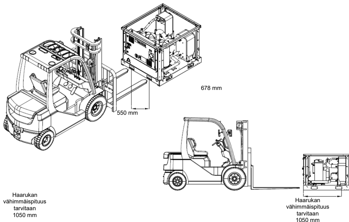
Kuva 12 – Vaihtoehtoinen käsittelytapa trukilla
