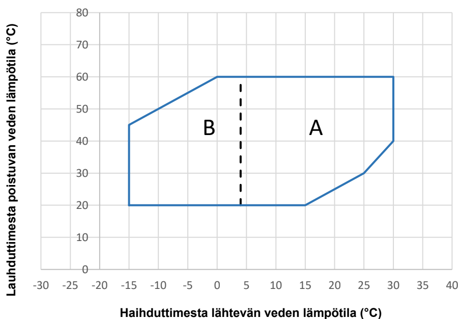
Kuva 7 – EWLT-Q Toimintarajat
