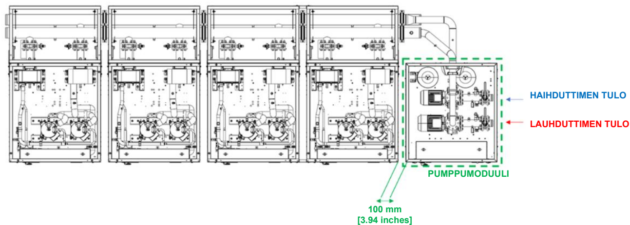
Kuva 45 – Pumppumoduulin asennus
