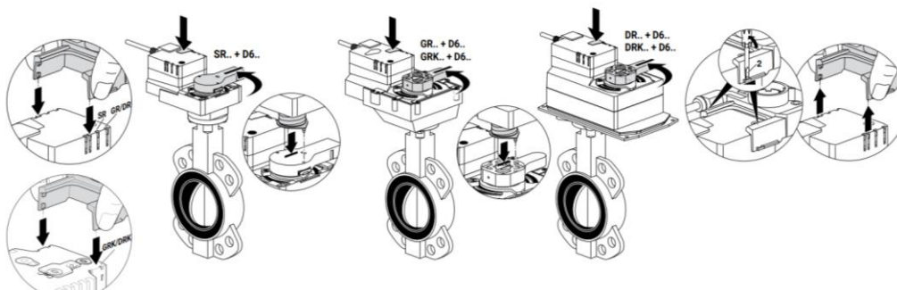
Kuva 33 – Toimilaitteen rajakytkimien asennusohjeet
