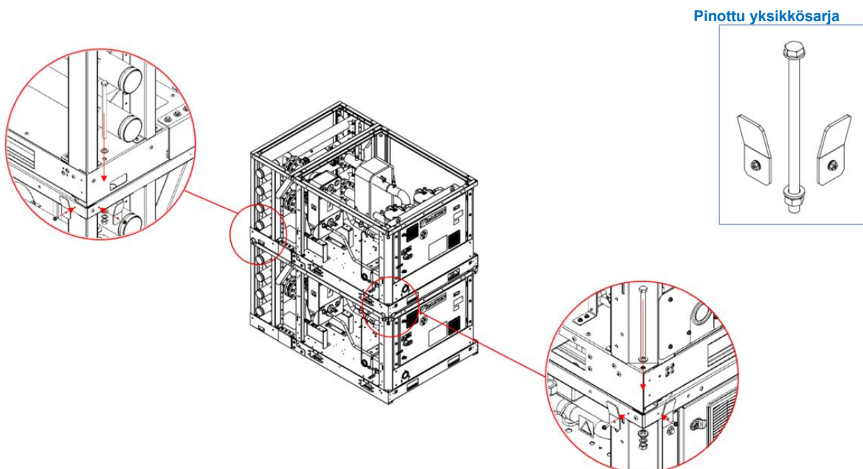
Kuva 43 – Pinottujen yksiköiden asennusohjeet
