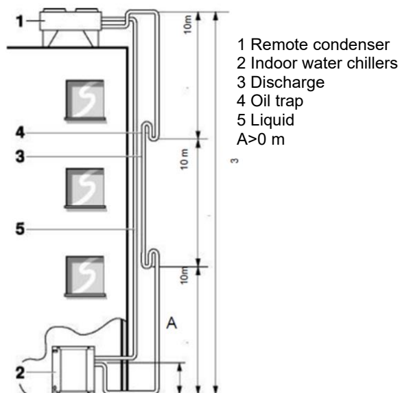
Kuva 20 – Kylmäainepiirin kytkeminen (1)
