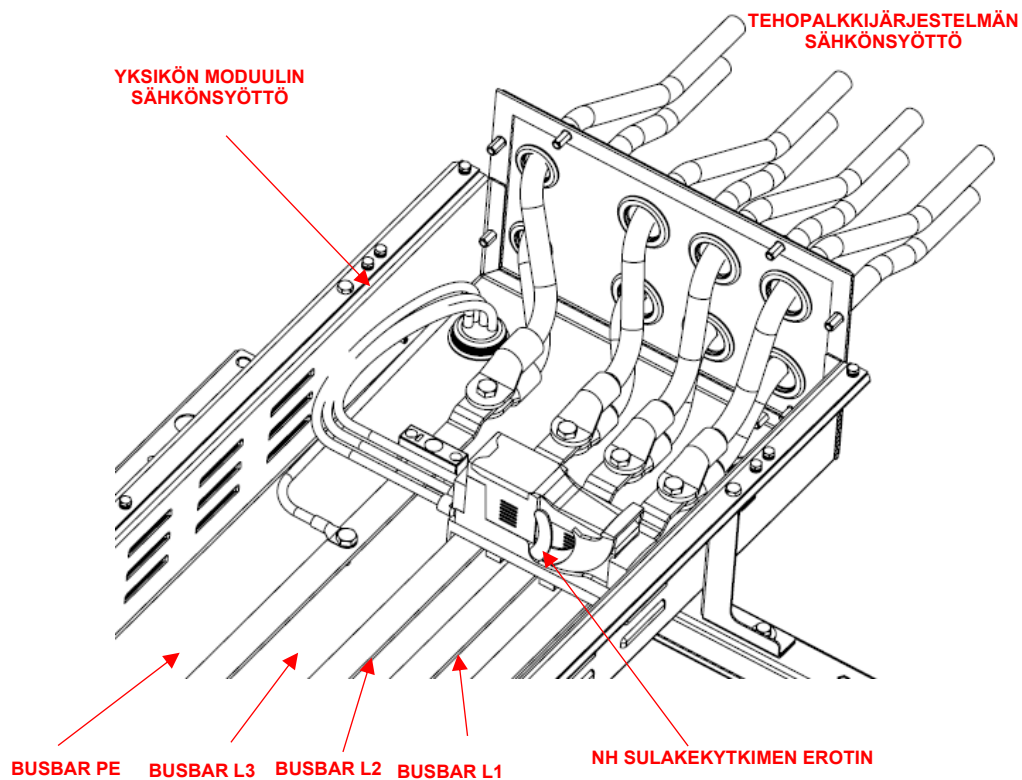
Kuva 59 – Yksityiskohta alkuyksikkömoduulin sähköliitännästä
