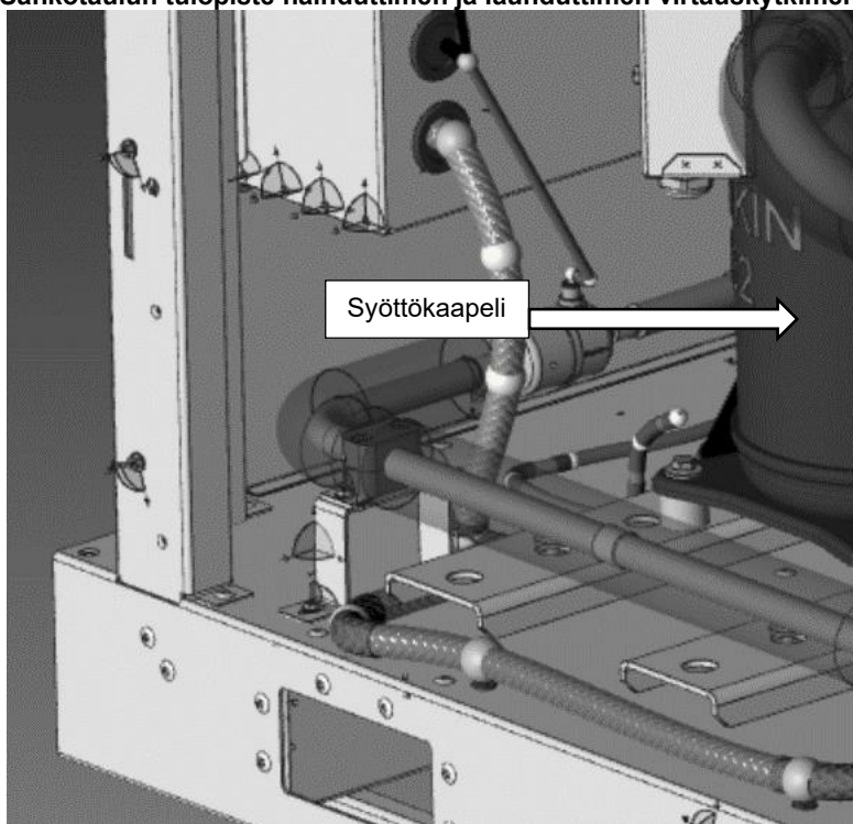
Kuva 18 – Sähkötaulun tulopiste haihduttimen ja lauhduttimen virtauskytkimen kaapeleille
