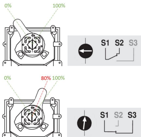
Kuva 42 – Rajakytkimien liipaisimen asetus
