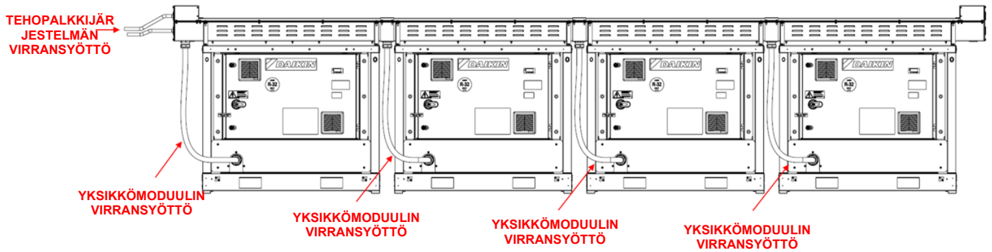
Kuva 54 – Kaapelien reitityksen yksityiskohdat
