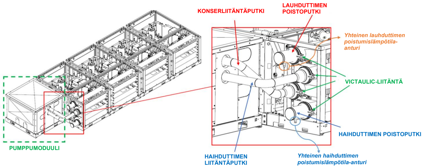
Kuva 63 – Putkissa olevien anturien sijainnin yksityiskohdat
