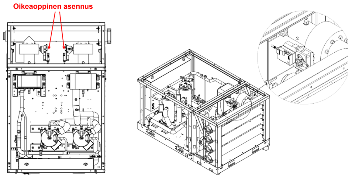
Kuva 34 – Venttiilin toimilaitteen kiinnitysmerkinnät
