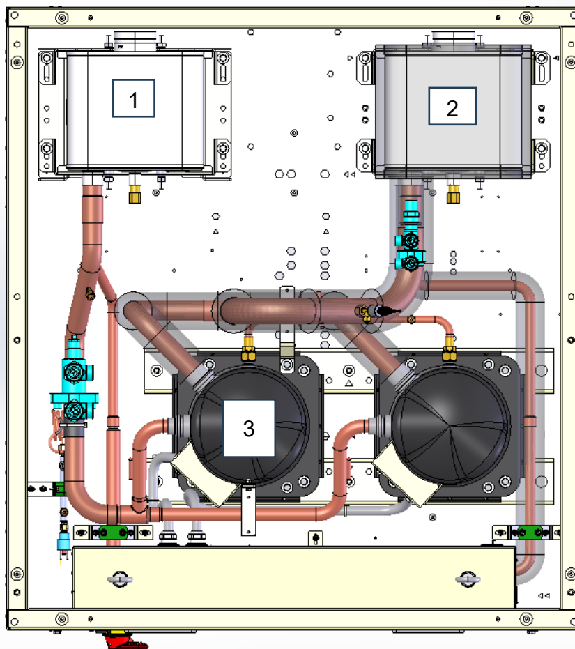
Kuva 14 – Haihduttimen ja lauhduttimen tunnistamisen viitepiirustus
