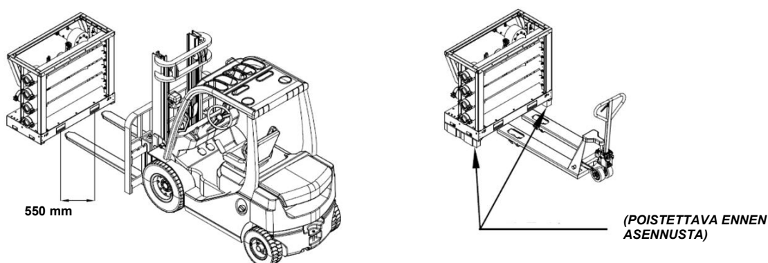
Kuva 47 – Jakotukkimoduulin käsittely
