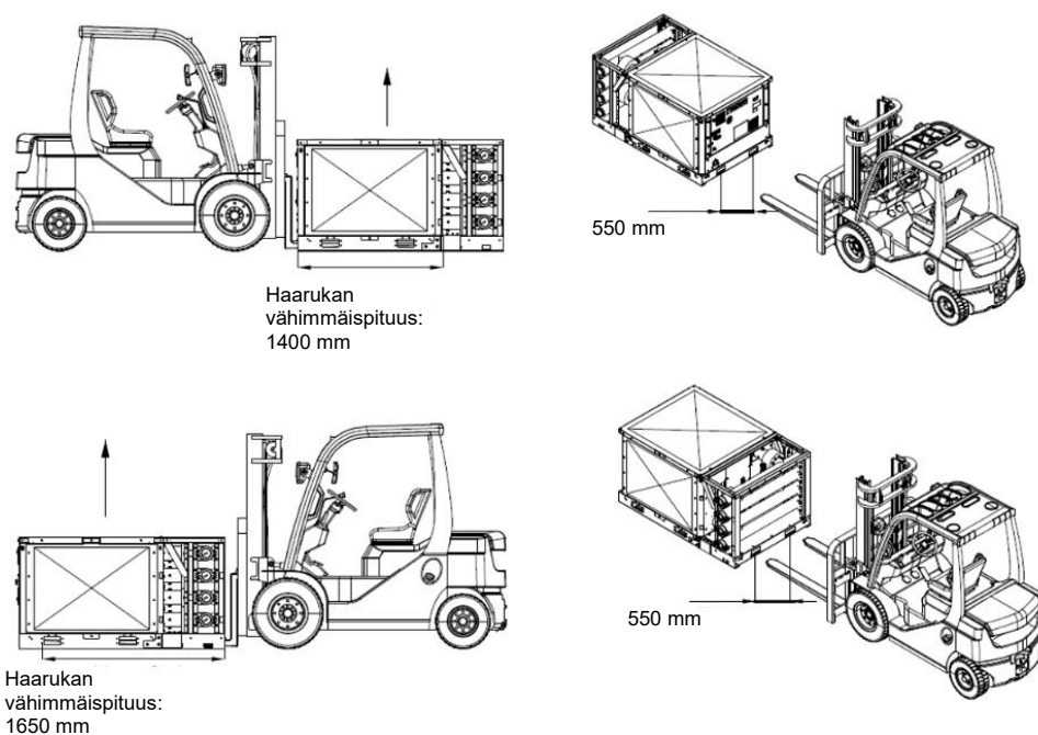
Kuva 48 – Yksikkö- ja jakotukkimoduulien käsittely
