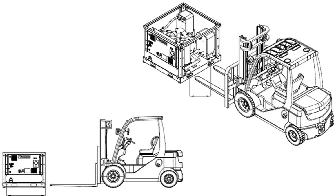
Kuva 11 – Yhden piirin yksikön käsittely
