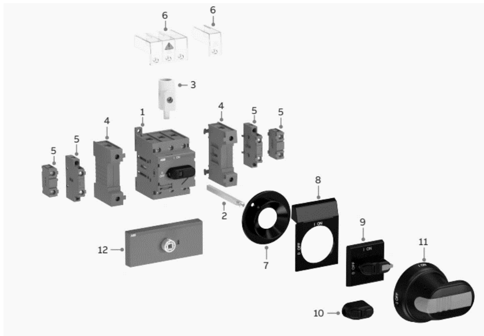
Kuva 23 – Kahvan asennusohjeet
