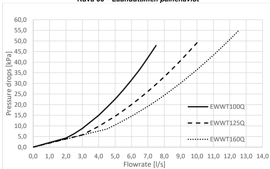
Kuva 66 – Lauhduttimen painehäviöt
