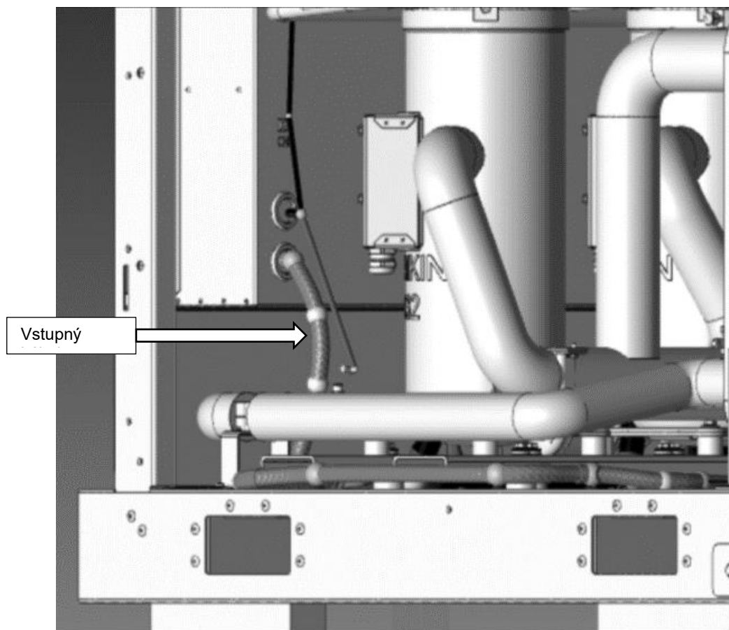
Obr. 41 – Vstup elektrického panelu pre káble ovládača výparníka a ventilu uzatvárania kondenzátora
