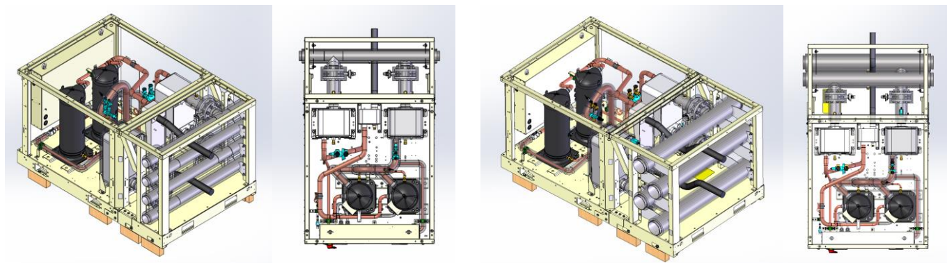
Obr. 27 – potrubia PHR s modulom rozdeľovača (vľavo pre 3-palcové – vpravo pre 5-palcové potrubia rozdeľovača)
