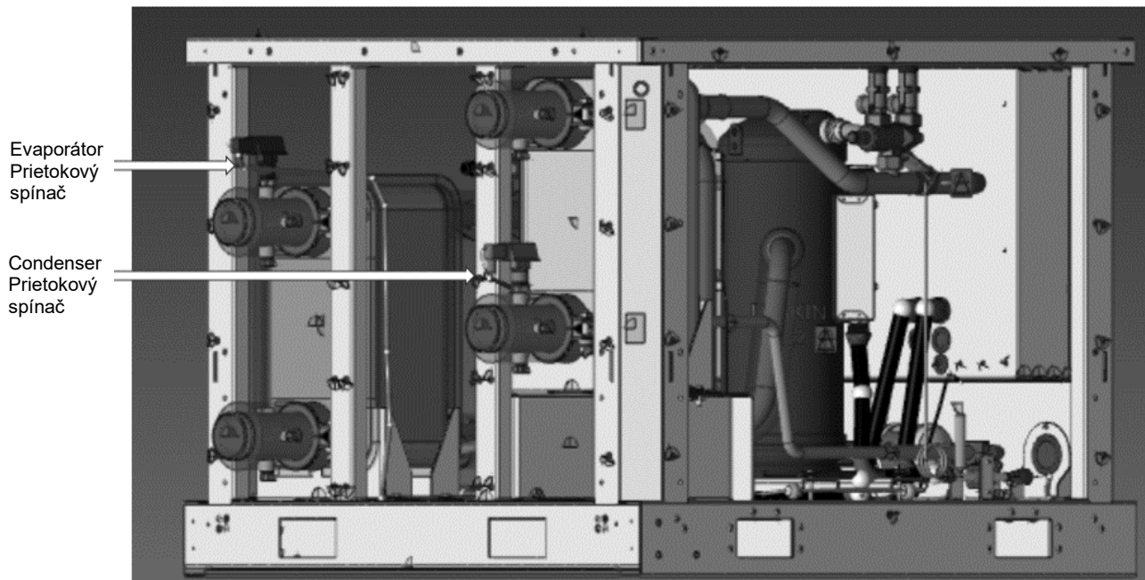
Obr. 16 – Vedenie káblov spínača prietoku výparníka
