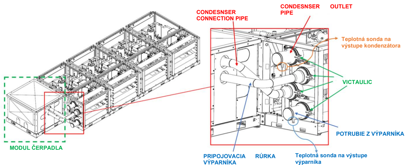
Obr. 63 – Podrobnosti o umiestnení sond na potrubíach
