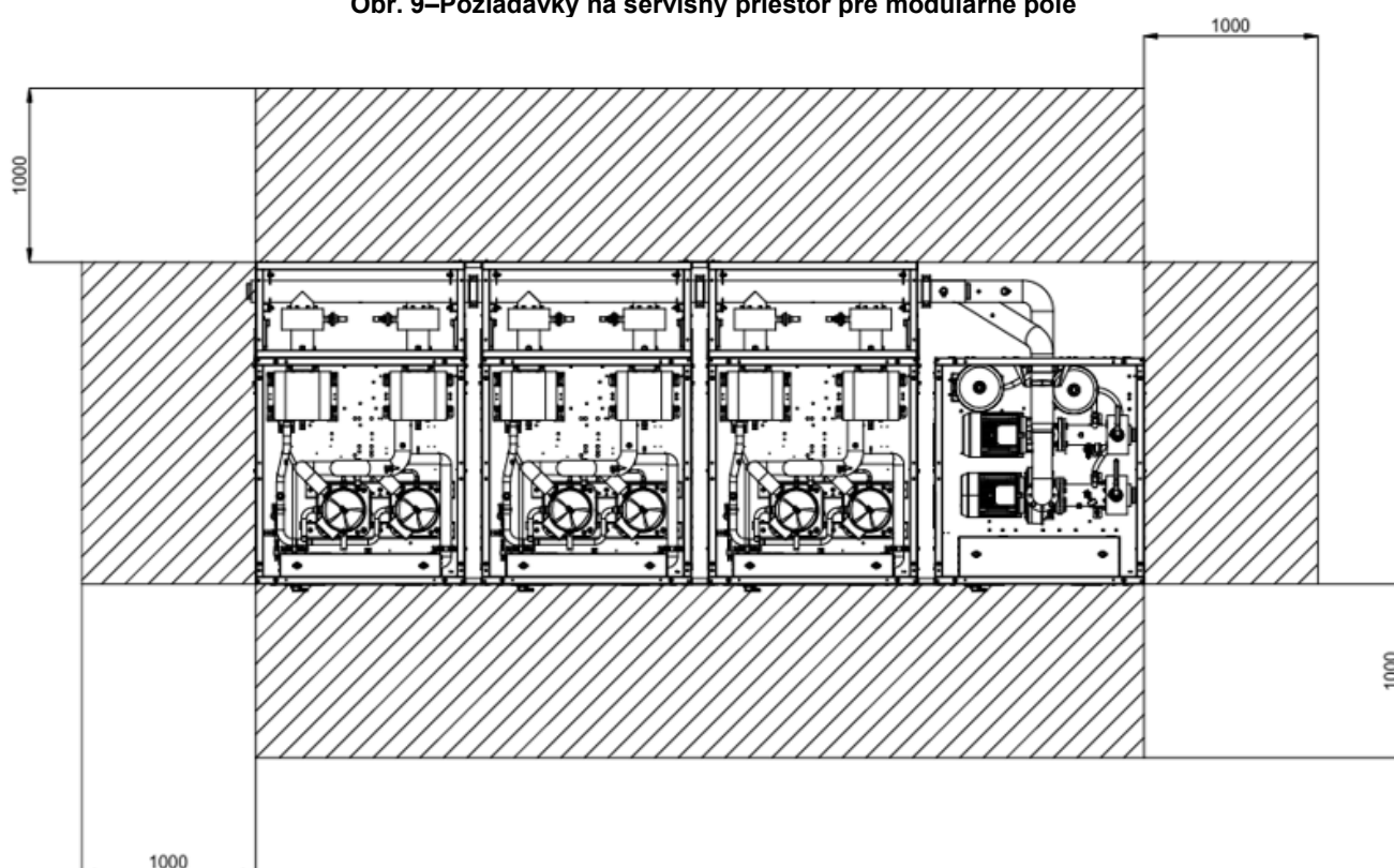
Obr. 9–Požiadavky na servisný priestor pre modulárne pole
