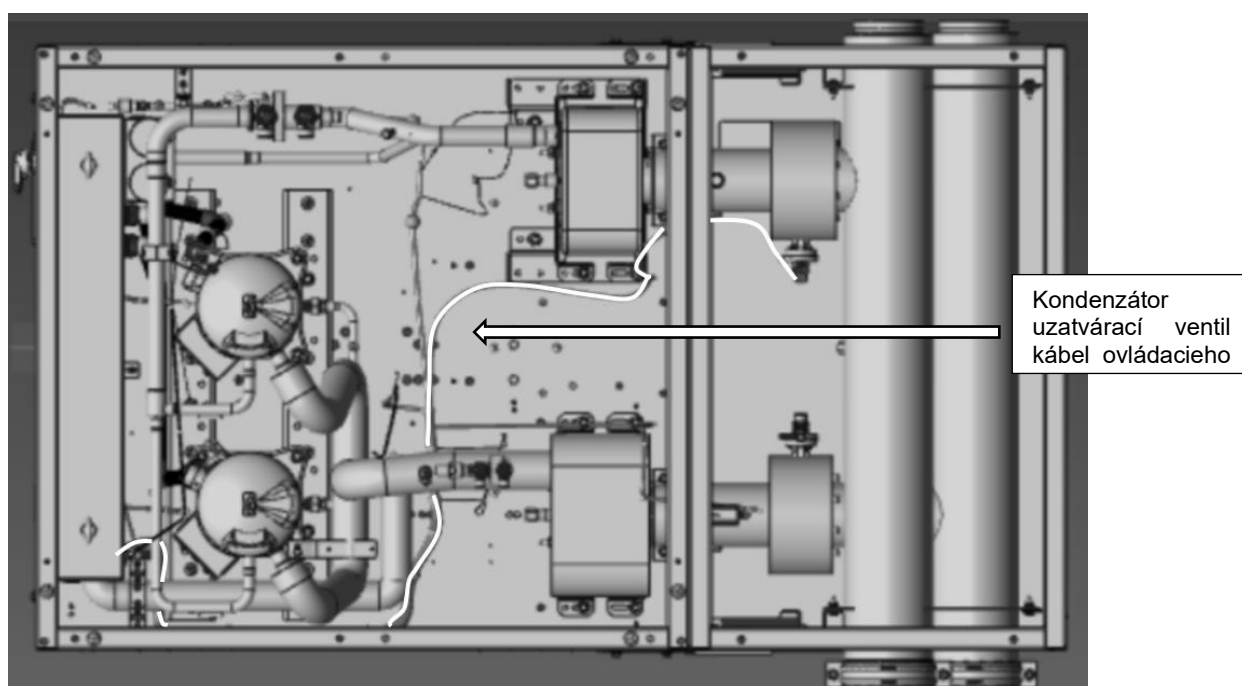
Obr. 40 – Vedenie kábla ovládača uzatváracieho ventilu kondenzátora
