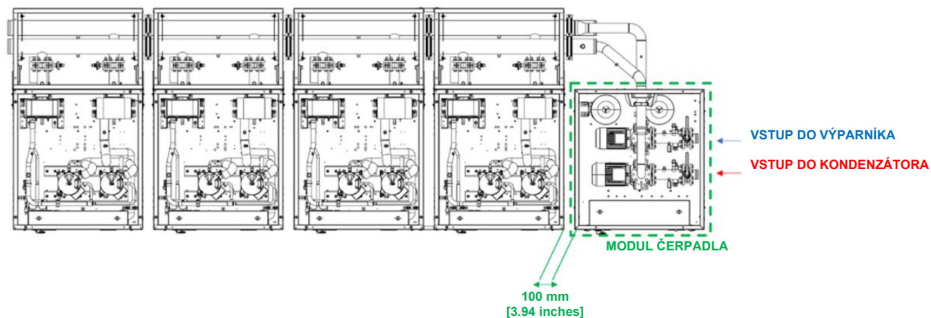
Obr. 46 – Inštalácia modulu čerpadla – podrobnosti o potrubí
