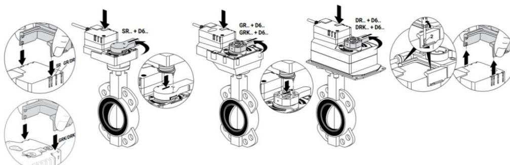
Obr. 33 – Montážne pokyny pre koncové spínače pohonu
