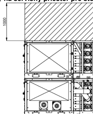
Obr. 10- Požiadavky na servisný priestor pre stohovanú konfiguráciu
