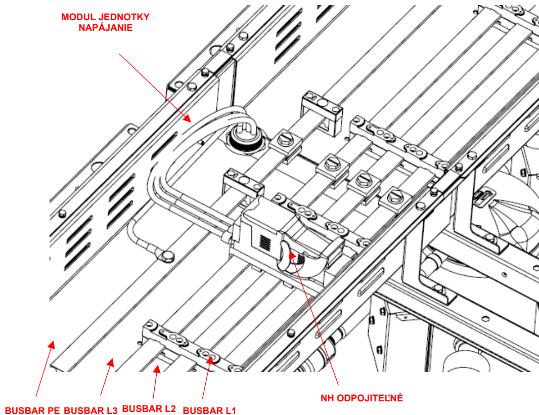
Obr. 60 – Detail elektrického pripojenia pre akýkoľvek iný modul jednotky
