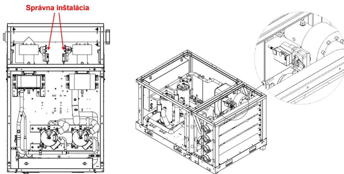
Obr. 34 – montážne indikácie pre pohon ventilu
