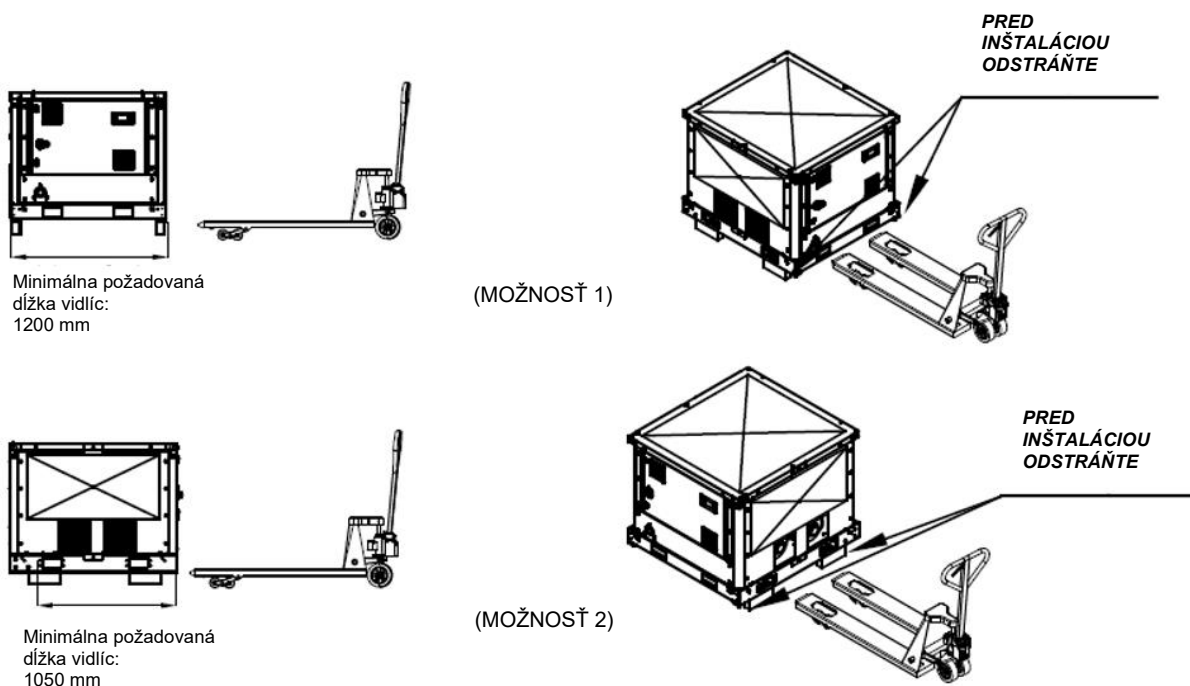
Obr. 51 – Manipulácia s modulom čerpadla pomocou paletového vozíka
