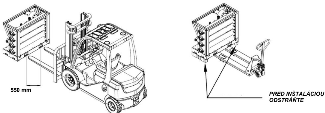
Obr. 47 – Manipulácia s modulom rozdeľovača
