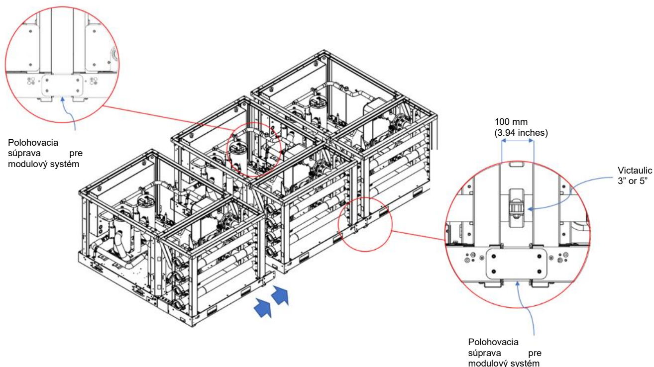
Obr. 29 – Pripojenie modulárnych systémov
