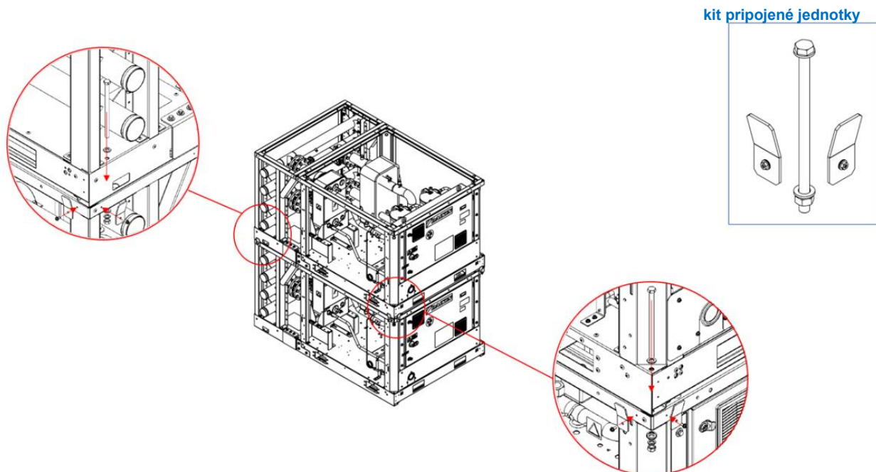
Obr. 43 – Montážne pokyny pre skladané jednotky
