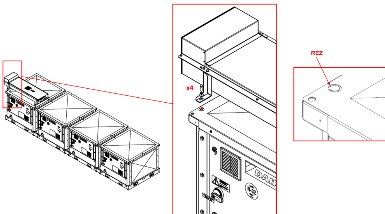
Obr. 55 – Upevnenie systému napájacej lišty k jednotke
