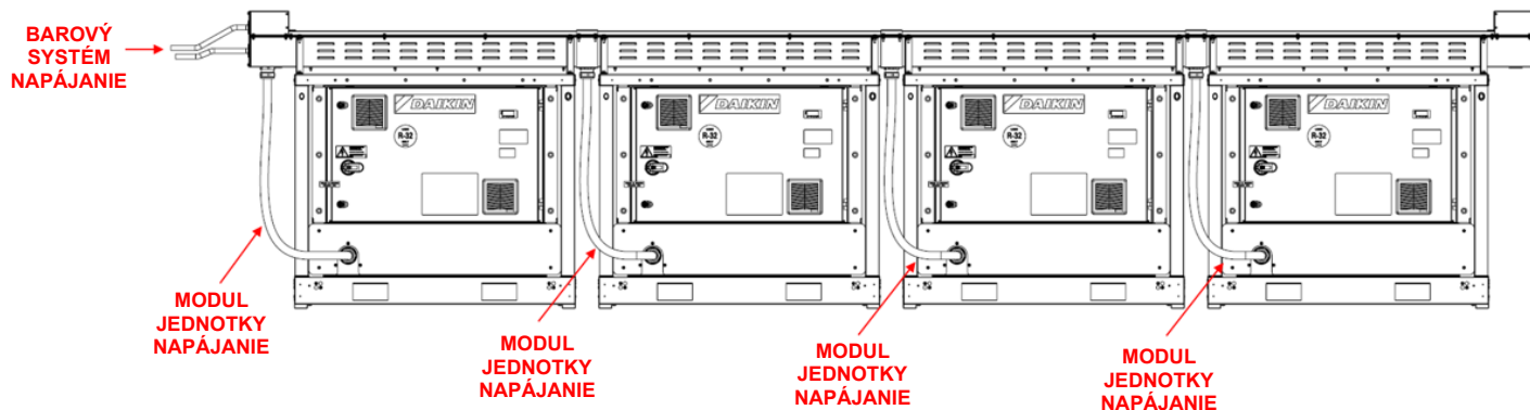
Obr. 54 – Podrobnosti o vedení káblov
