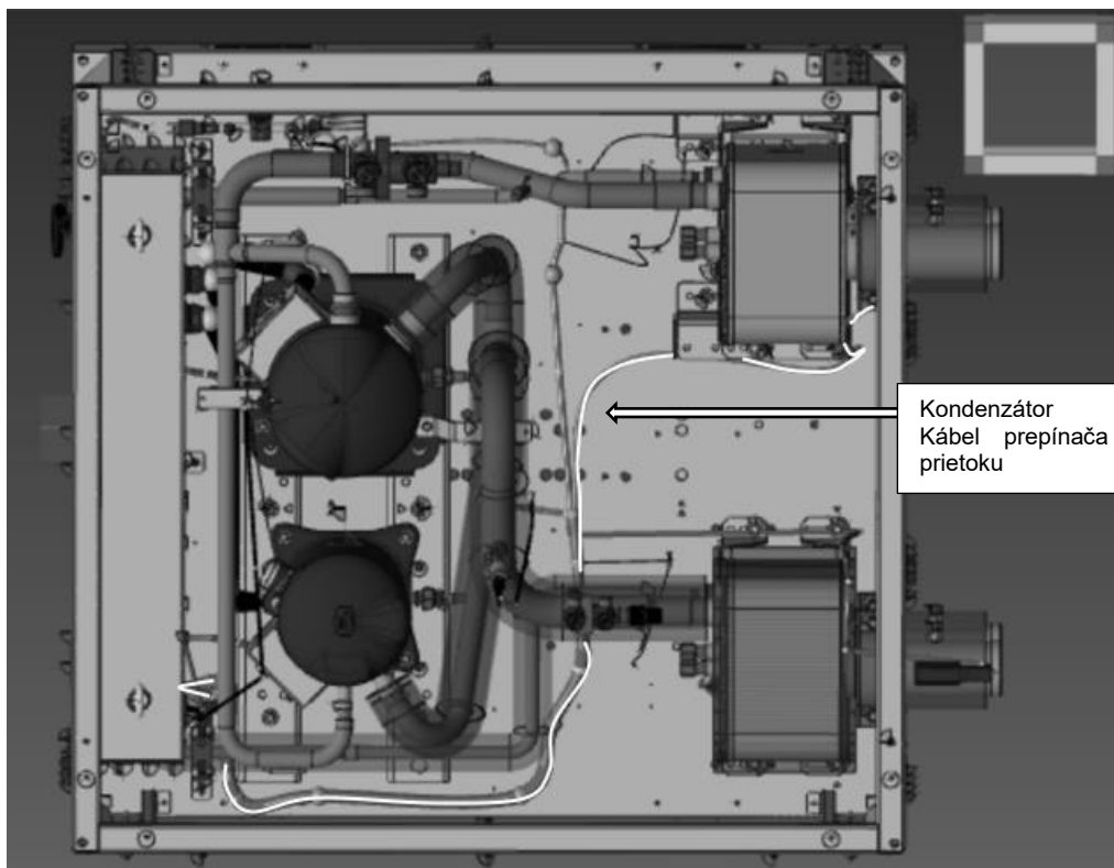
Obr. 18 – Vstupný bod elektrického panelu pre káble výparníka a prietokového spínača kondenzátora
