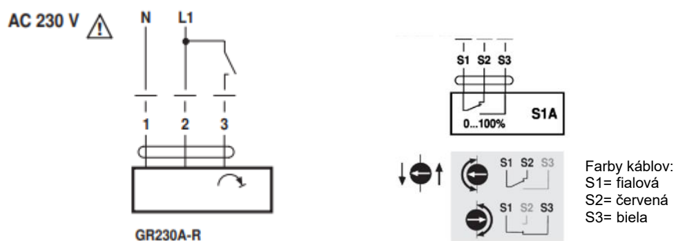
Obr. 35 – Schéma zapojenia motora (ľavý obrázok) a koncových spínačov (pravý obrázok)
