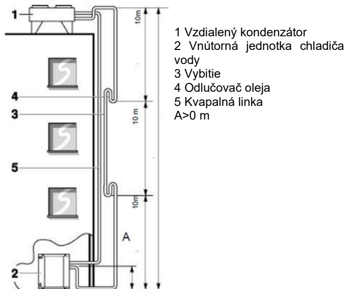
Obr. 20 – Pripojenie okruhu chladiva (1)
