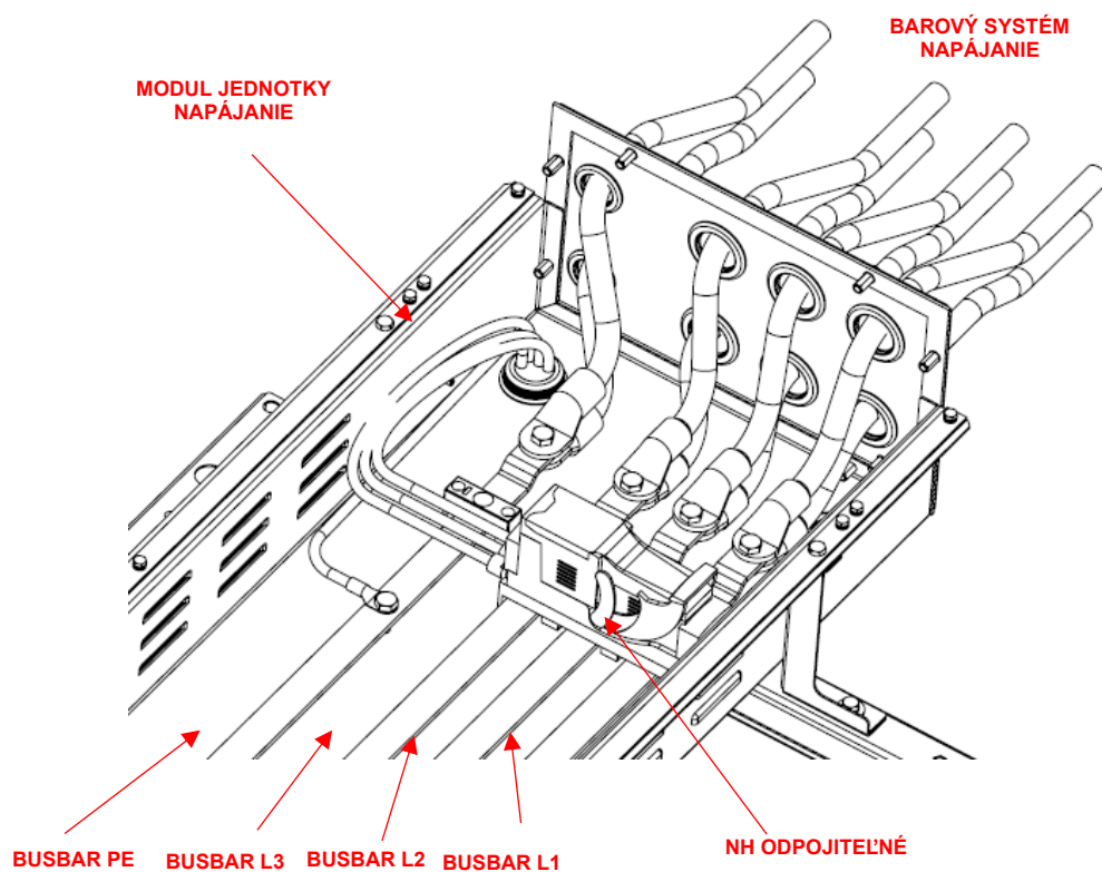
Obr. 59 – Detail elektrickej prípojky pre modul počiatkovej jednotky
