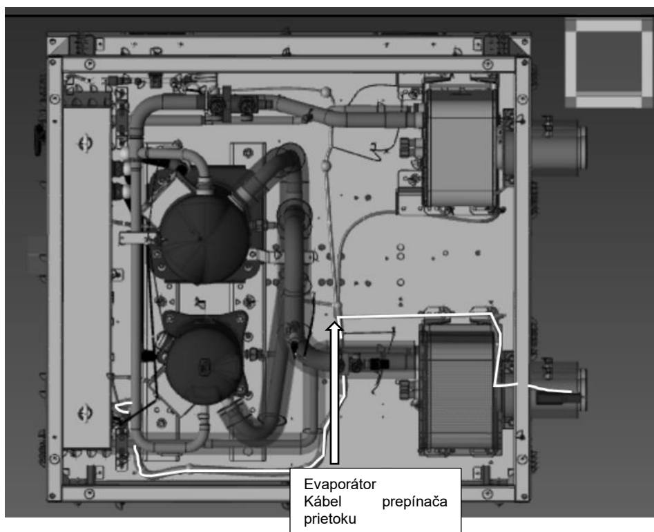
Obr. 16 – Vedenie káblov spínača prietoku výparníka
