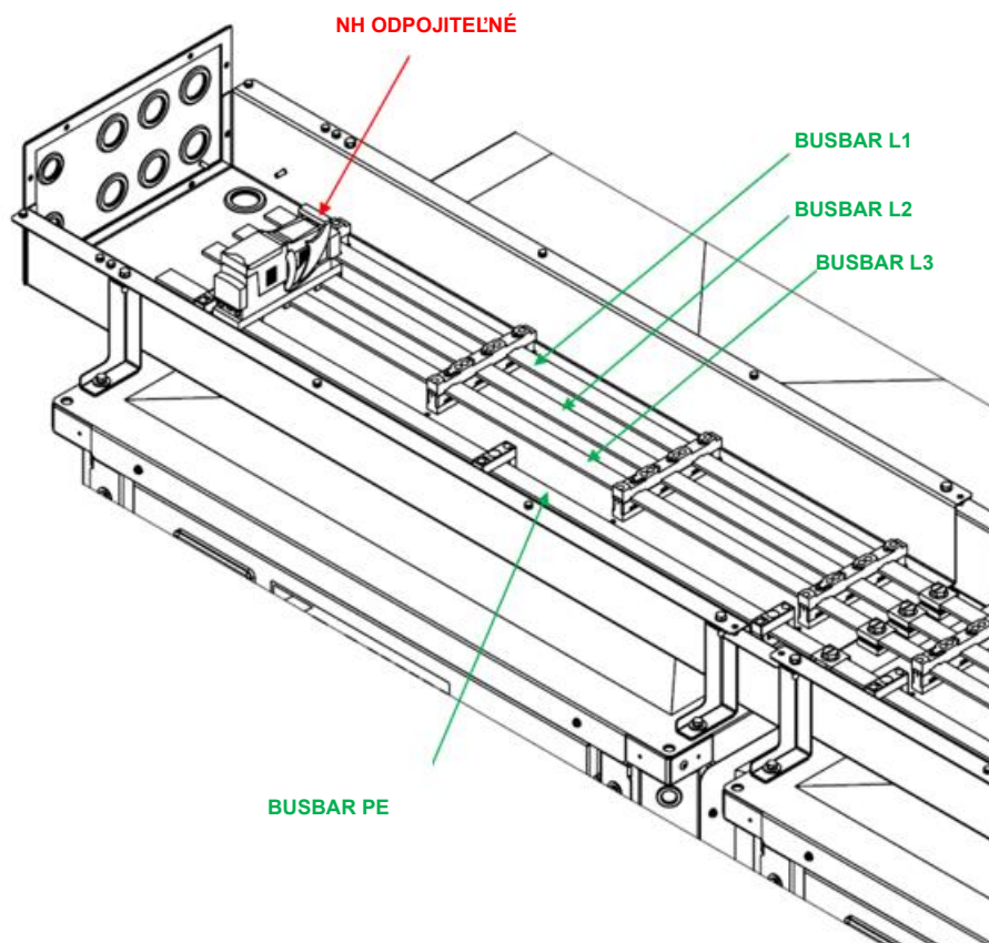
Obr. 58 – Detail poistiek a skrinky na vedenie káblov modulu silnoprúdovej tyče
