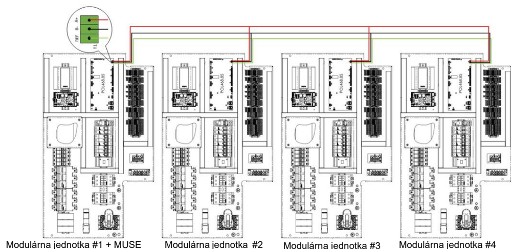
Obr. 64 – Pripojenie 4 PLC na rovnakú sieť Modbus
