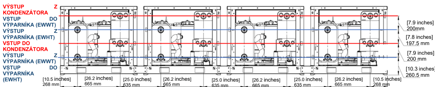
Obr. 28 – Konfigurácia vodovodného potrubia
