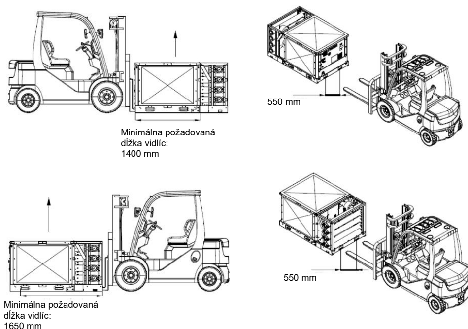
Obr. 48 – Manipulácia s modulmi jednotky a rozdeľovača
