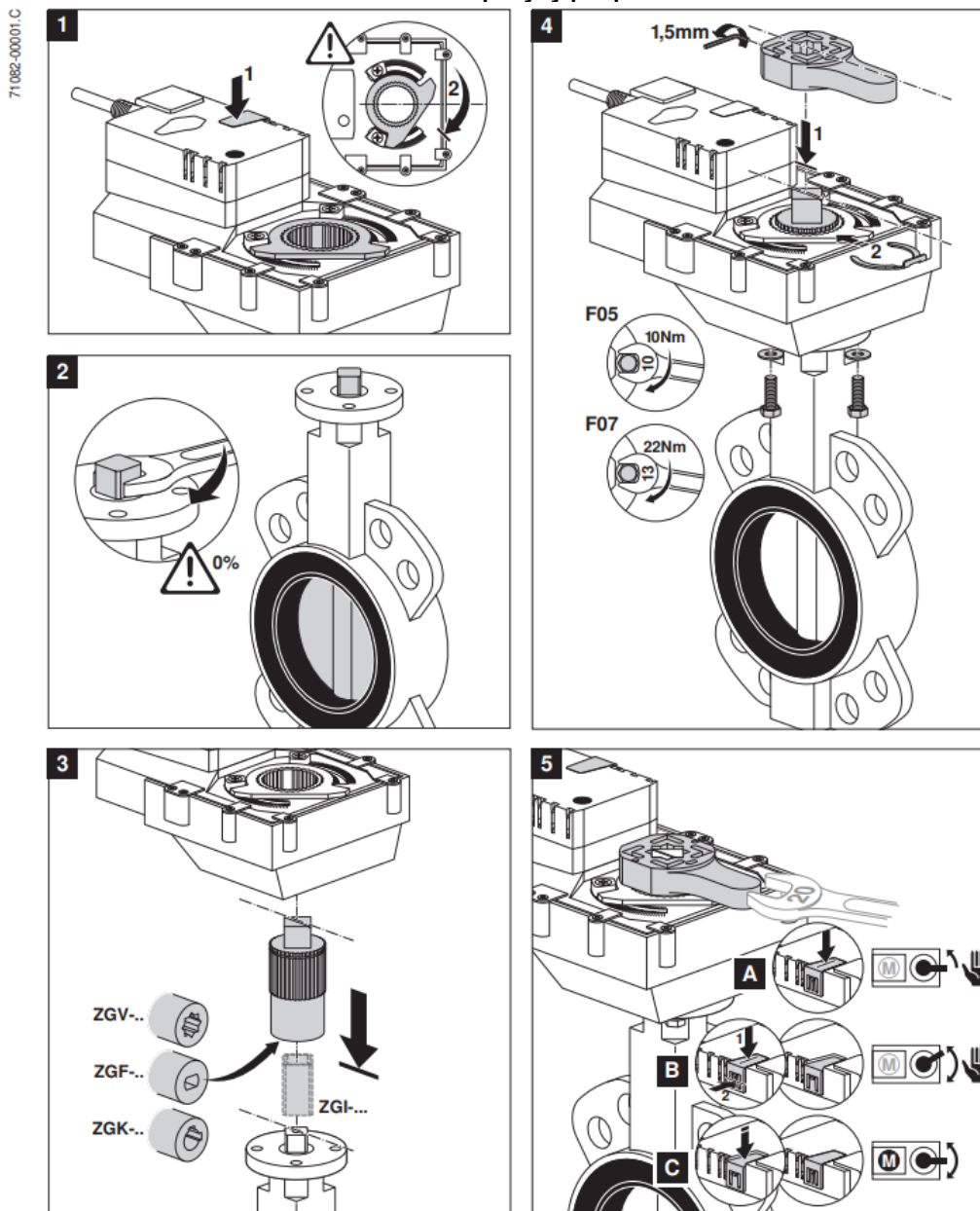
Obr. 32 – Montážne pokyny pre pohon ventilu
