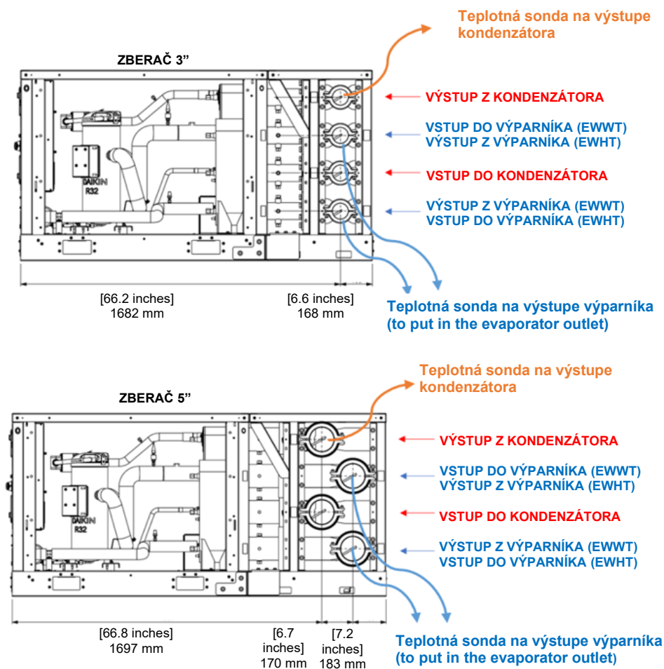
Obr. 62 – Polohy teplotných sond pre 3" a 5" rozdeľovač
