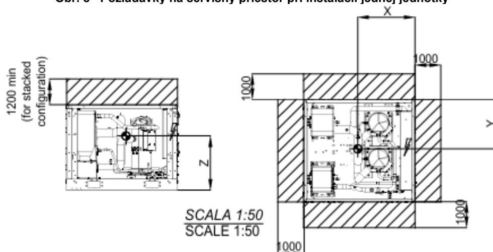
Obr. 8– Požiadavky na servisný priestor pri inštalácii jednej jednotky
