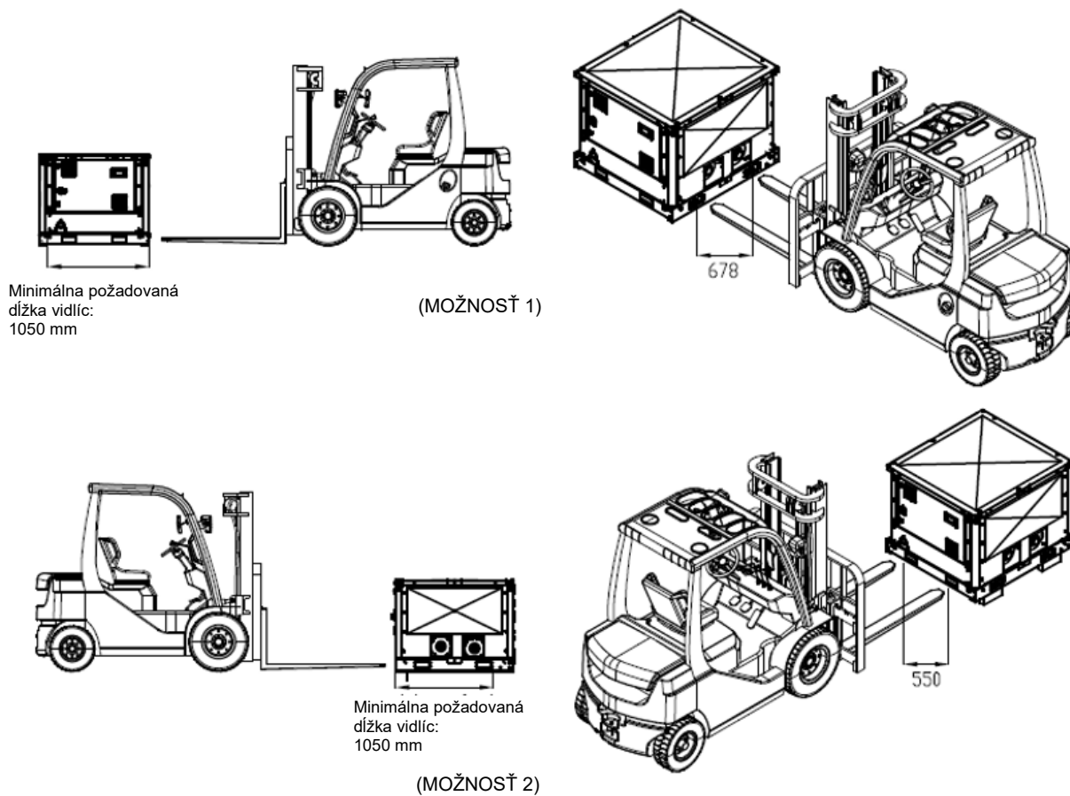
Obr. 50 – Manipulácia s modulom čerpadla pomocou vysokozdvížného vozíka
