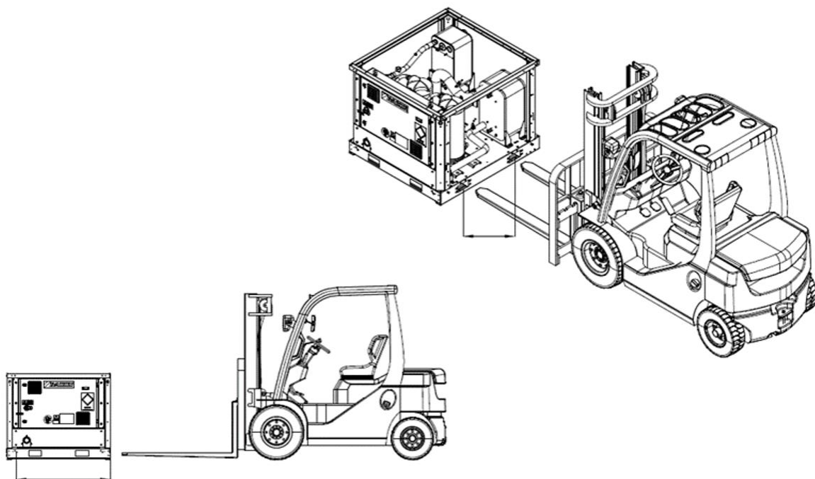
Obr. 11 – Manipulácia s jednotkou s jedným okruhom
