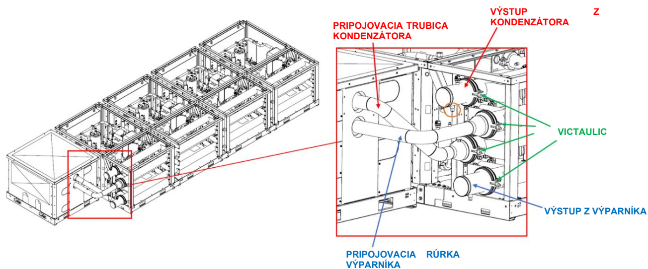
Obr. 46 – Inštalácia modulu čerpadla – podrobnosti o potrubí
