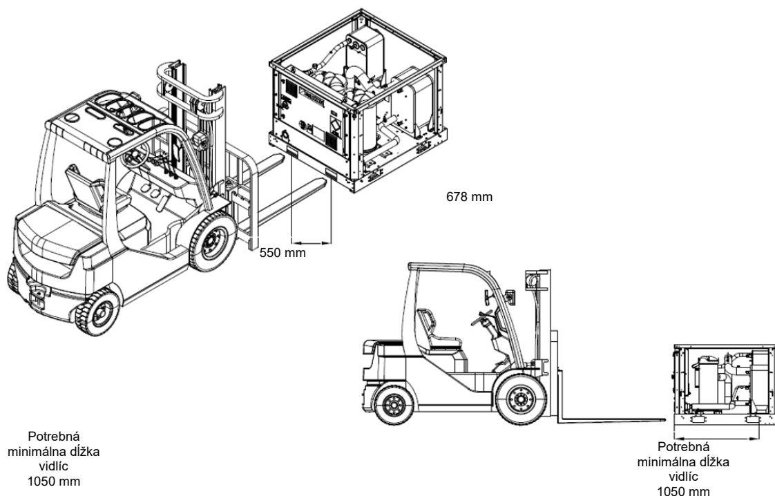
Obr. 12 – Alternatívny spôsob manipulácie s vysokozdvížným vozíkom
