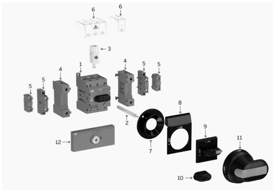
Obr. 23 – Pokyny na montáž rukoväte
