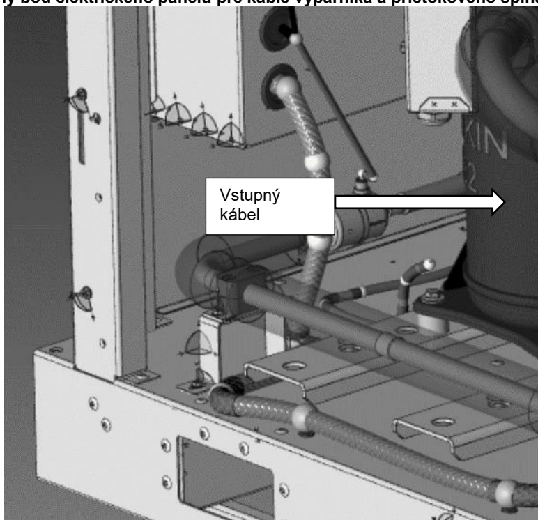
Obr. 18 – Vstupný bod elektrického panelu pre káble výparníka a prietokového spínača kondenzátora
