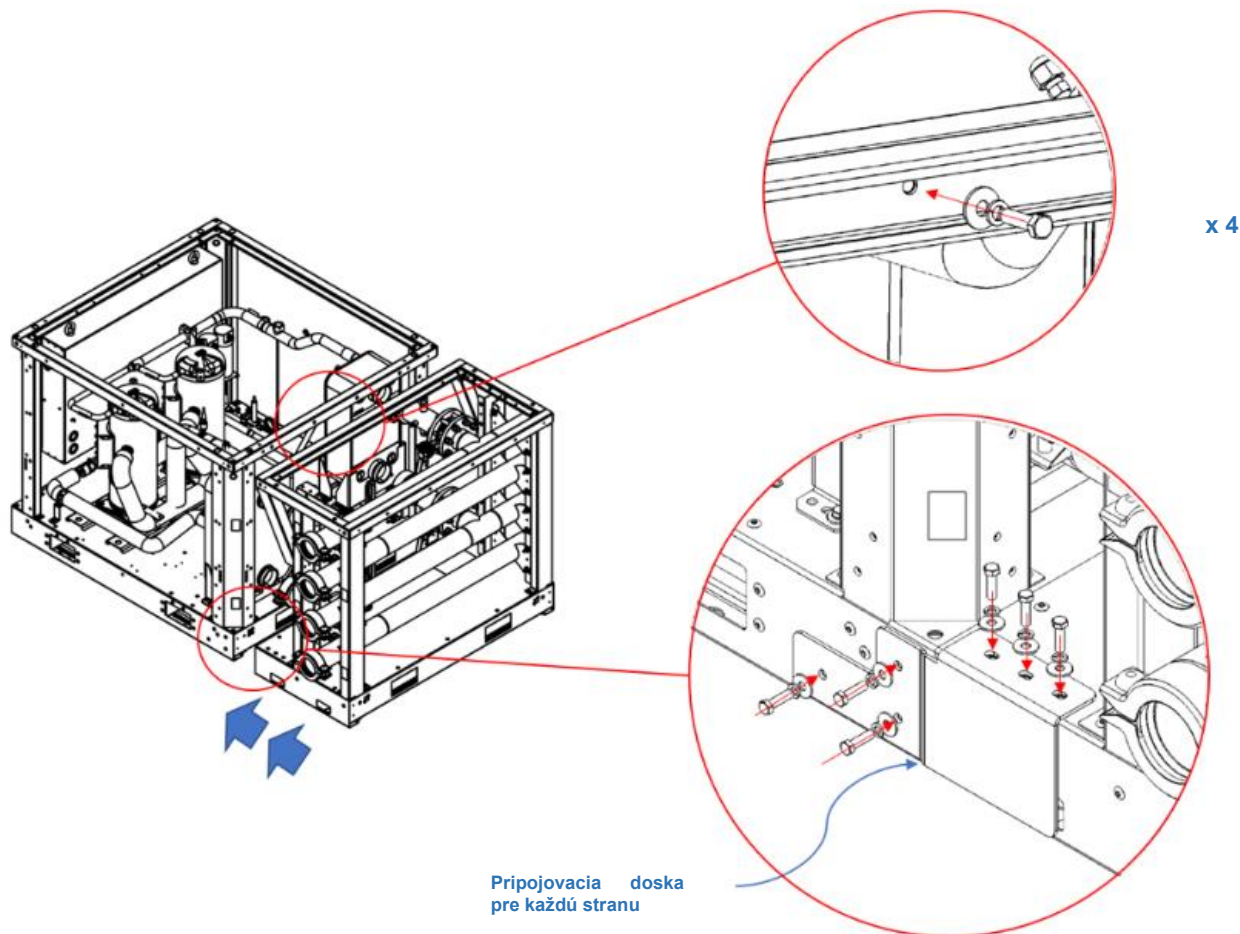
Obr. 26 – Pokyny na pripojenie medzi modulmi chladiča a rozdeľovača
