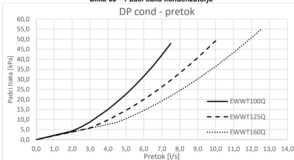
Slika 66 – Padci tlaka kondenzatorja
