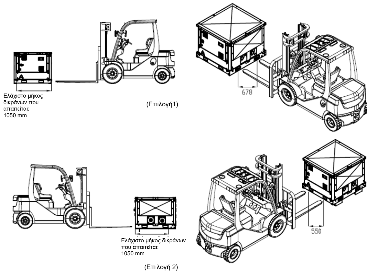
Εικόνα 50 – Χειρισμός μονάδας αντλίας με χρήση περονοφόρου
