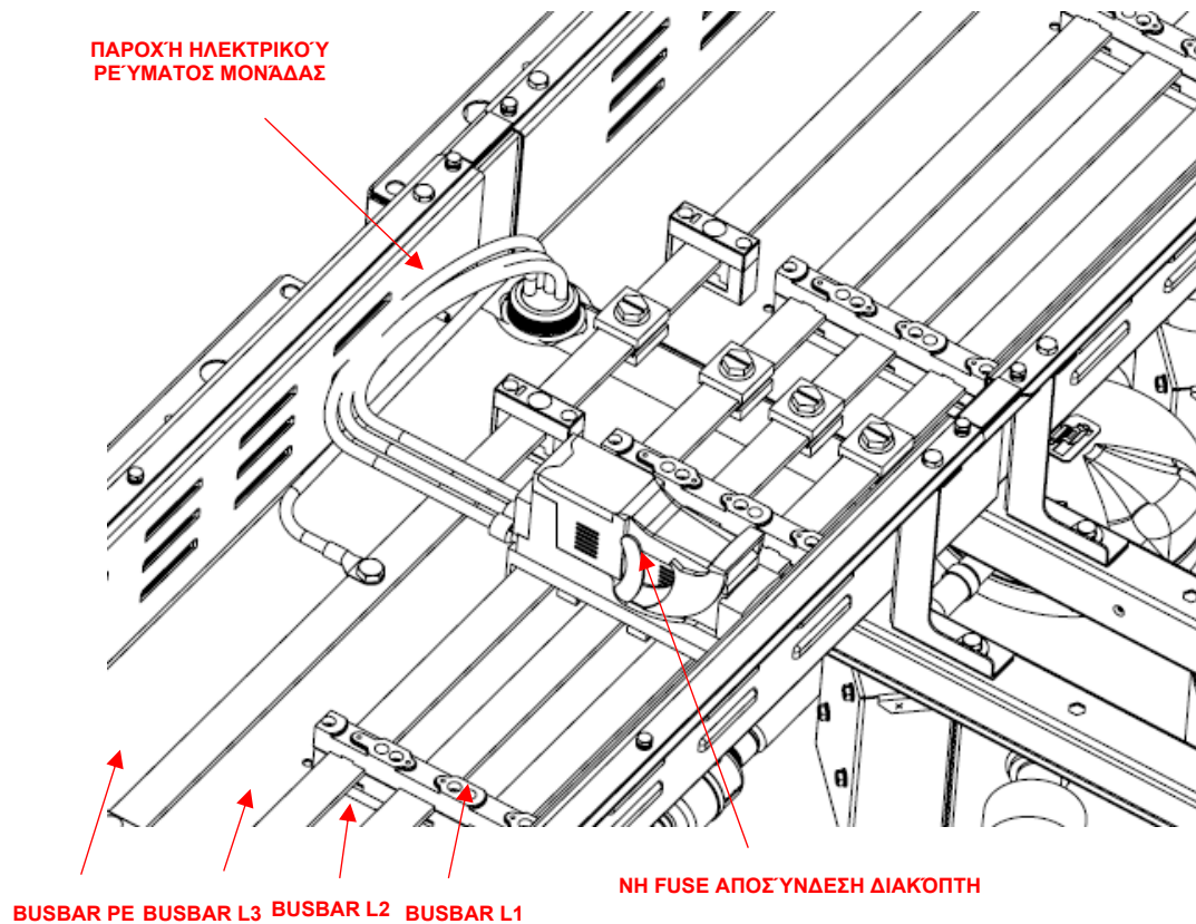
Εικόνα 60 – Λεπτομέρεια ηλεκτρικής σύνδεσης για κάθε άλλη μονάδα
