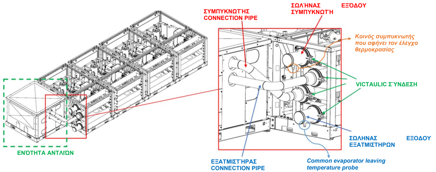
Εικόνα 63 – Λεπτομέρειες τοποθέτησης ανιχνευτών στους σωλήνες
