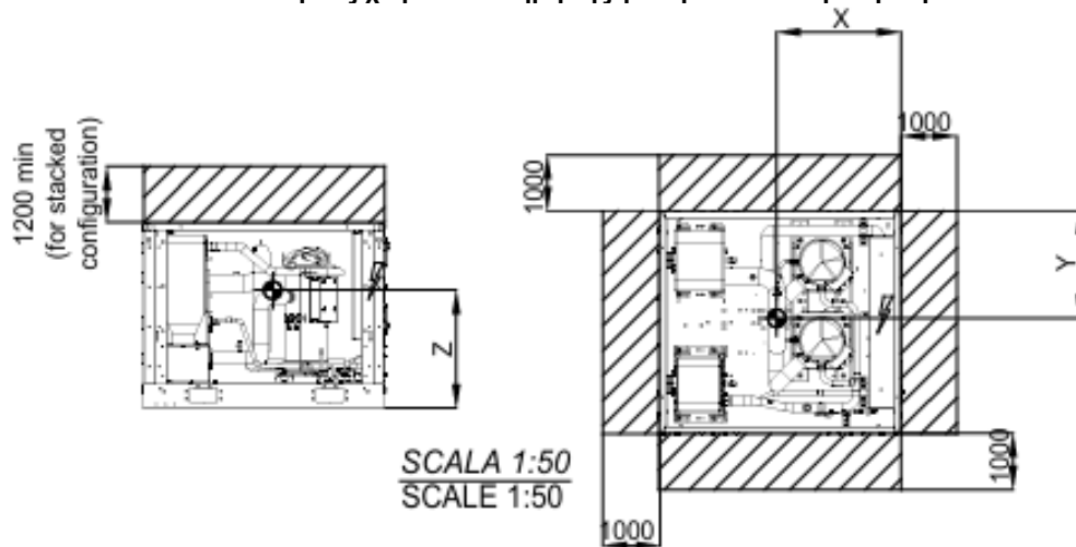
Εικόνα 8 – Απαιτήσεις χώρου συντήρησης για εγκατάσταση σε μία μονάδα
