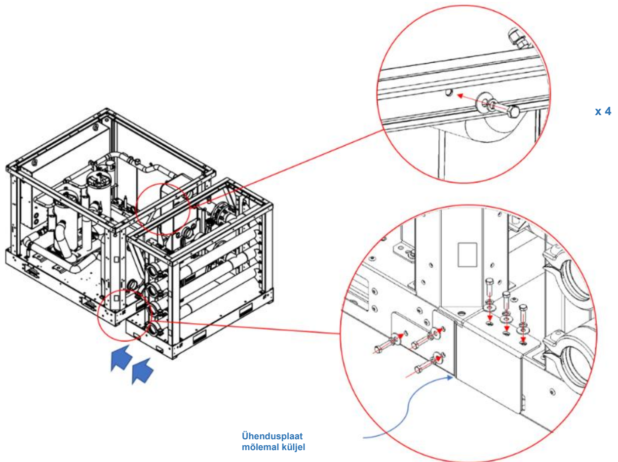
Joonis. 26 – Jahuti ja kollektori moodulite ühendamisjuhised
