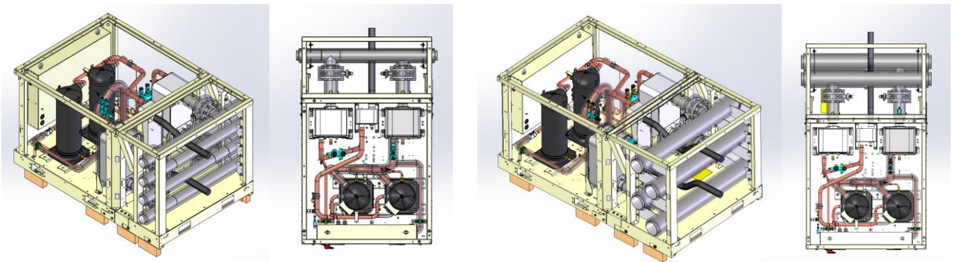
Joonis. 27 – PHR torud kollektori mooduliga (vasakul 3 tolli jaoks – paremal 5 tolliste kollektori torude jaoks)
