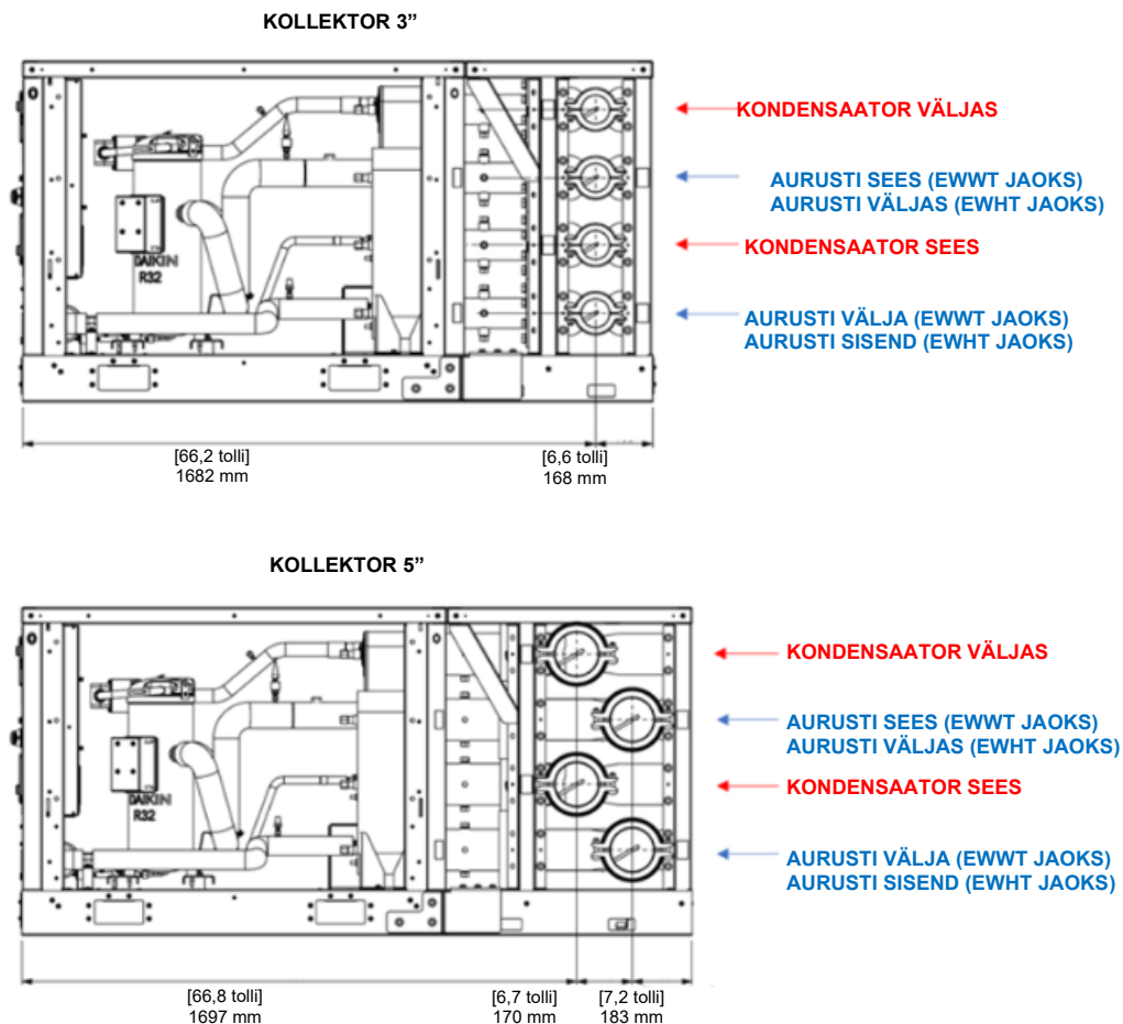
Joonis. 30 – Veekollektori suurused
