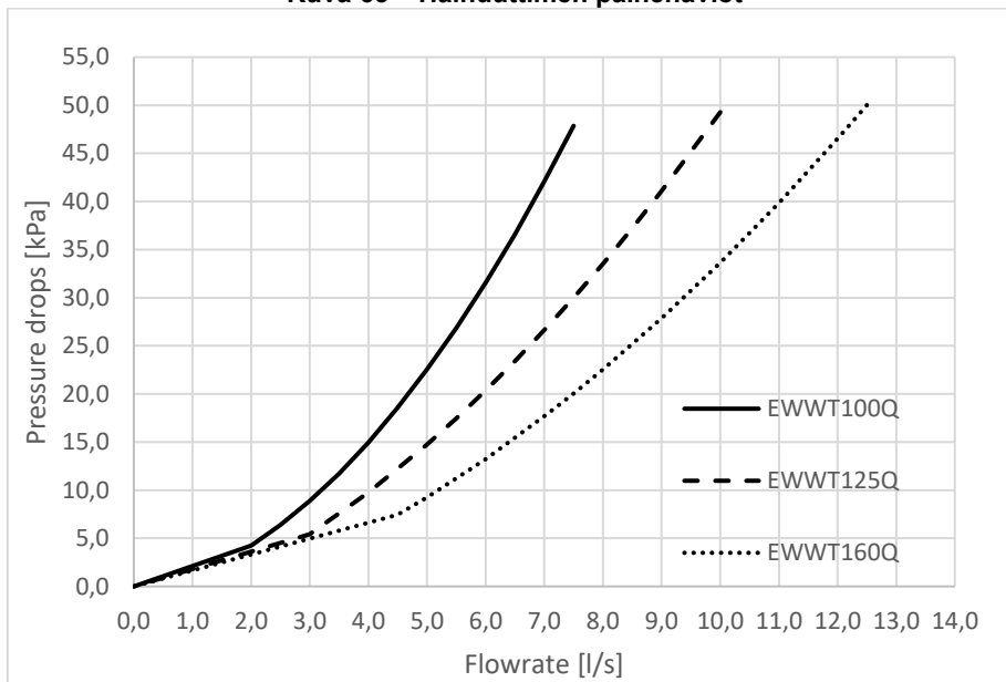
Kuva 66 – Lauhduttimen painehäviöt
