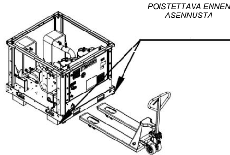
Kuva 13 – Vaihtoehtoinen käsittelytapa lavansiirtovaunulla
