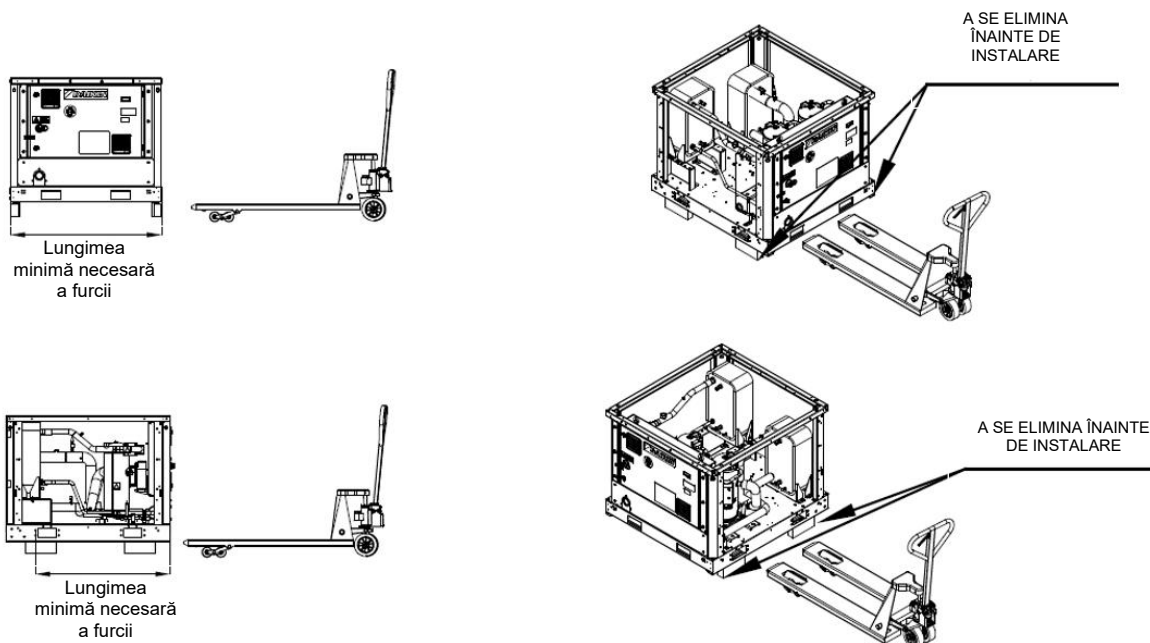
Fig. 13 – Metodă alternativă de manevrare cu transpalet
