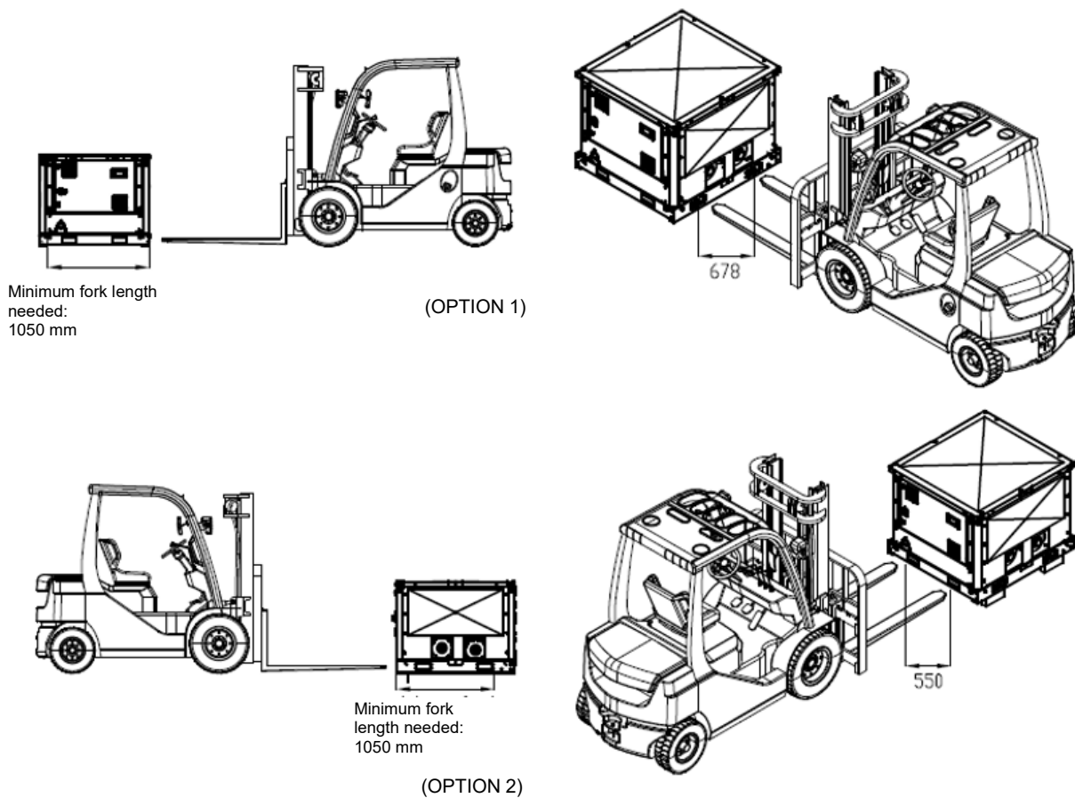
Fig. 50 – Manevrarea modului pompei cu ajutorul motostivuitoarelor
