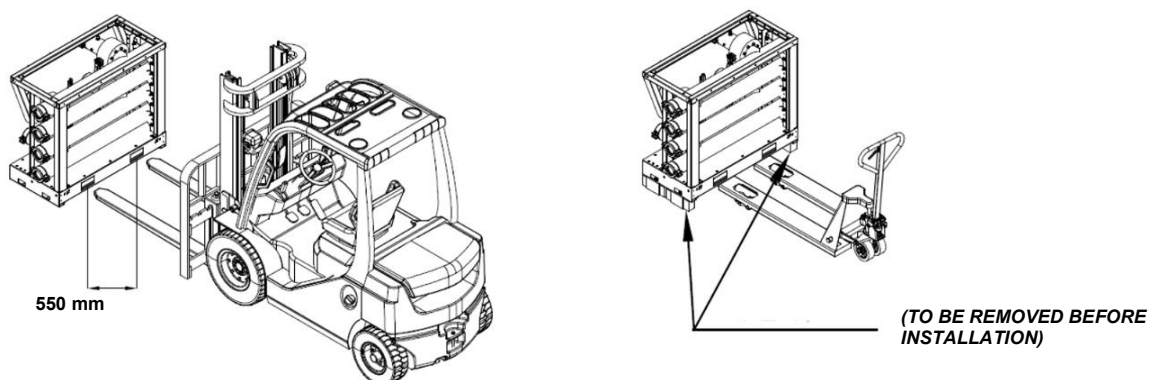
Fig. 47 – Manevrarea moduluiui colectorului
