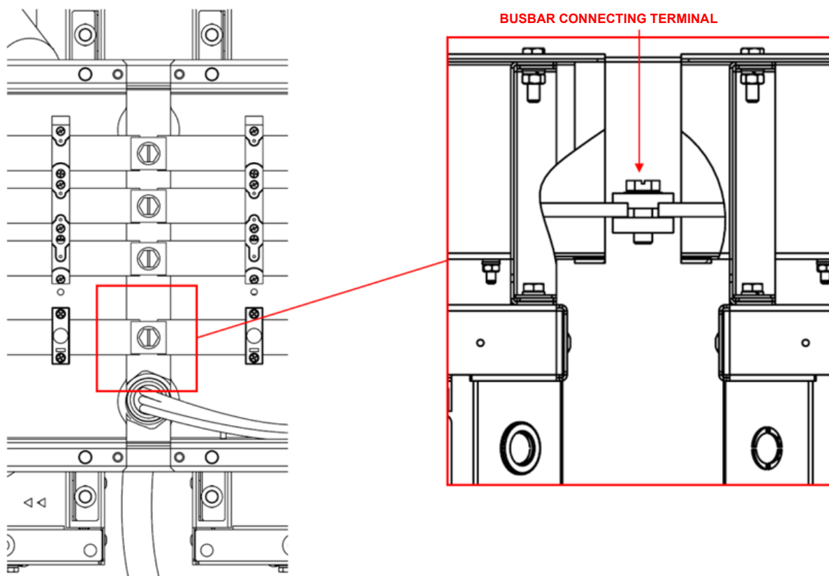
Fig. 57 – Detalii de conectare a modulelor de prelungitoare de alimentare
