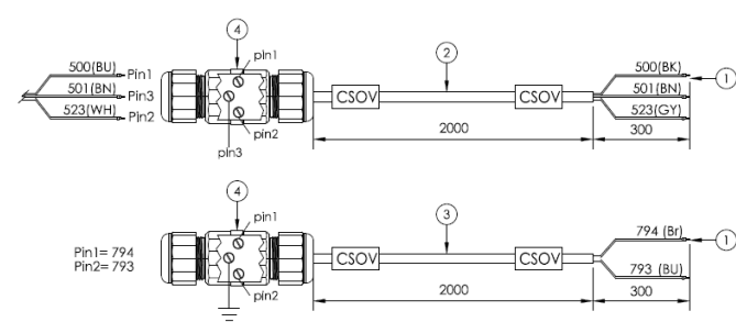
Fig. 37 – Adaptoare de cablu pentru mecanismul de acționare a supapei de închidere a condensatorului și limitatoare de cursă
