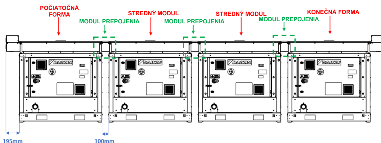
Obr. 53 – Káble smerujúce medzi tyčovým systémom a jednotkou
