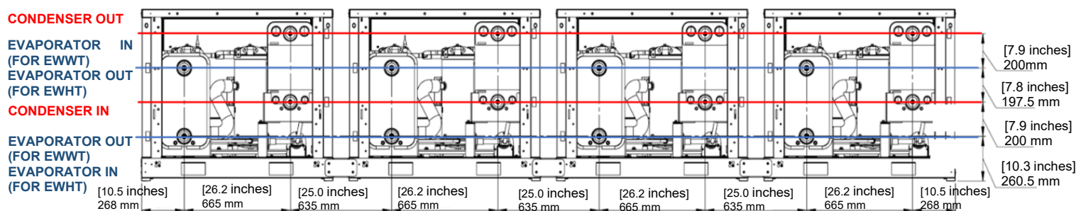
Figur 28– Vattenrörledningens konfiguration
