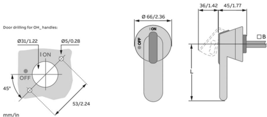
Figur 24– Detaljer över det pistolformade handtaget
