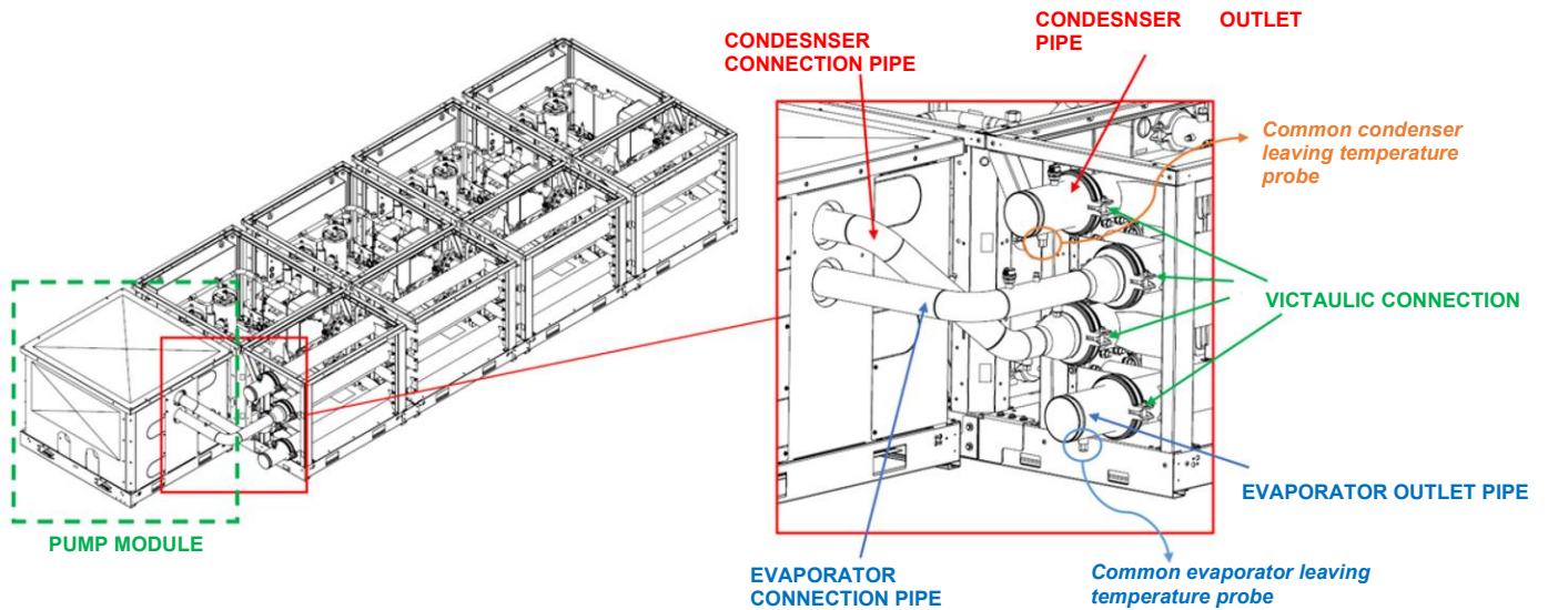
Figur 63– Detaljer över givarnas placering på rören
