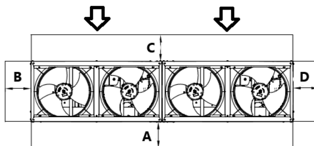
Obrázek 8 – Jednotka DUAL
