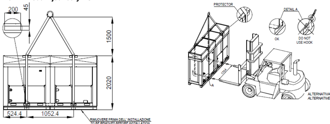
Obrázek 4 – Zvedání jednotky DUAL
