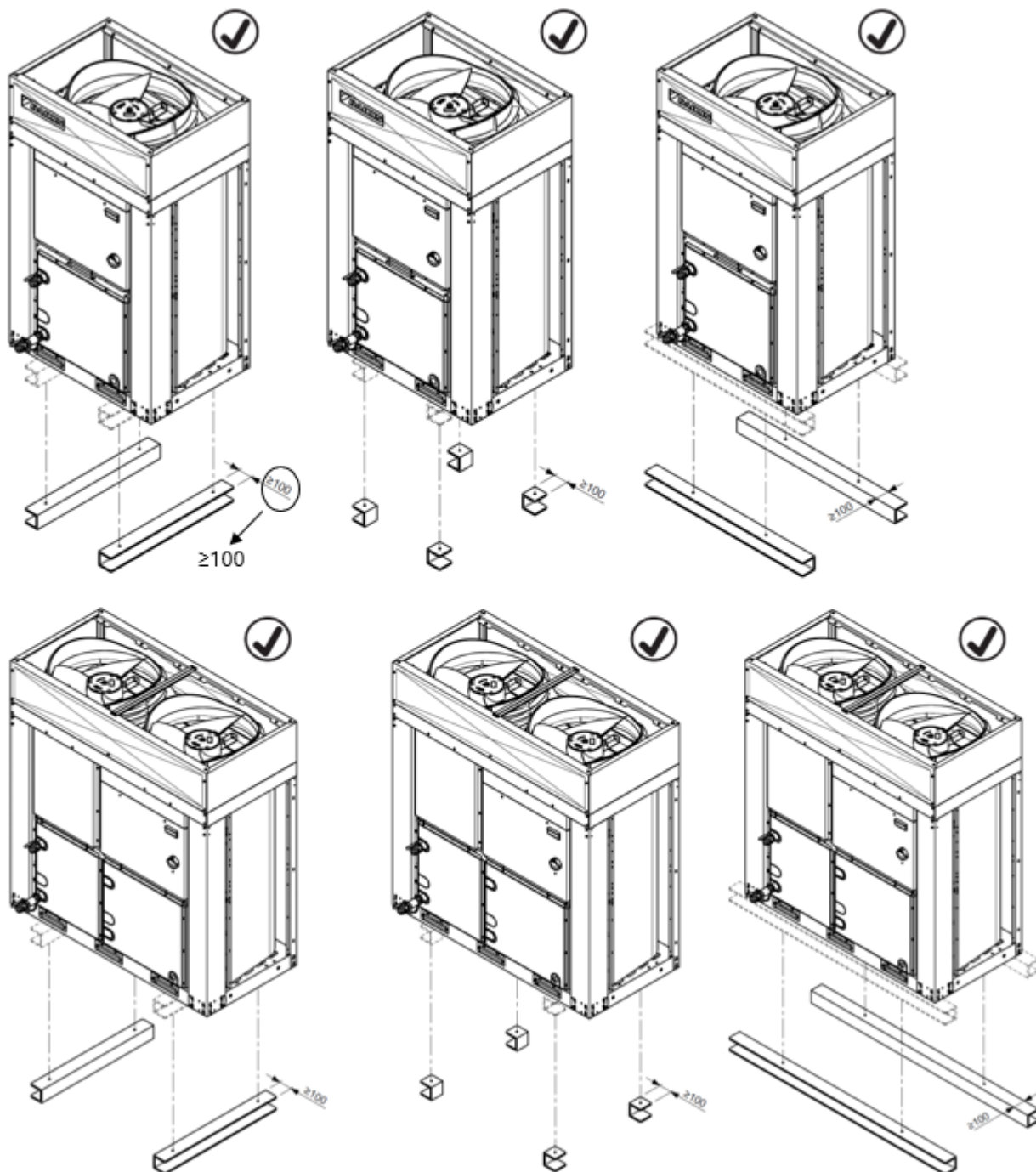
Obrázek 5 – Vyvážení jednotky MONO
