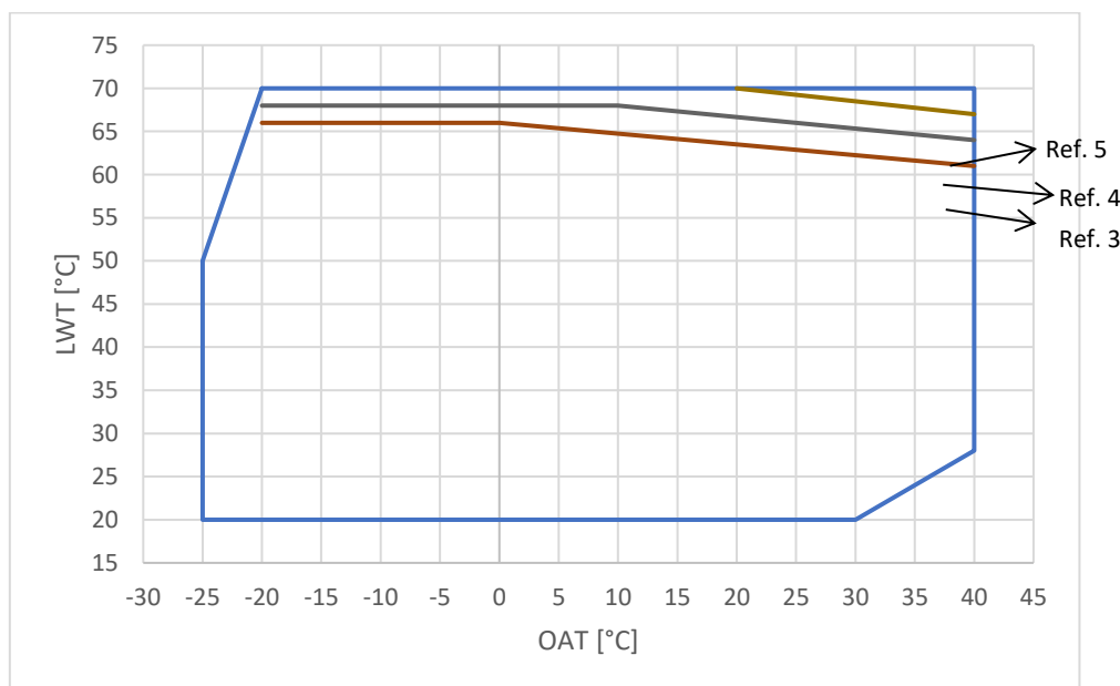
Rysunki 2 - Ograniczenia robocze EWYE-CZ
