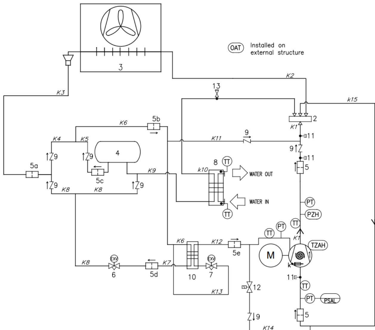
Figura 16 - Esquema do circuito de refrigeração (P&ID) para a unidade EWYE ~CZ circuito MONO
