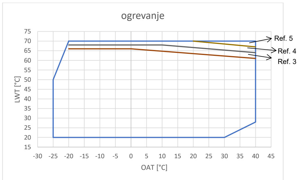
Slika 2 – Omejitve delovanja za EWYE-CZ v načinu ogrevanja
