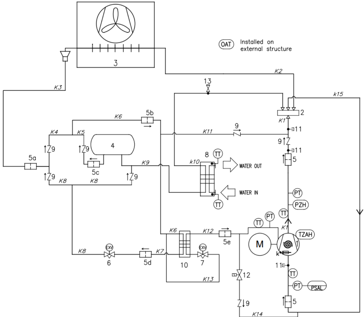
Εικόνα 16 - Διάγραμμα κυκλώματος ψυκτικού μέσου (P&ID) για μονάδα MONOY κυκλώματος EWYE~CZ
