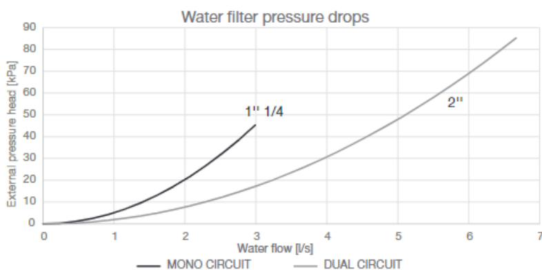
Obrázek 13 - Poklesy tlaku vodního filtru
