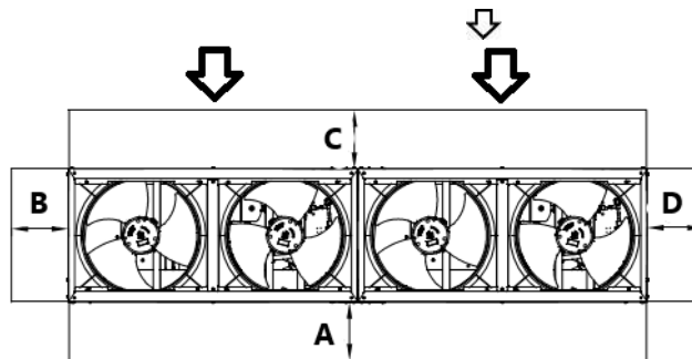
Abbildung 8 – DUAL-Einheit
