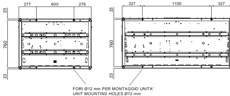
Abbildung 7 – Anordnung der Montagebohrungen (Ansicht von unten)
