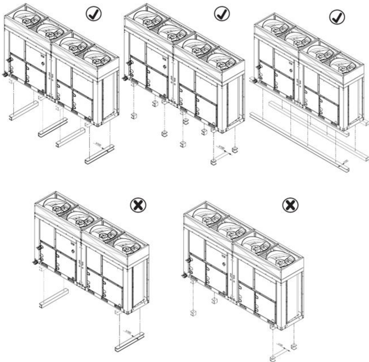
Abbildung 6 – Anheben der DUAL-Einheit
