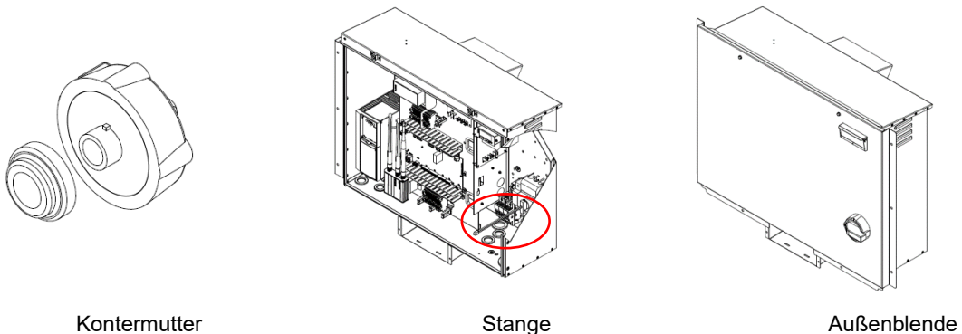
Kontermutter
