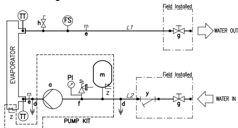
Abbildung 12 – Hydraulikschema
