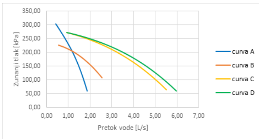
Εικόνα 14 - - Εξωτερική κεφαλή πίεσης αντλίας μικρής ανύψωσης
