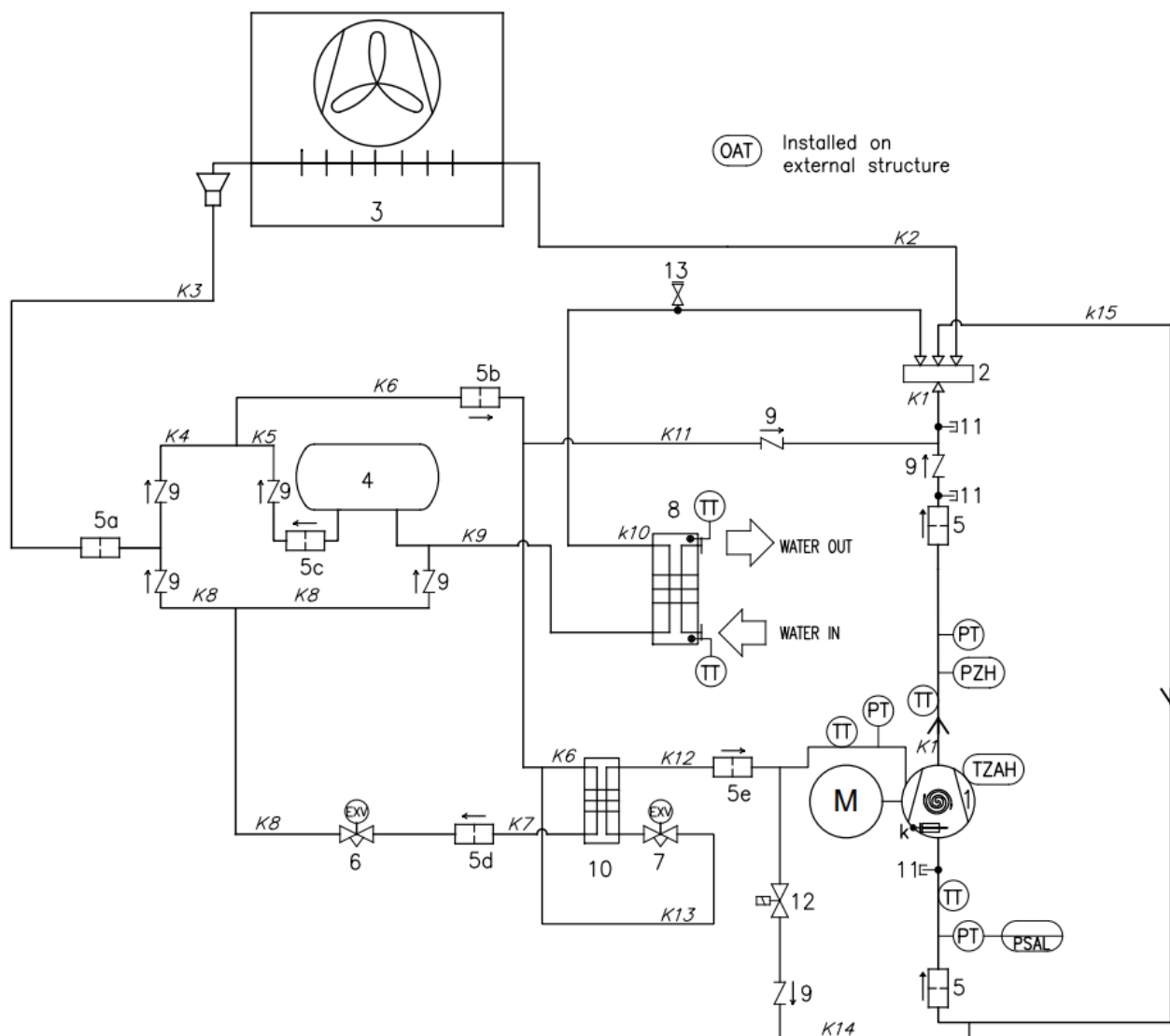
Εικόνα 16 - Διάγραμμα κυκλώματος ψυκτικού μέσου (P&ID) για μονάδα ΜΟΝΟΥ κυκλώματος ΕWYΕ~CZ
