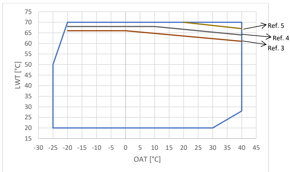
Εικόνα 2 - Όρια λειτουργίας στο EWYE-CZ
