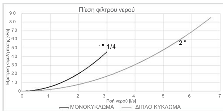
Εικόνα 13 - Πτώσεις πίεσης του φίλτρου νερού
