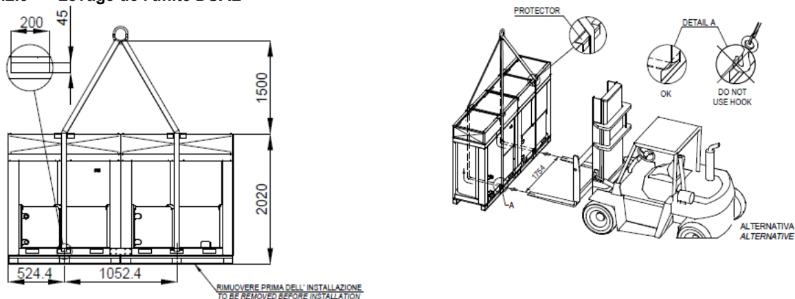
Figure 4 – Levage de l'unité DUAL
