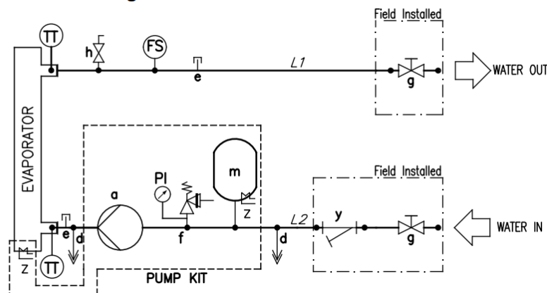
Figura 12 –Schema idraulico
