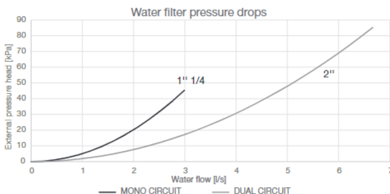
Afbeeldingen 13 - Drukvermindering waterfilter
