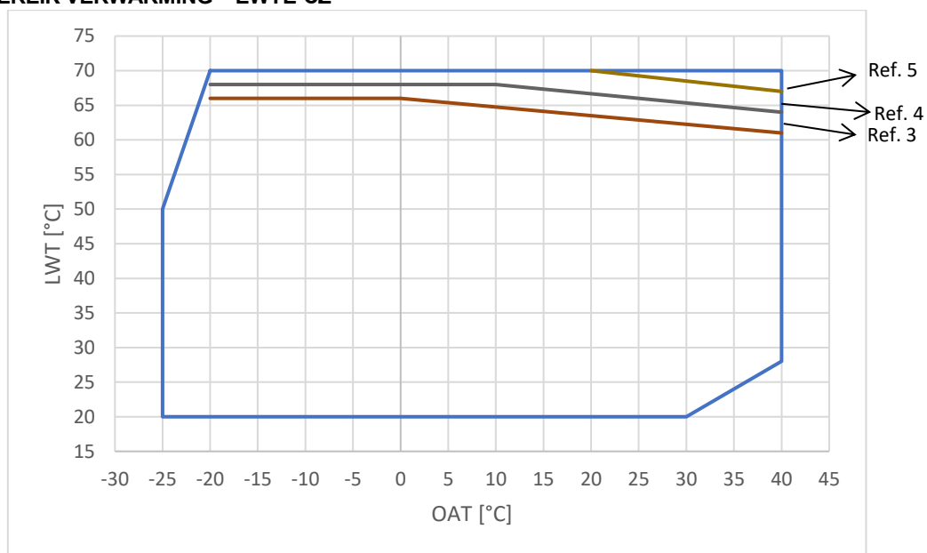
Afbeeldingen 2 - werkingssbereik verwarming EWYE-CZ
