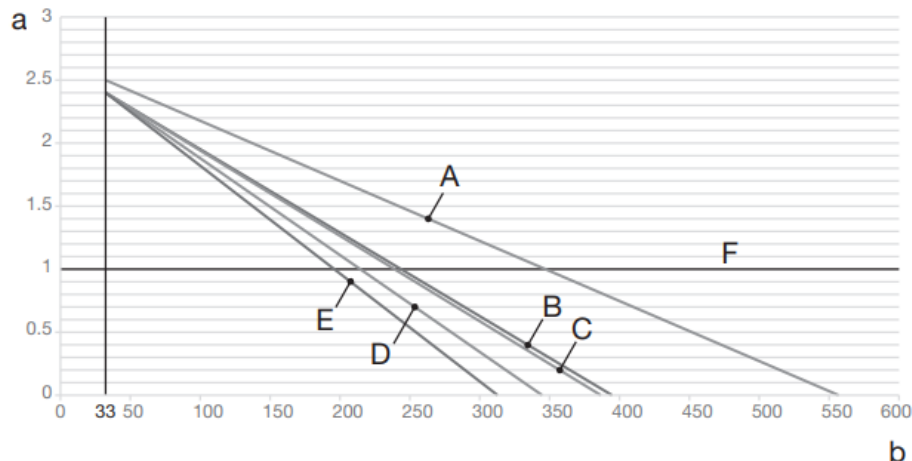
Afbeeldingen 15 - Begindruk van het expansievat op basis van de maximale waterhoeveelheid
