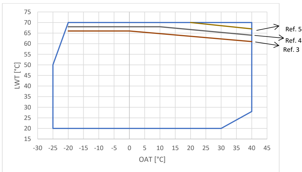
Rysunki 2 - Ograniczenia robocze EWYE-CZ
