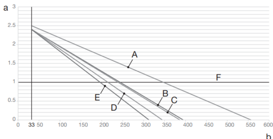
Rysunki 15 - Ciśnienie początkowe w zbiorniku rozprężnym w zależności od maksymalnej objętości wody
