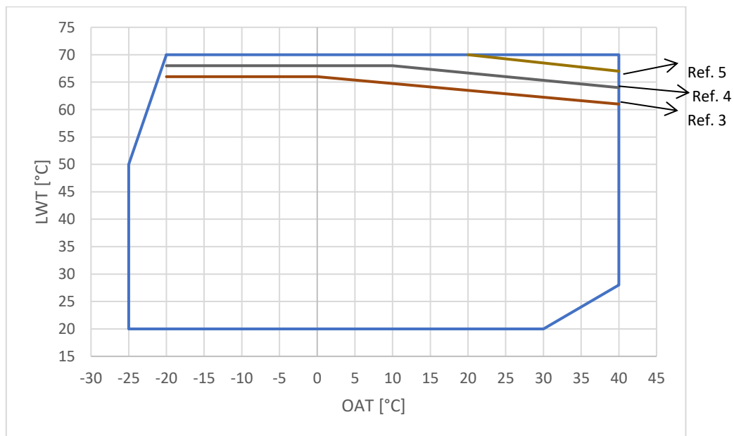
Figura 2 - Limites de operação no EWYE-CZ
