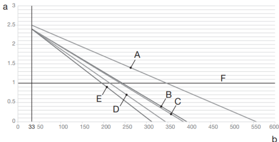
Figura 15 - Pressão inicial do vaso de expansão com base no volume máximo de água
