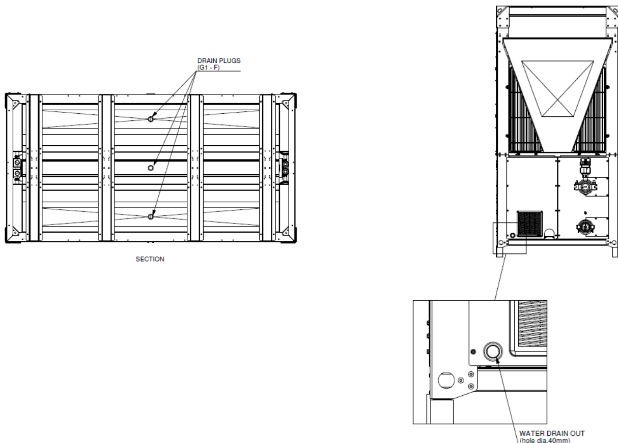
Afbeelding 31 – Condensaatopvangbak
