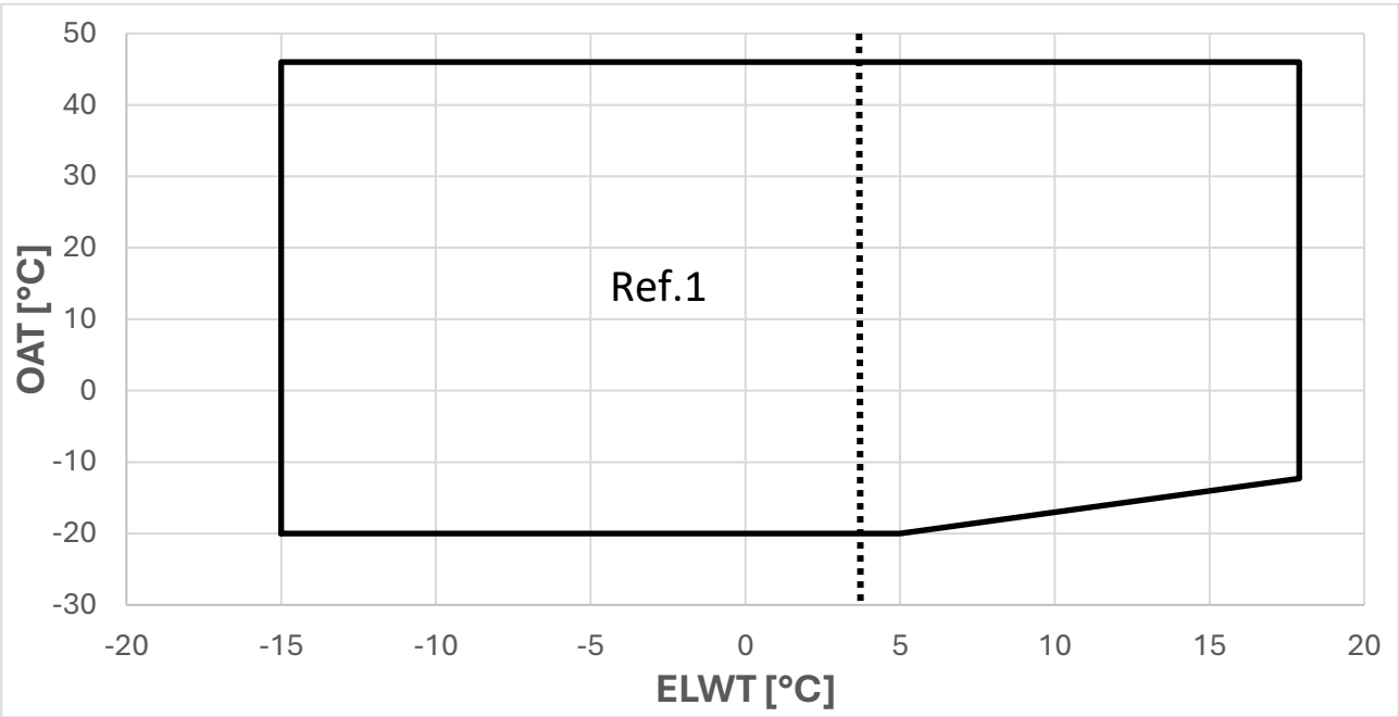
Afbeelding 35 - Bedieningslimieten koelmodus
