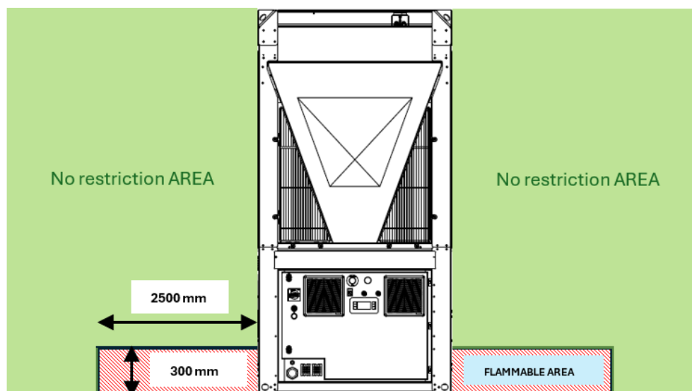
Afbeelding 13 – Ontvlambaar gebied
