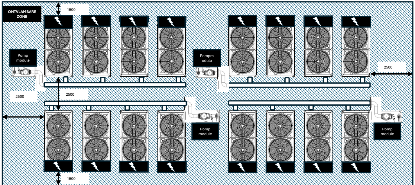
Afbeelding 18 - Multi-array met eenheden geplaatst met waterzijden naar elkaar toe
