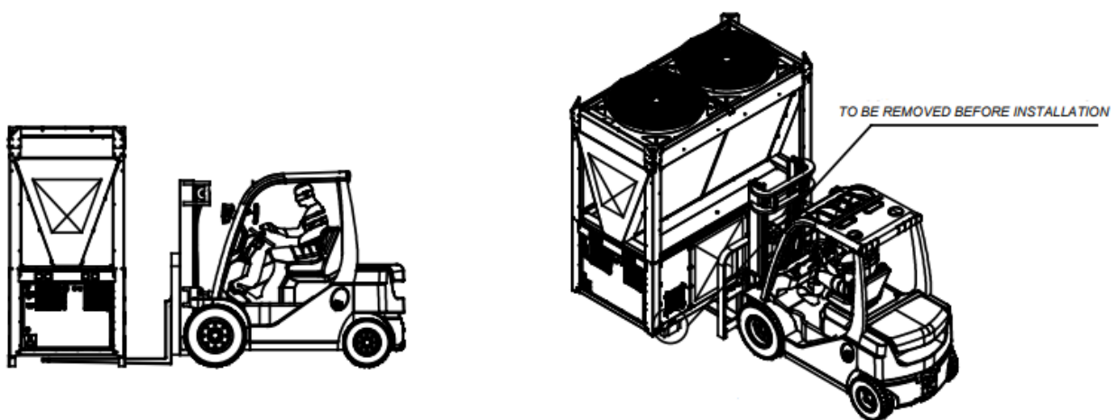
Afbeelding 20 – Hefinstructies met vorkheftruck
