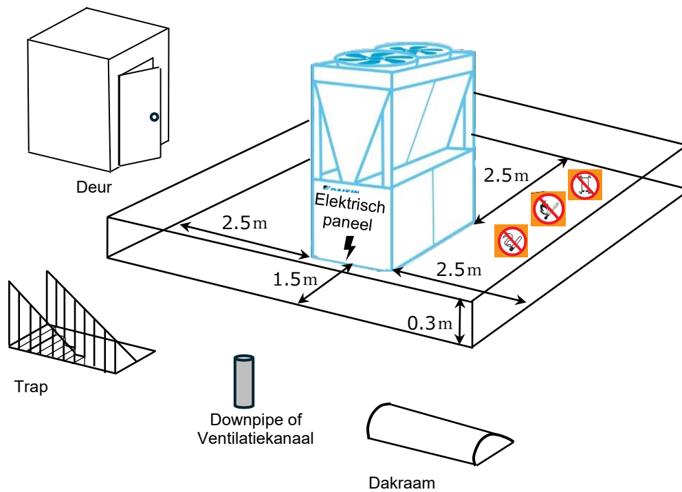
Afbeelding 14 – BRANDBARE ZONE voor enkele eenheid
