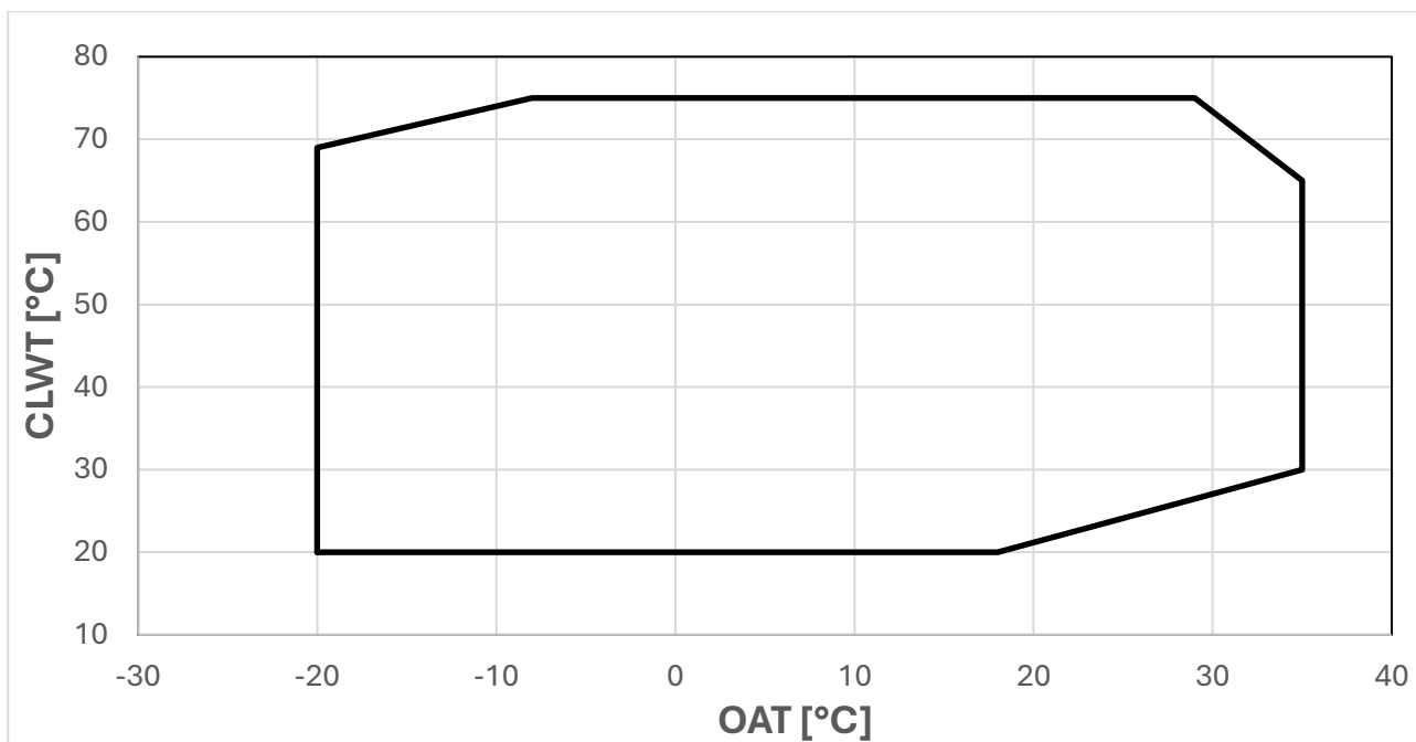
Afbeelding 36 - Bedieningslimieten verwarmingsmodus
