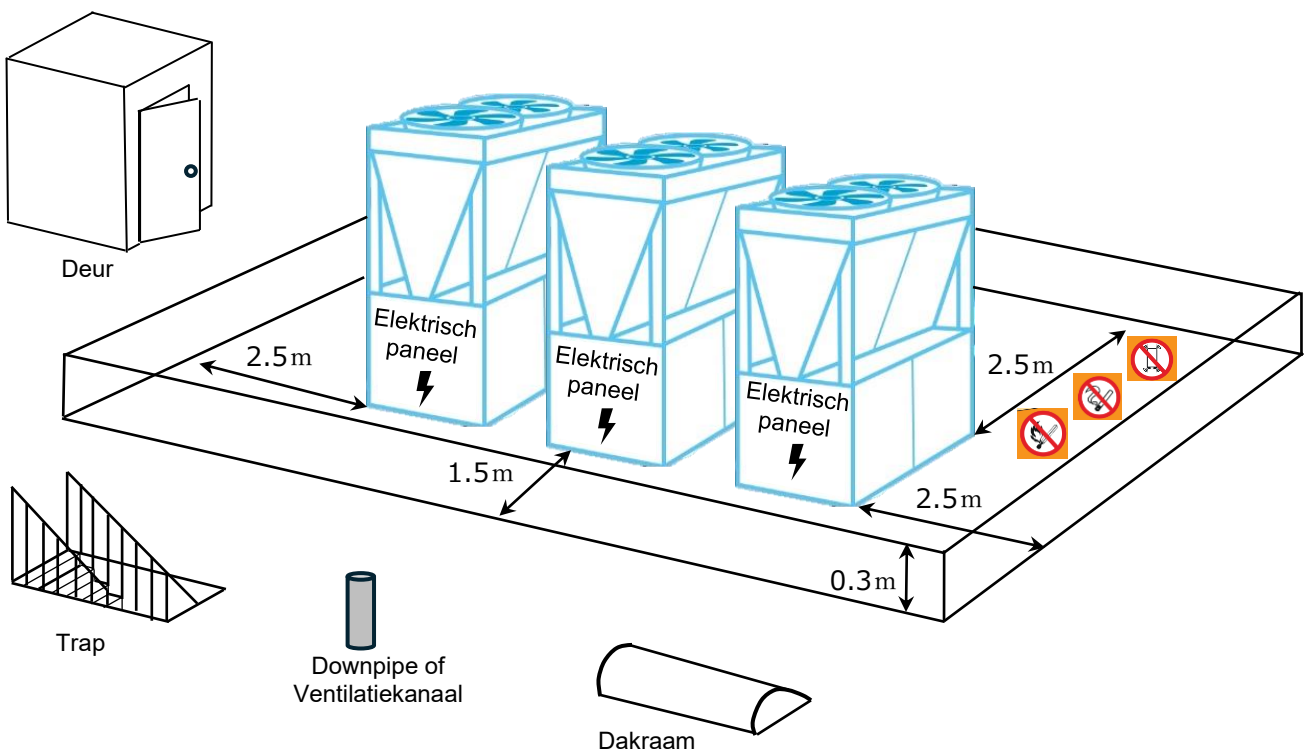
Afbeelding 15 – BRANDBARE ZONE voor modulaire eenheden
