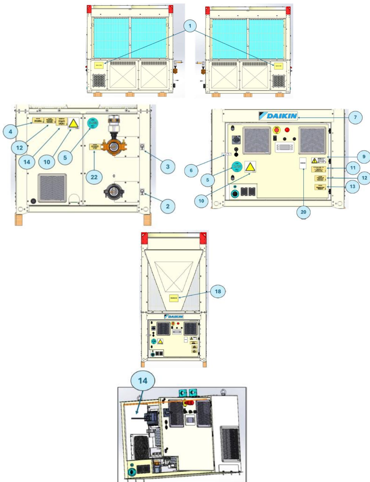
Afbeelding 37 - Labels op de eenheid
