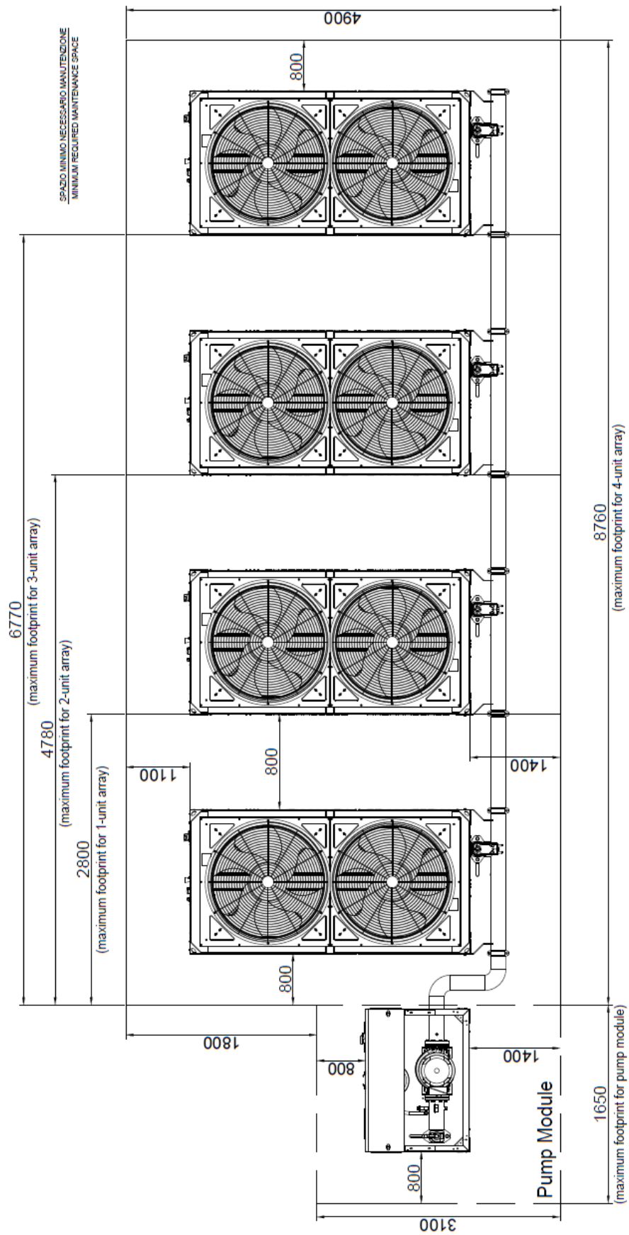
Afbeelding 6 – Maatschetsen – array installatie PAR3
