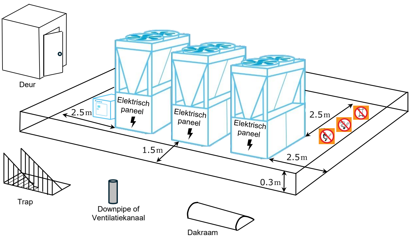
Afbeelding 17 – BRANDBARE ZONE voor modulaire eenheden met Daikin-pompmodule
