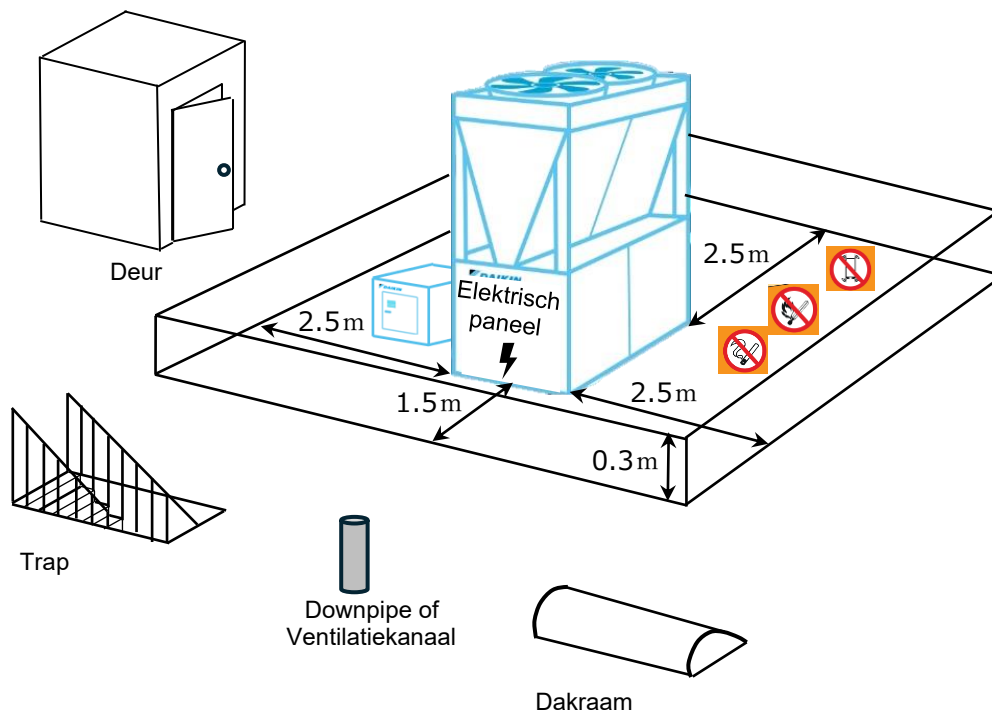
Afbeelding 16 – BRANDBARE ZONE voor enkele eenheid met Daikin-pompmodule
