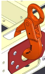
Obrázek 23 – Připojení bezpečnostního háku
