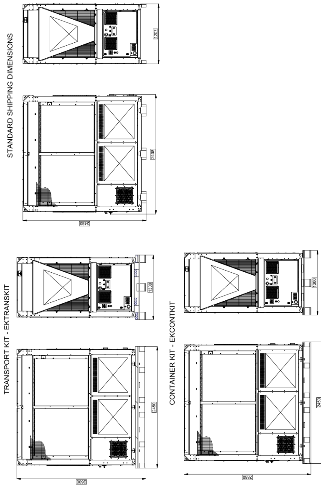
Obrázek 5 – Převážní sada, Kontejnerová sada a Převážní rozměry rozměrový výkres
