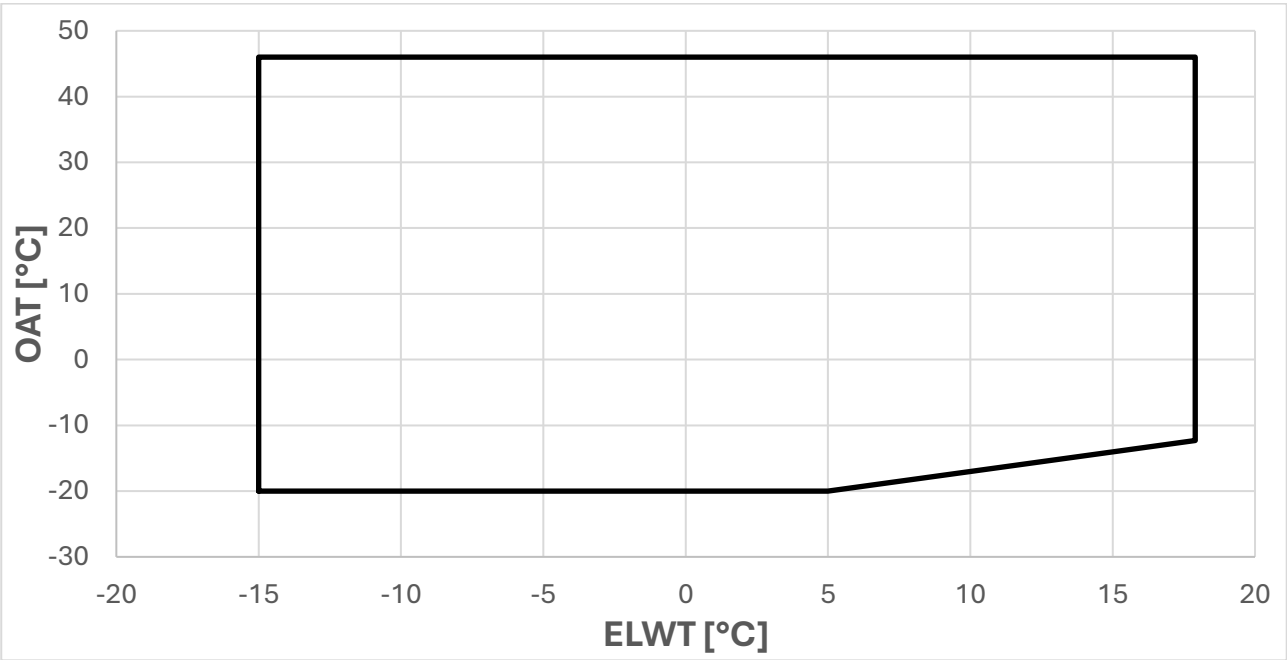
Figura 35 - Límites de Funcionamiento del Modo de Enfriamiento-EWYK100
