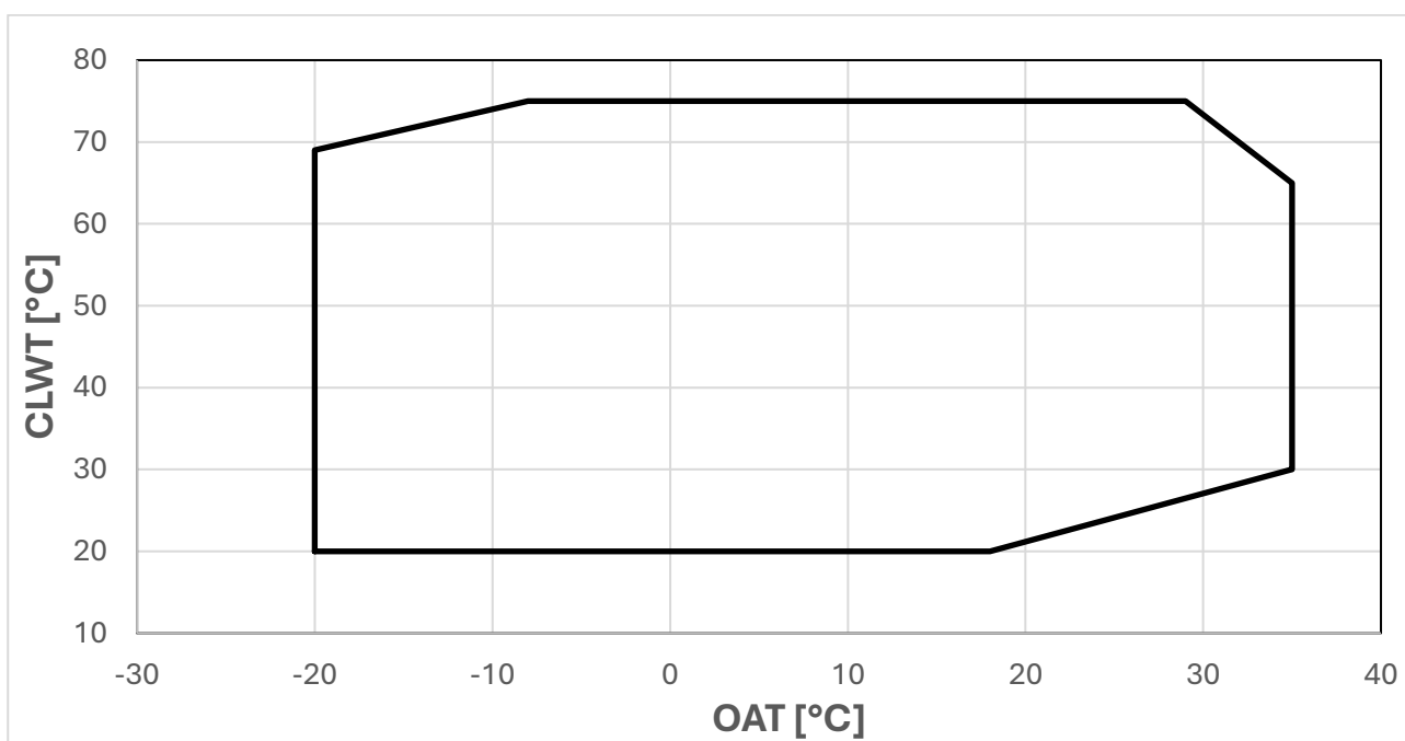
Figura 38 - Límites de Funcionamiento del Modo de Calentamiento-EWYK135
