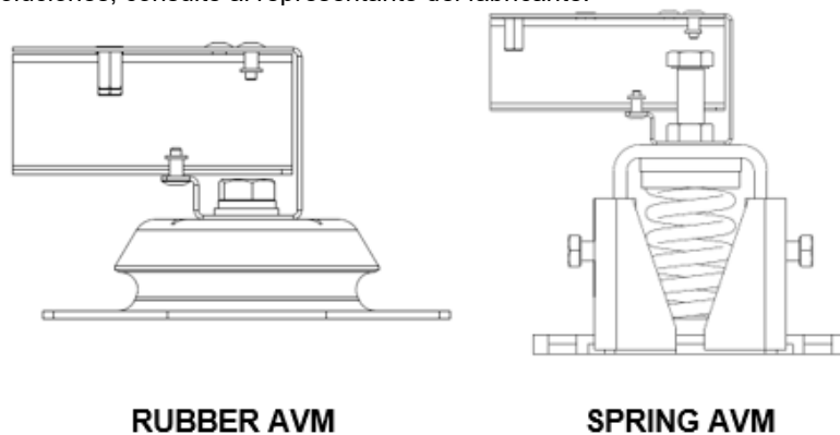
Figura 26 – Aisladores
