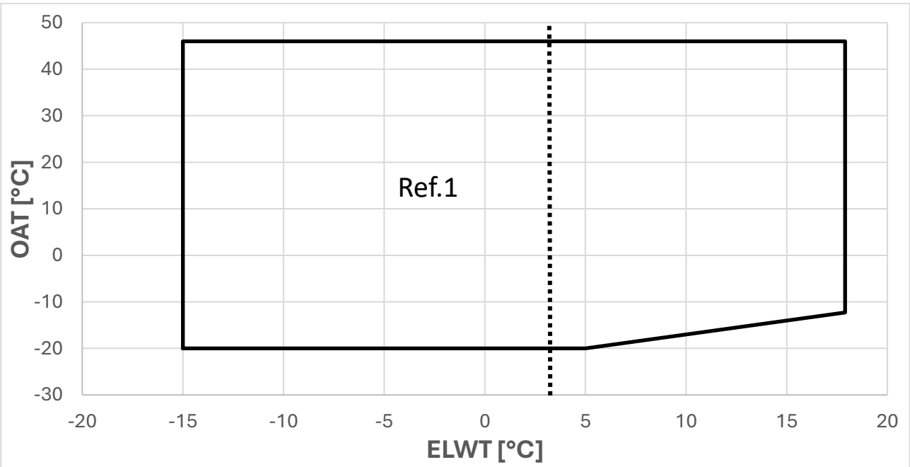
Figura 36 - Límites de Funcionamiento del Modo de Enfriamiento EWYK135
