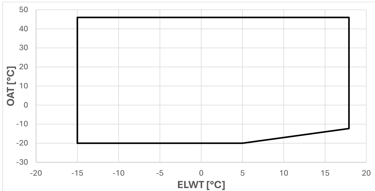
Afbeelding 35 - Bedieningslimieten koelmodus-EWYK100
