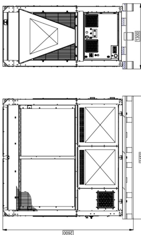
Afbeelding 5 – Transportkit, Containerset en Verzendafmetingen maatschets
