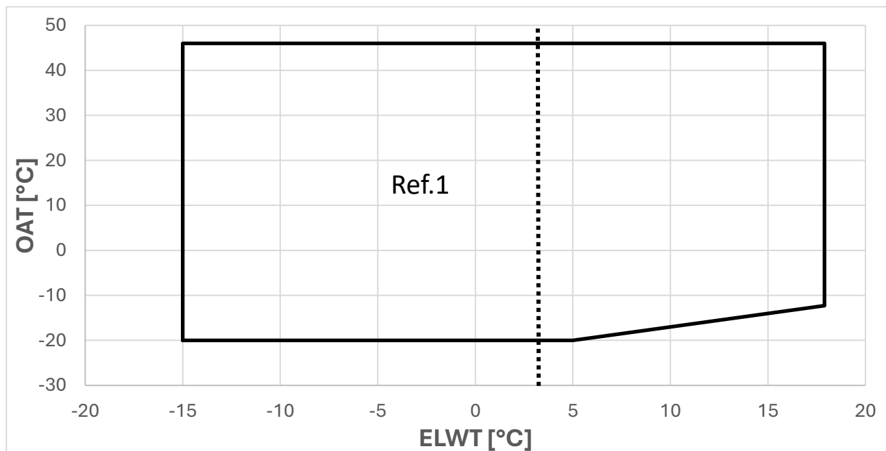
Afbeelding 36 - Bedieningslimieten koelmodus-EWYK135
