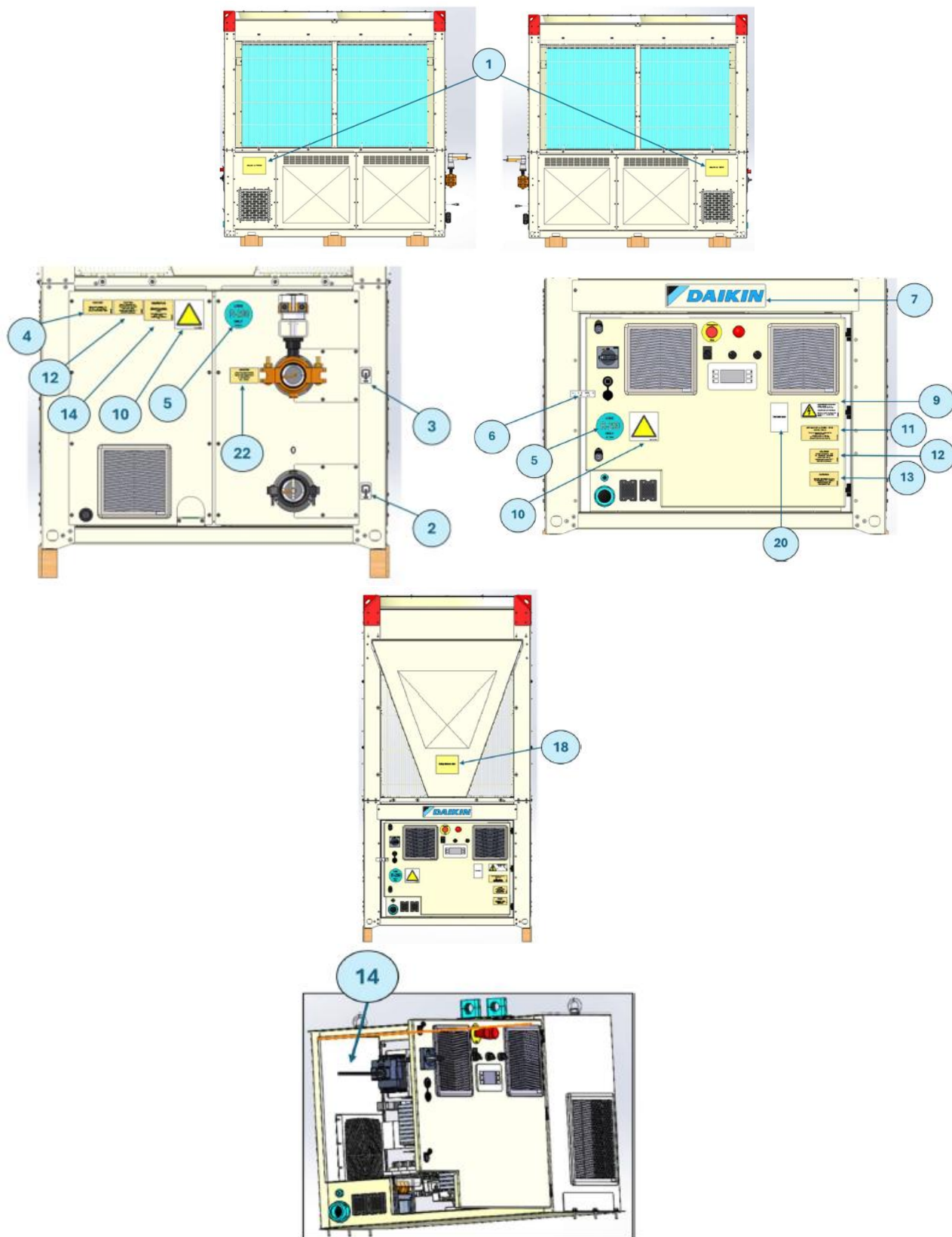
Afbeelding 39 - Labels op de eenheid
